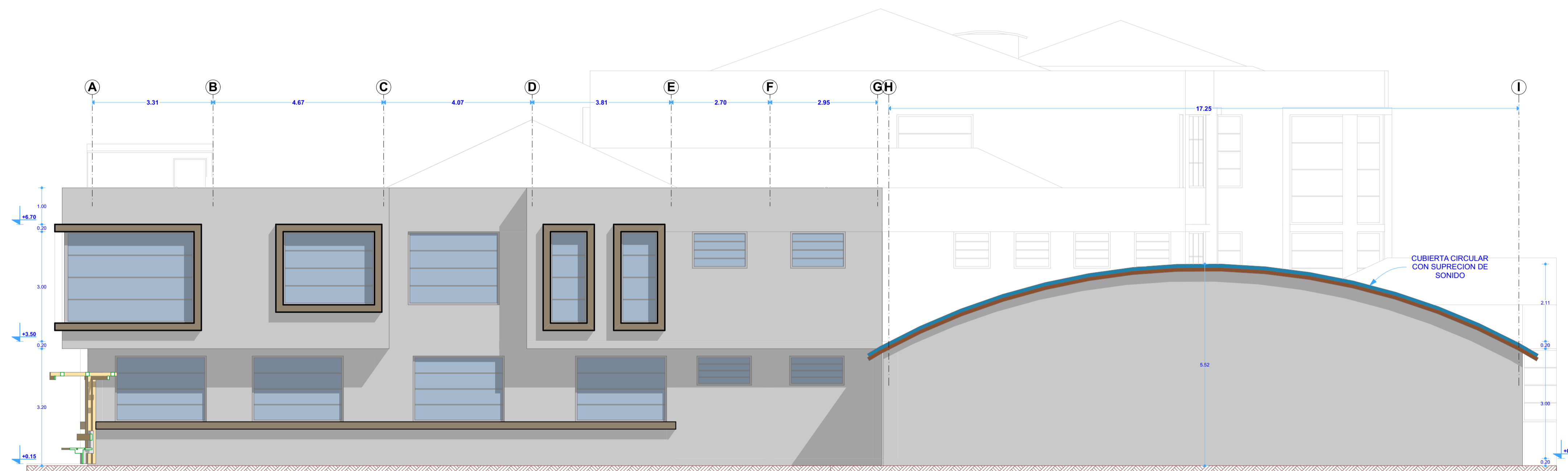
E5 ELEVACION Esc: 1:75 ZONA DE TRATAMIENTO
