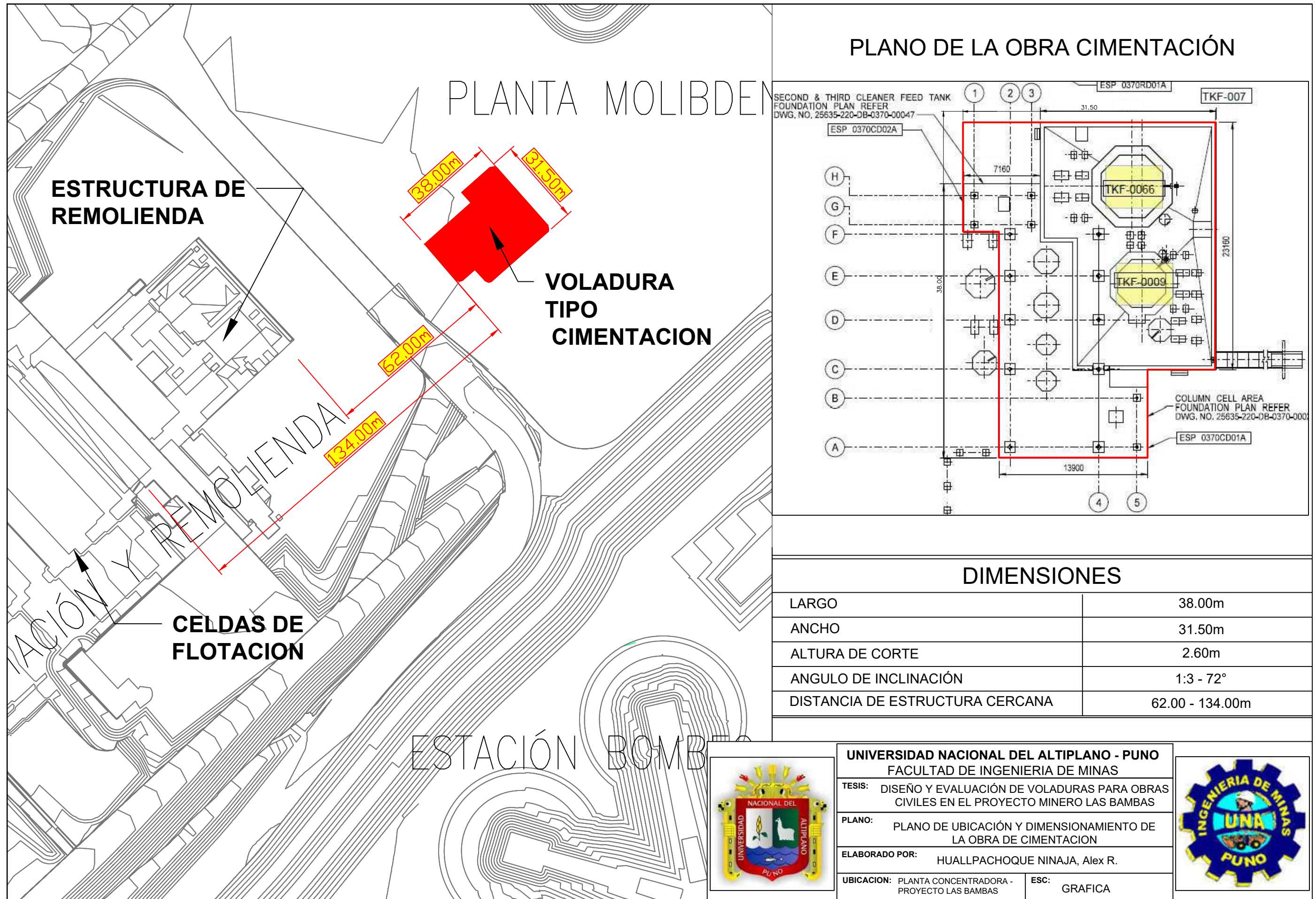
Figura N° 28: Plano de ubicación y dimensionamiento de la cimentación
