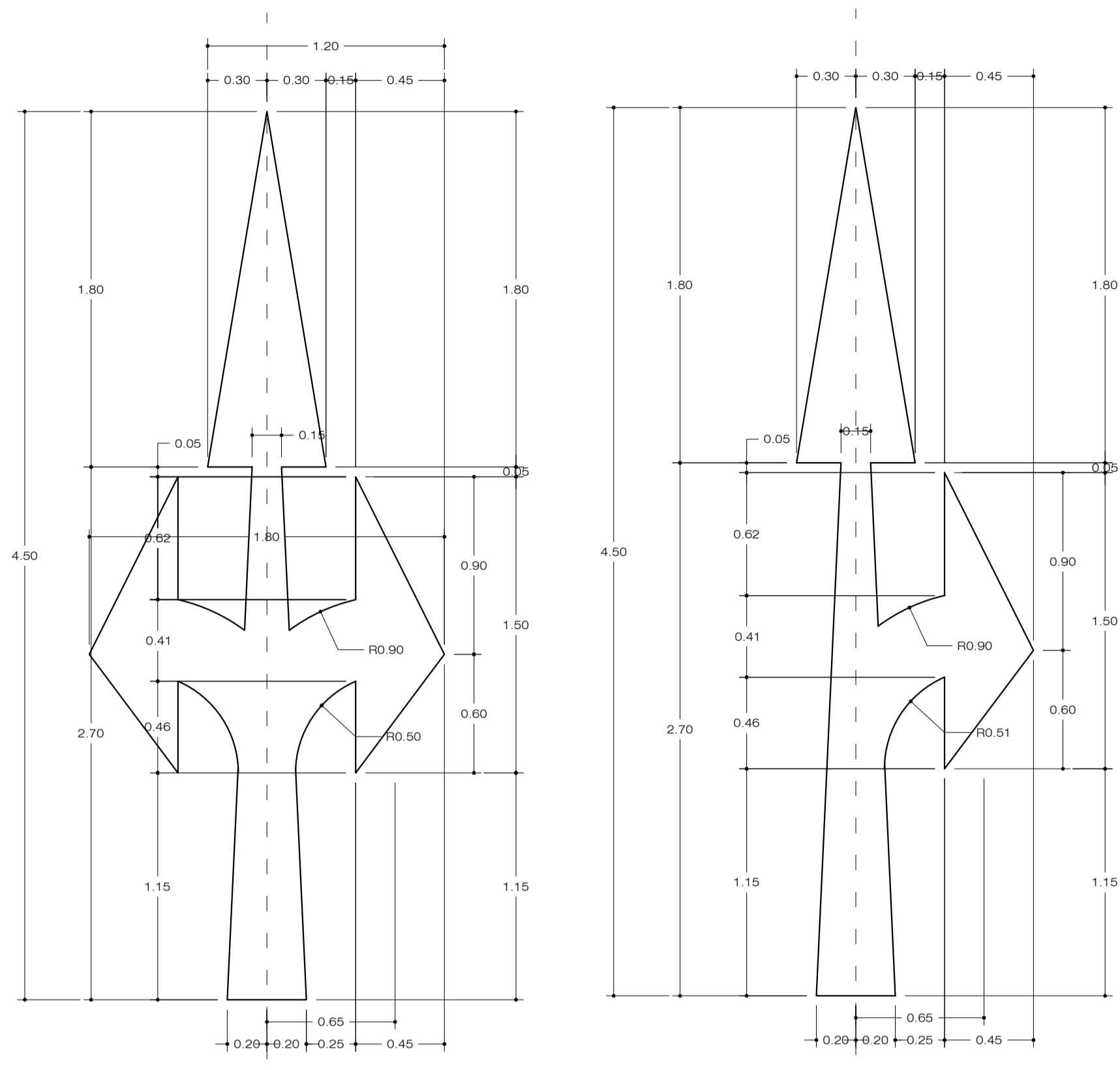
FLECHA DIRECCIONAL TIPO 1 ÁREA DE PINTURA: 2.30 M2. FLECHA DIRECCIONAL TIPO 2 ÁREA DE PINTURA: 1.80 M2.
