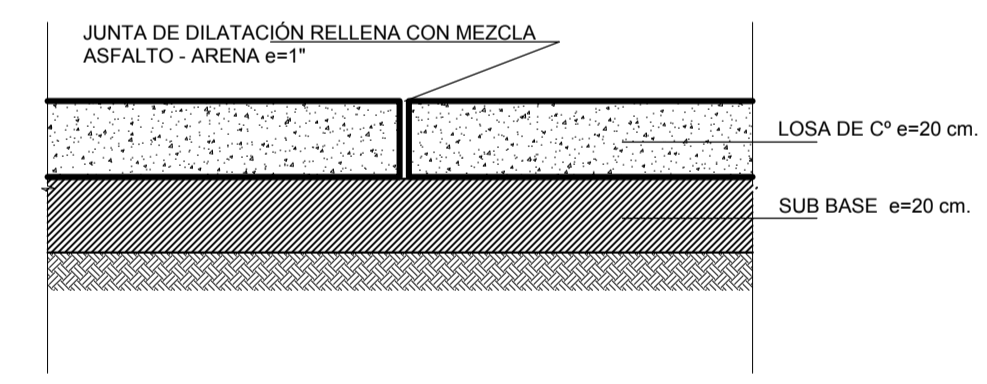
SECCIÓN 1-1 ESC: 1 / 20
