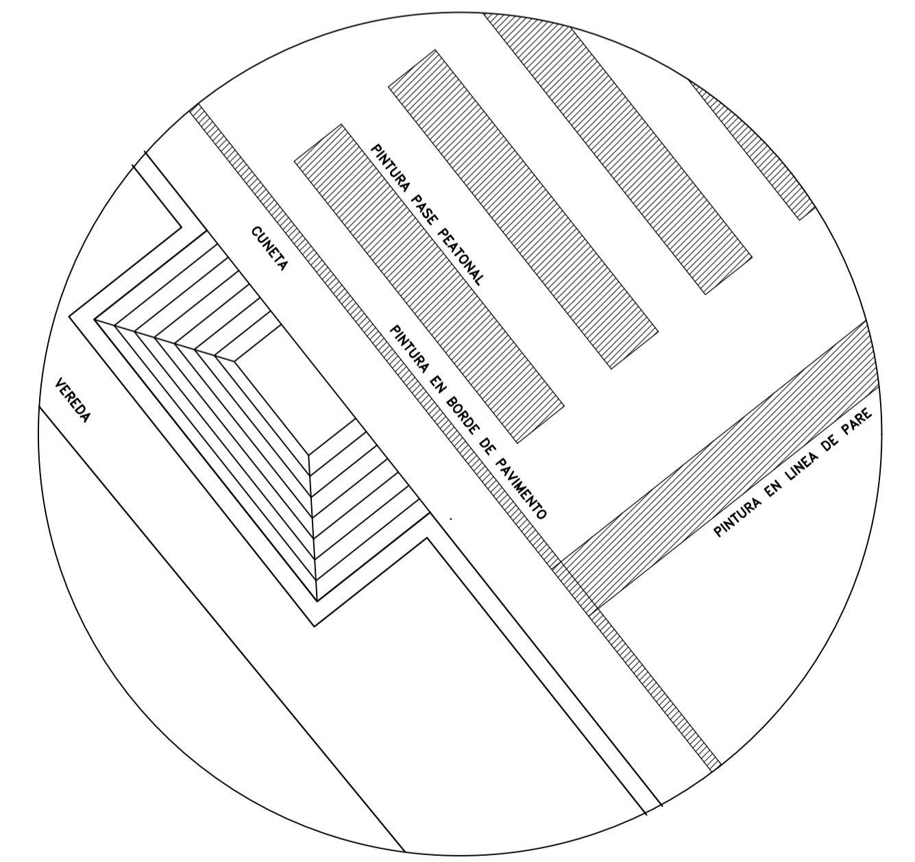
ENCUENTRO CRUCE Y RAMPAS PEATONALES
