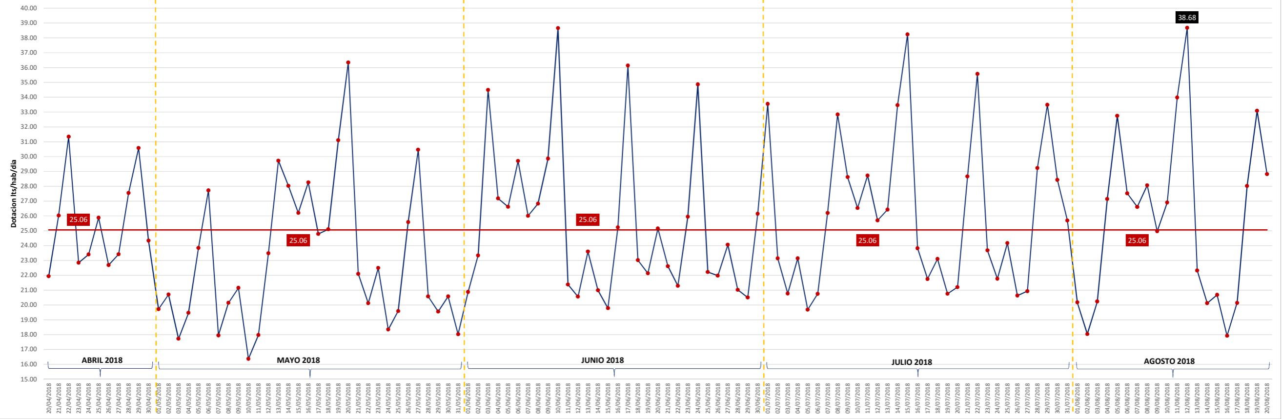
CURVA DE VARIACION DE CONSUMOS DIARIOS POR HABITANTE(Its/hab/dia)
