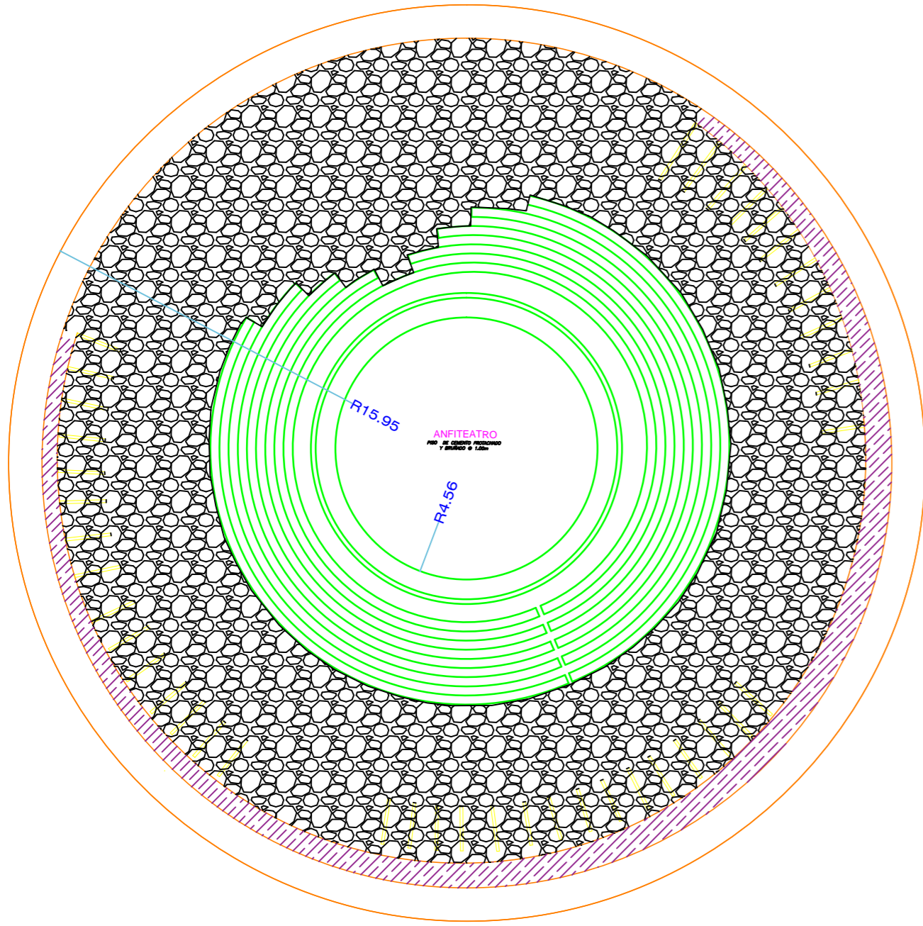
PLANTA DEL ANFITEATRO ESC. 1/125
