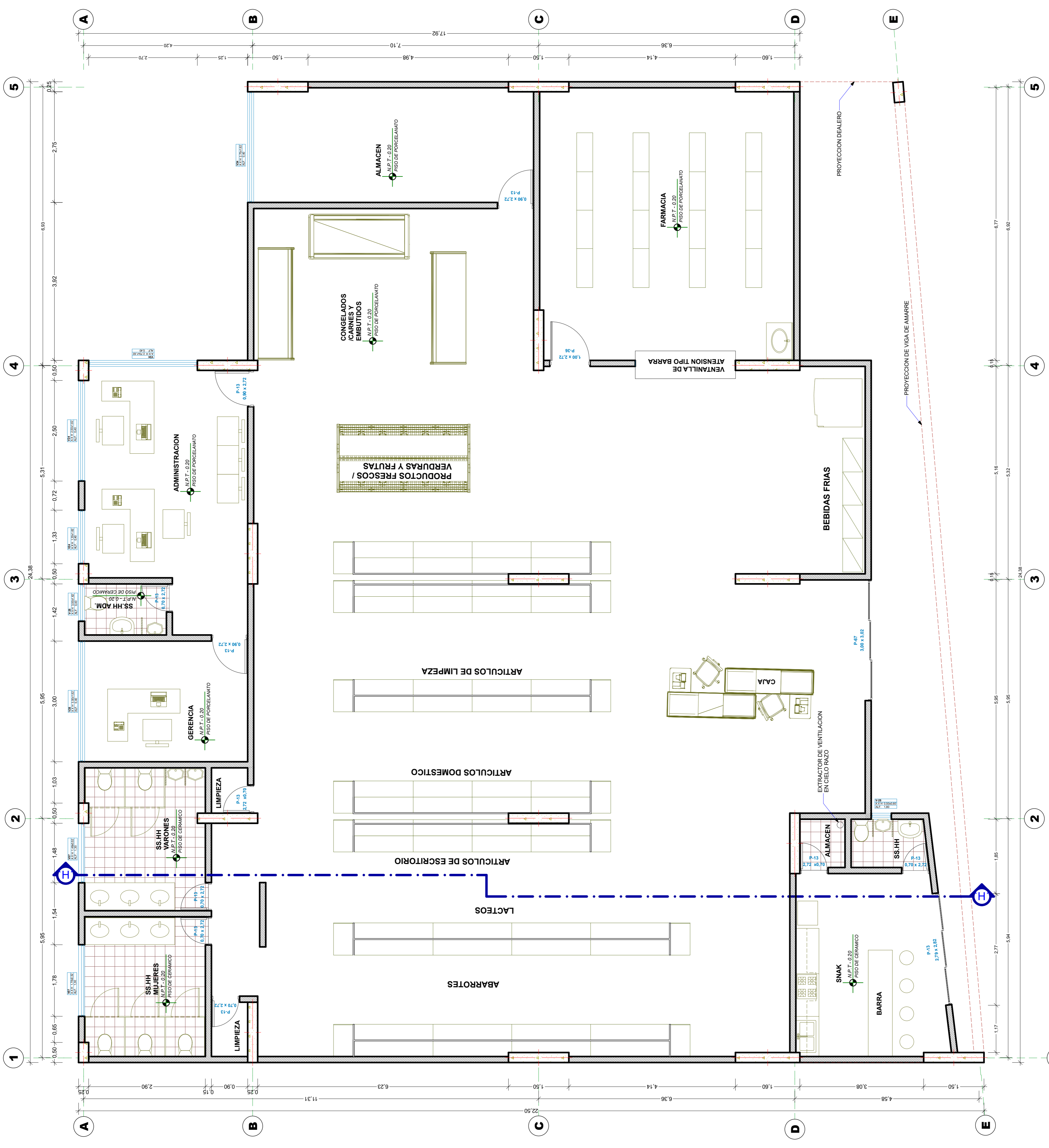
BLOQUE 05-PLANTA DE DISTRIBUCION- MINIMARQUET ESC. 1/50
