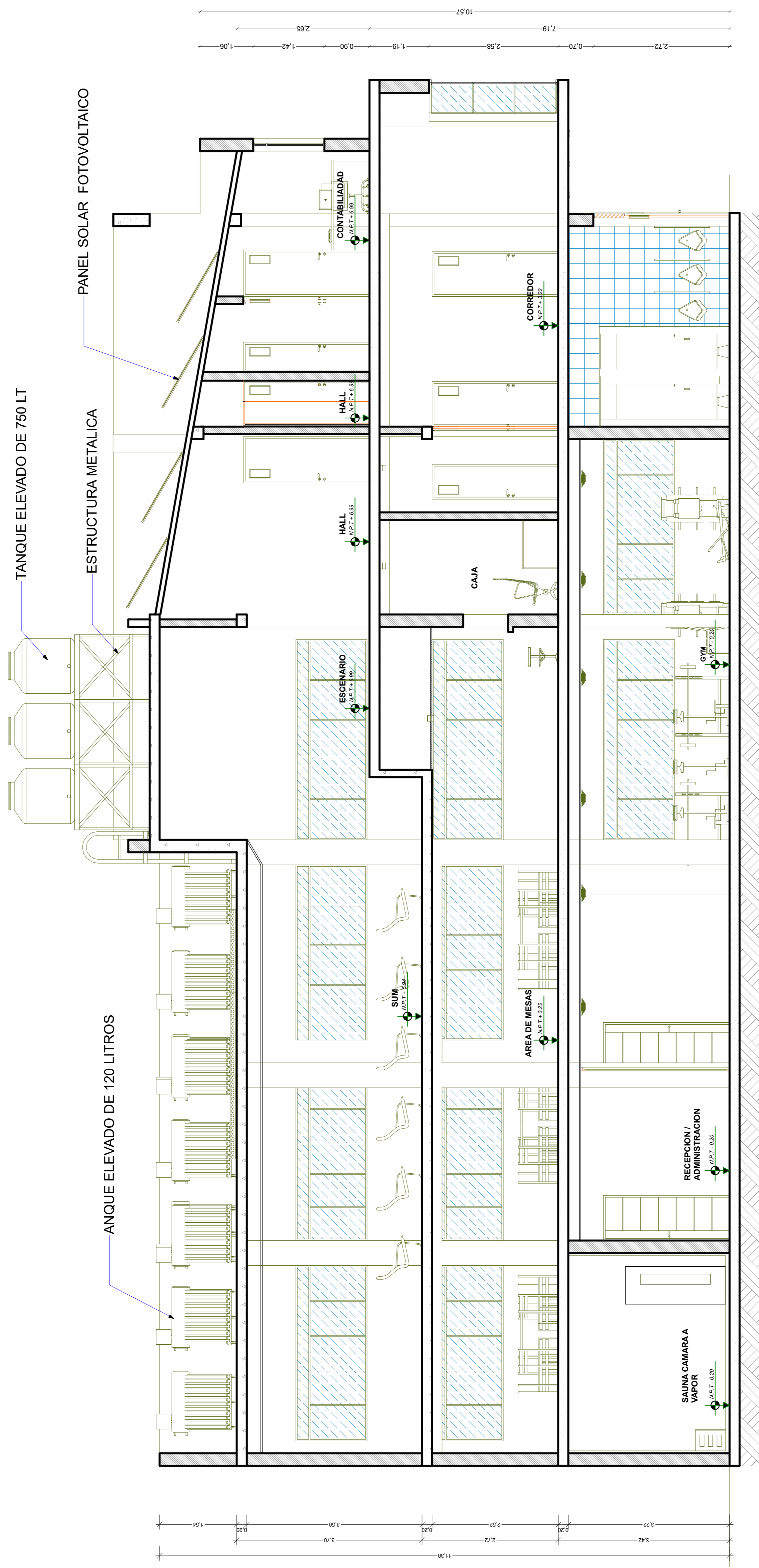
SECCION 'G'-G' / BLOQUE 04 ESC. 1/20
