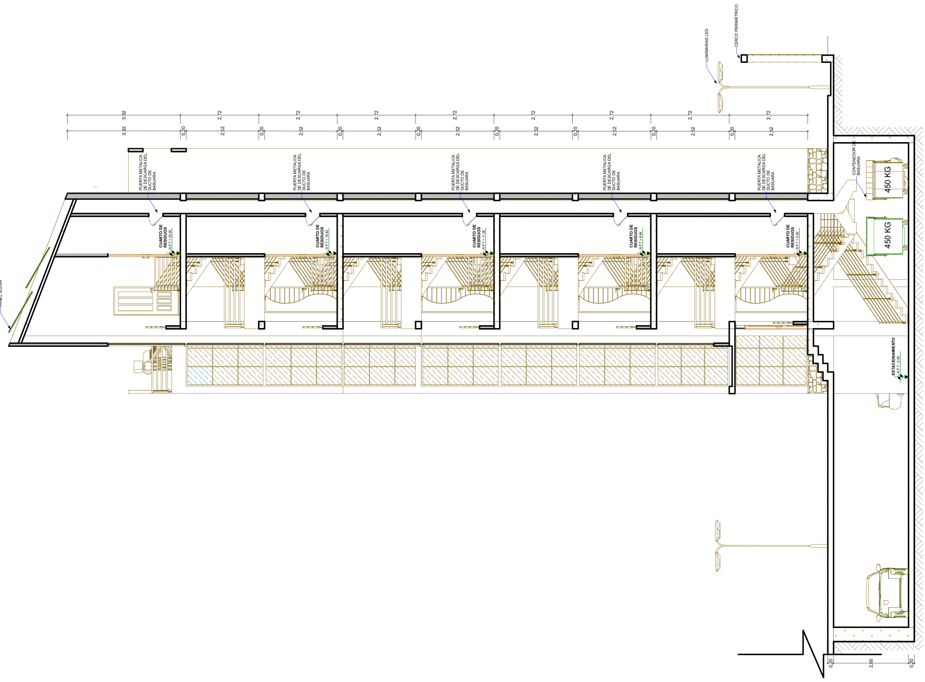
SECCION 'A-A' ESC. 1/75
