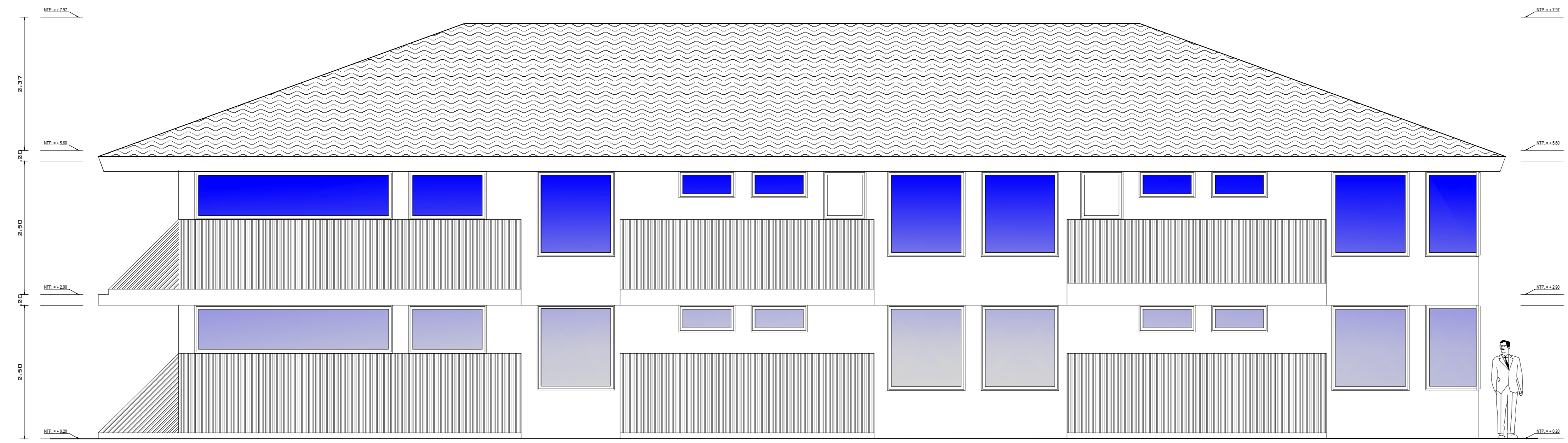
ELEVACION LATERAL Esc : 1 / 50
