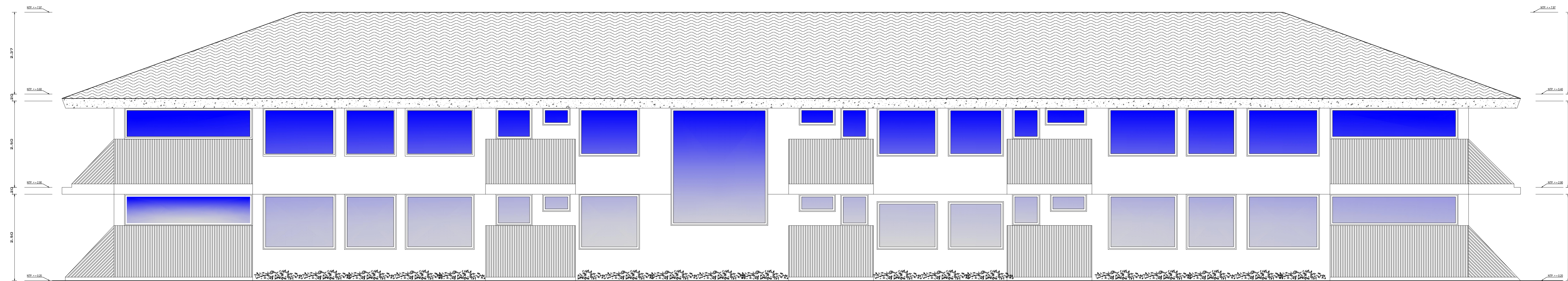
ELEVACION POSTERIOR Esc : 1 / 50
