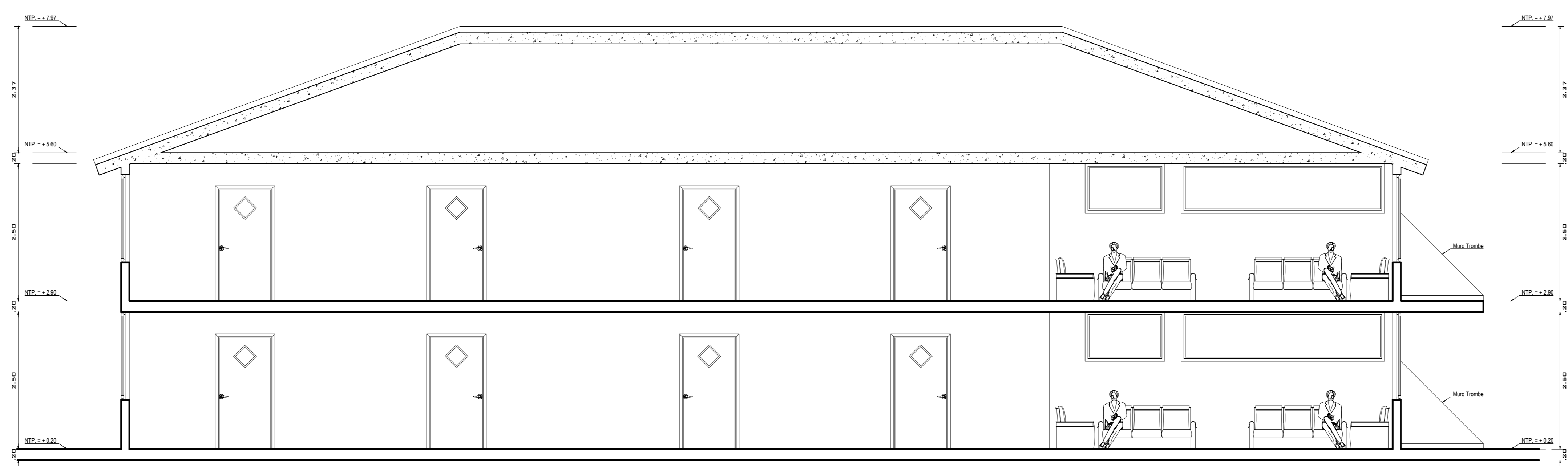
CORTE SECCION C - C Esc: 1 / 50
