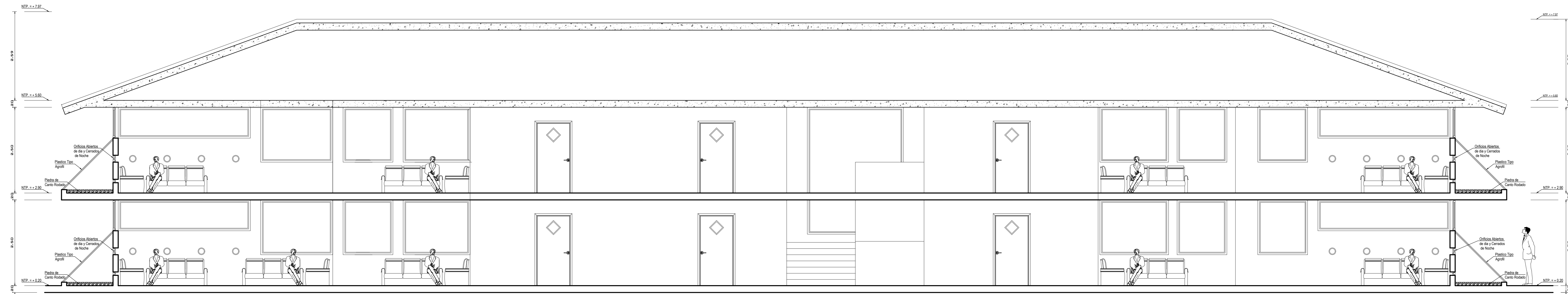
CORTE SECCION A - A Esc: 1 / 50
