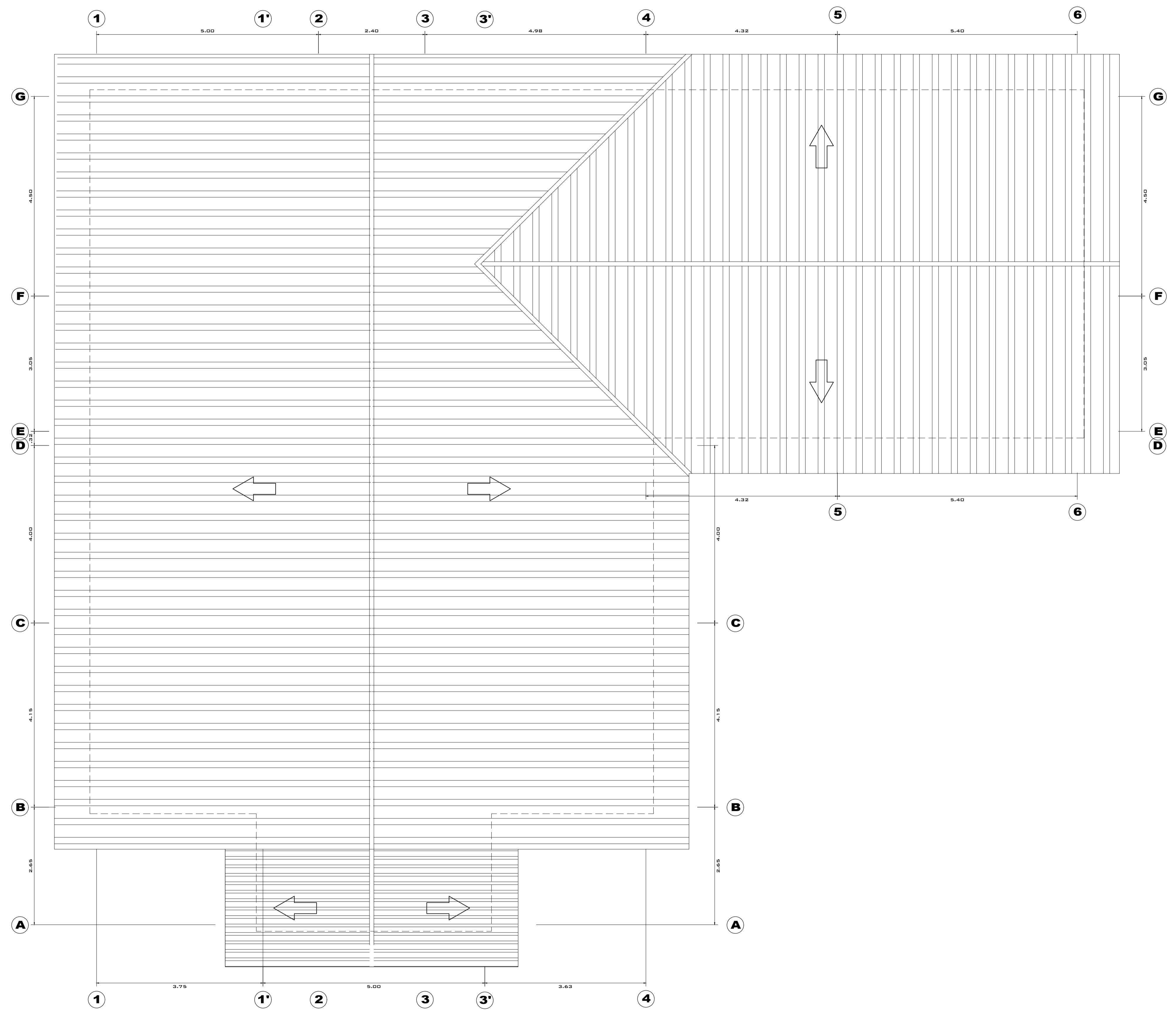
PLANO DE TECHOS Esc : 1 / 50
