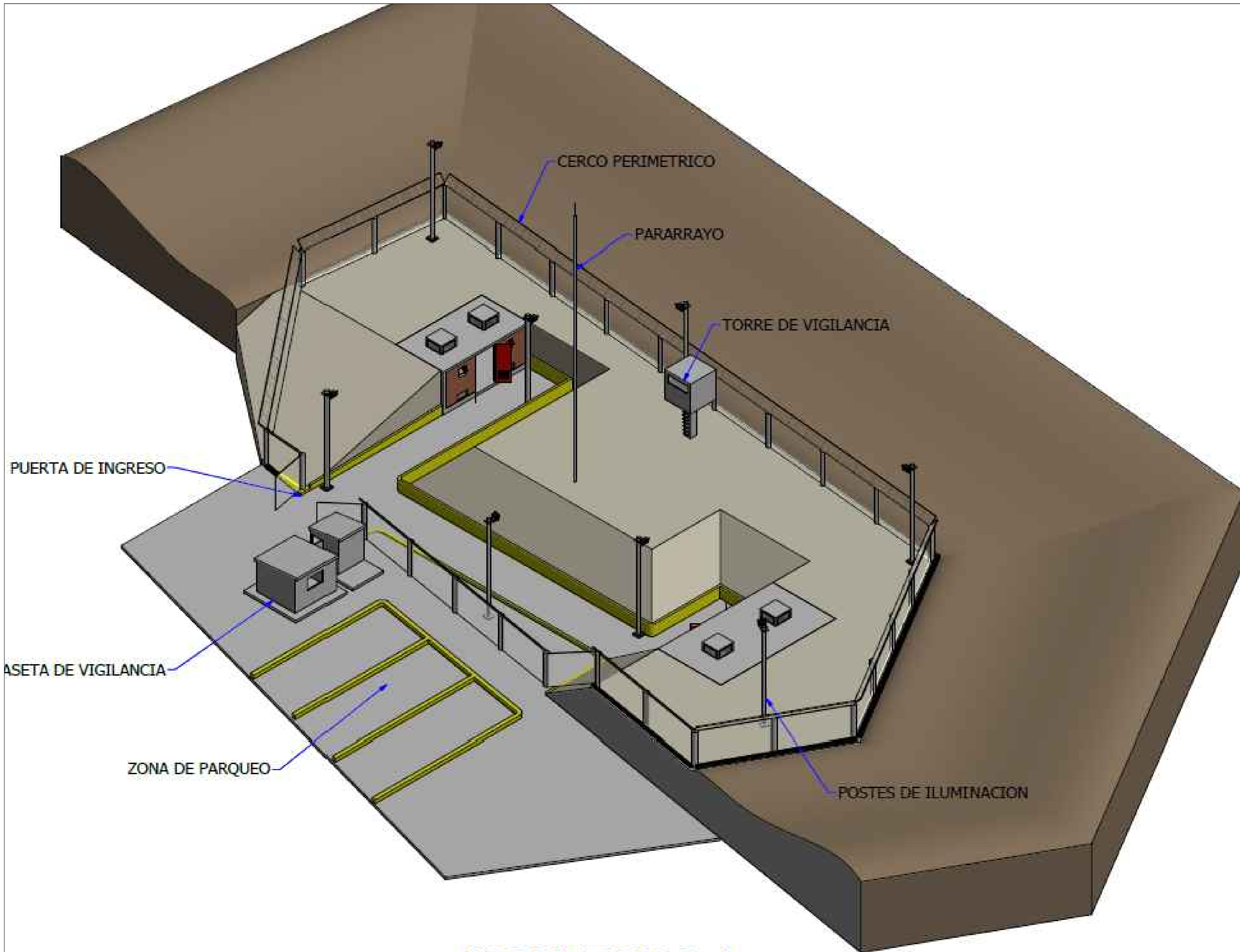
ISOMETRICO 1
