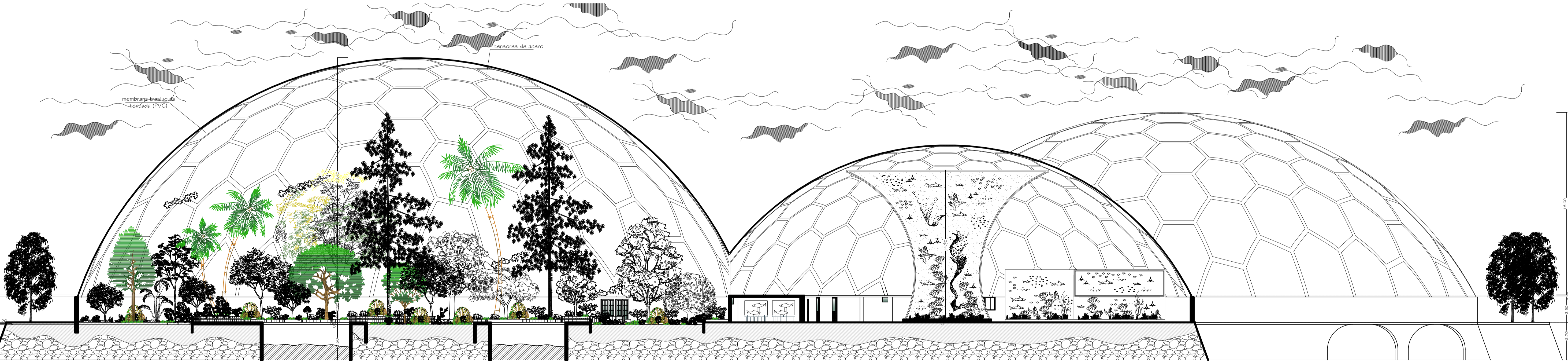
CORTE A - A Eso 1 / 200
