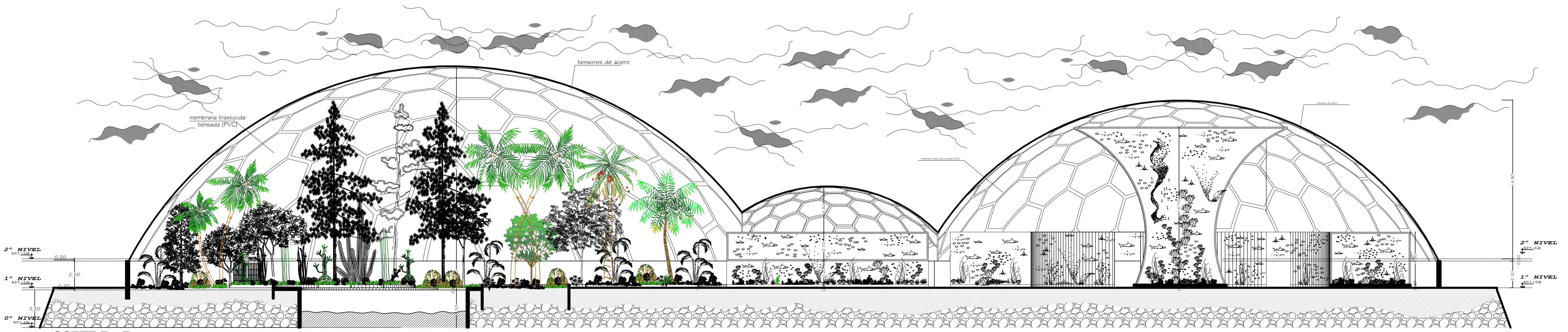
CORTE B - B Eso 1 / 200
