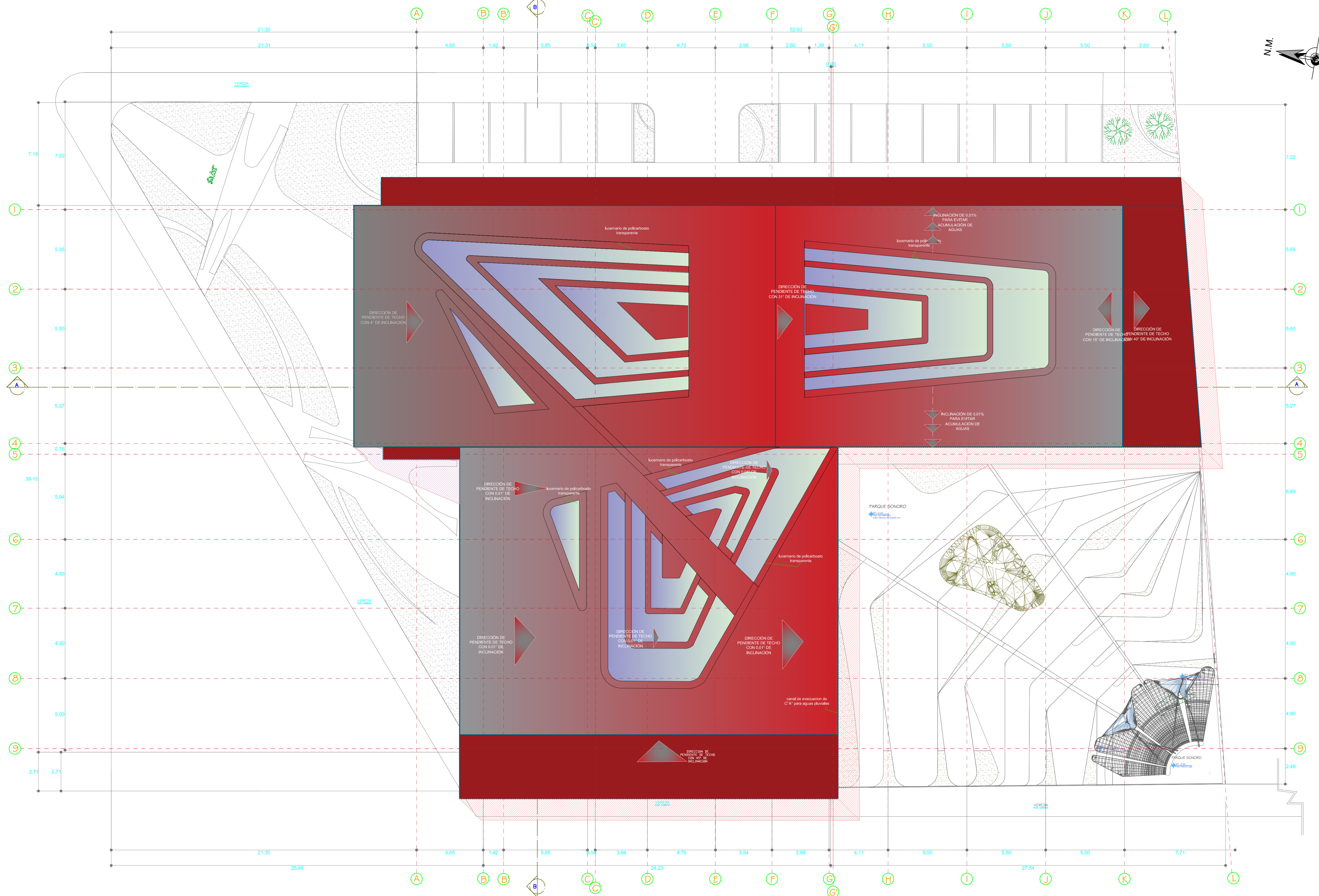
PLANO DE TECHOS - PLANO EN PLANTA Esc: 1 / 200
