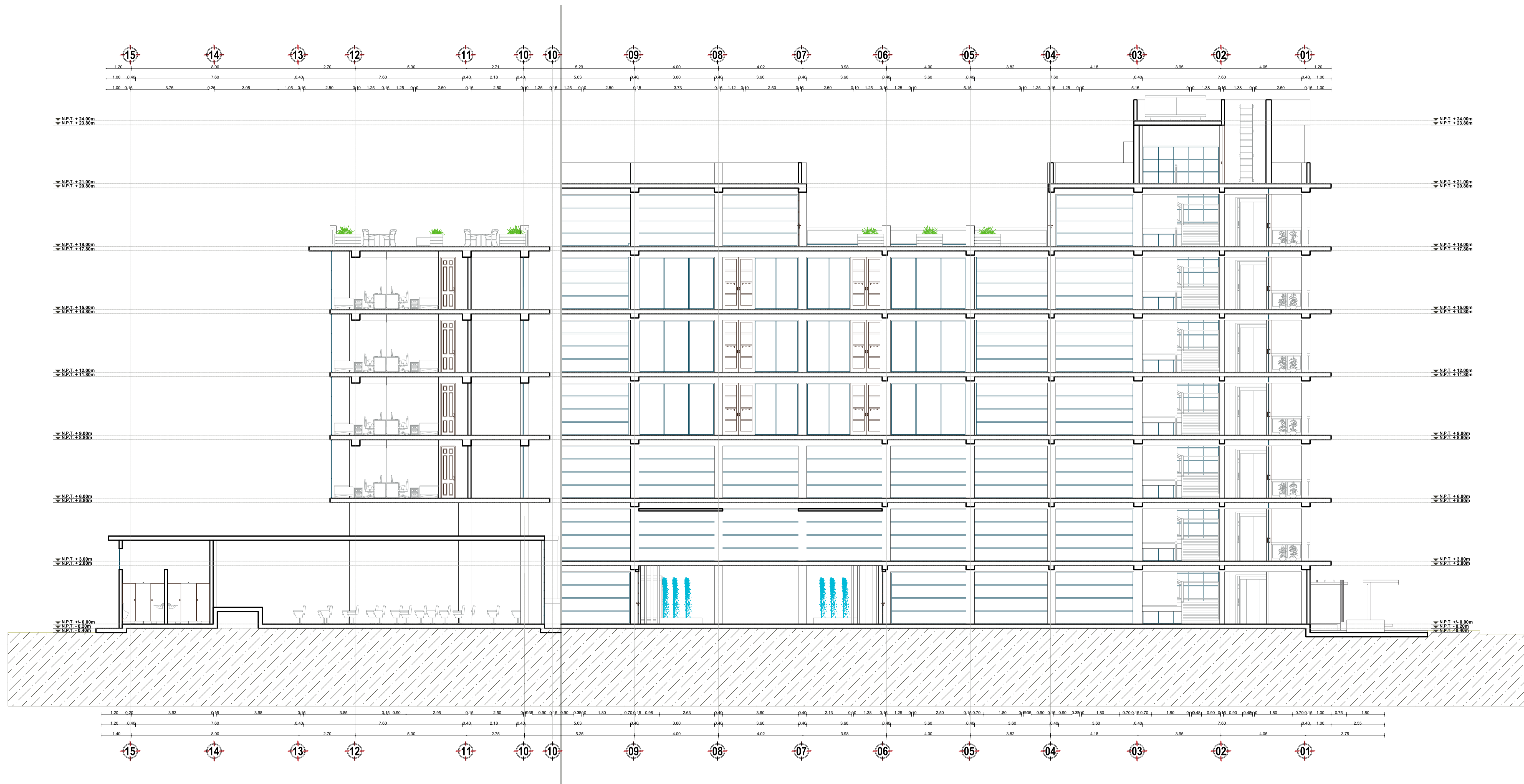
PLANO DE SECCION D-D VISTA DEL - BLOQUE DAMAS ESC: 1/100
