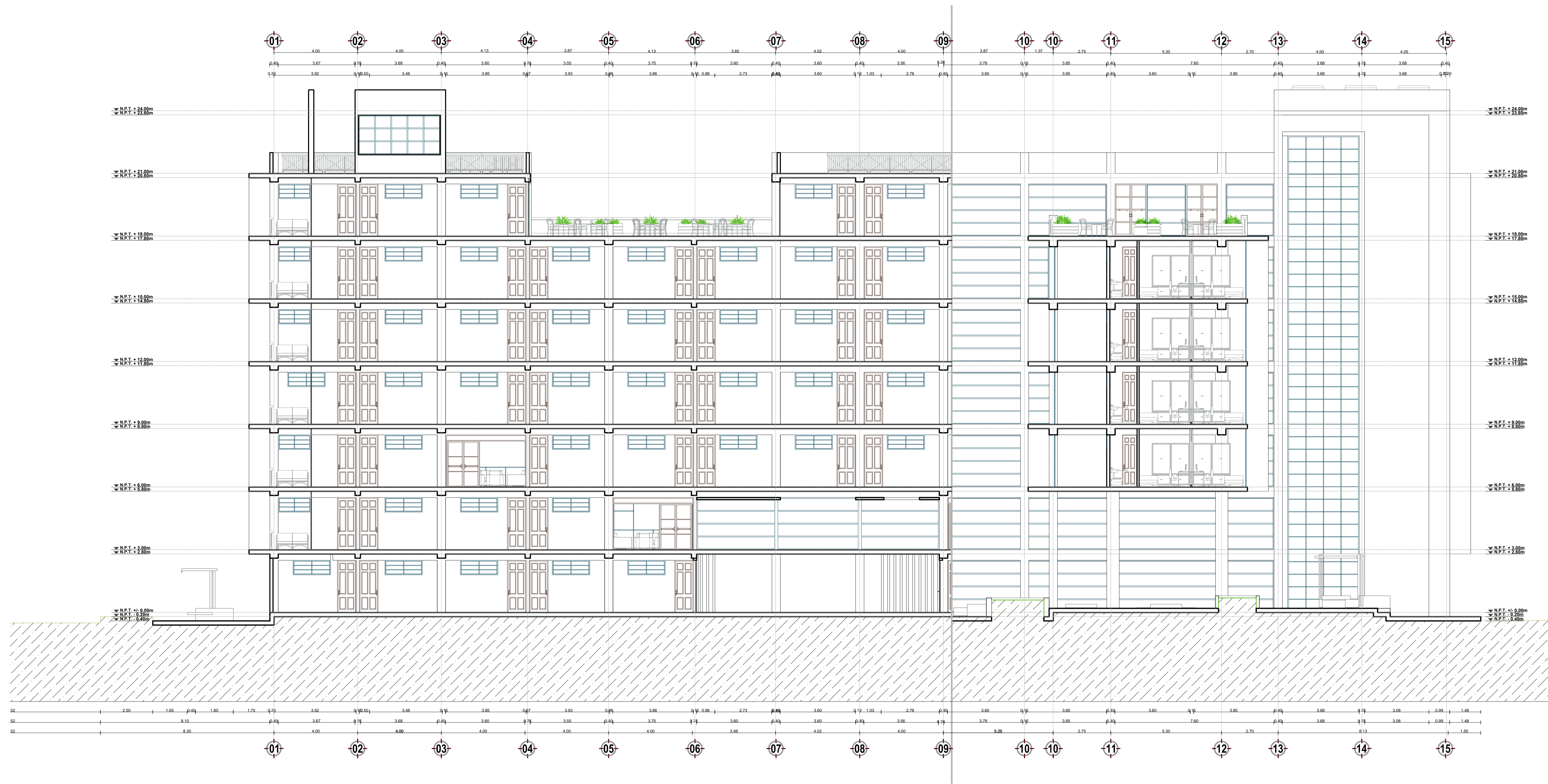
PLANO DE SECCION B-B VISTA DEL LADO OESTE - BLOQUE VARONES ESC: 1/100
