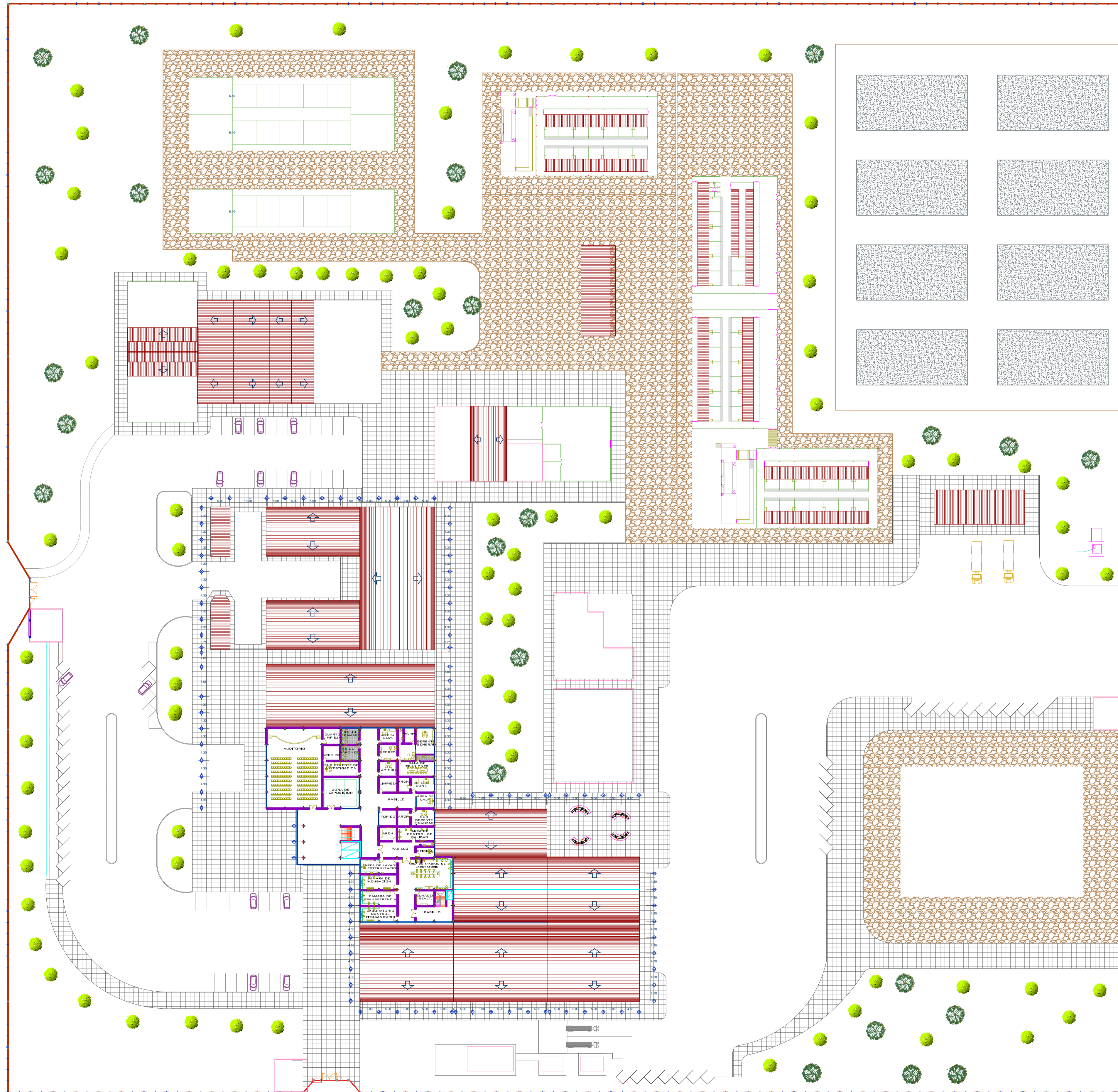
PLANIMETRIA GENERAL SEGUNDO NIVEL ESC: 1/500
