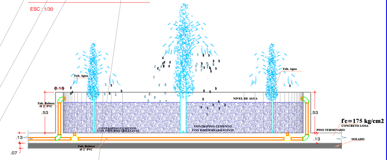
PILETA - REBOSE DE PILETA ESC: 1/30
