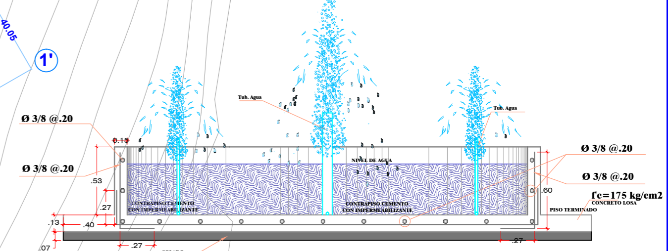
PILETA - SECCION A-A ESC: 1/30
