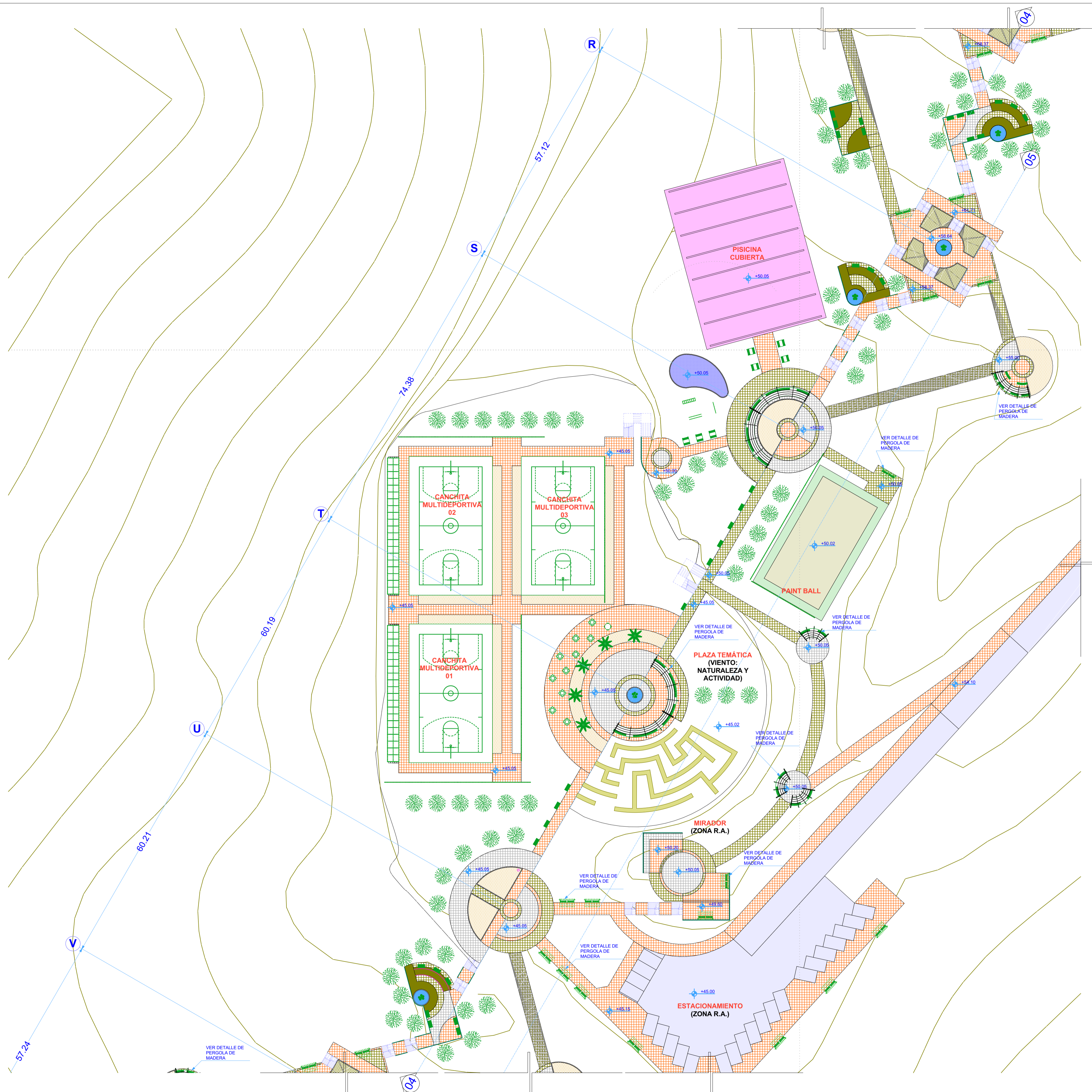
PLAZA ZONA RECREATIVA ACTIVA ESC: 1/500
