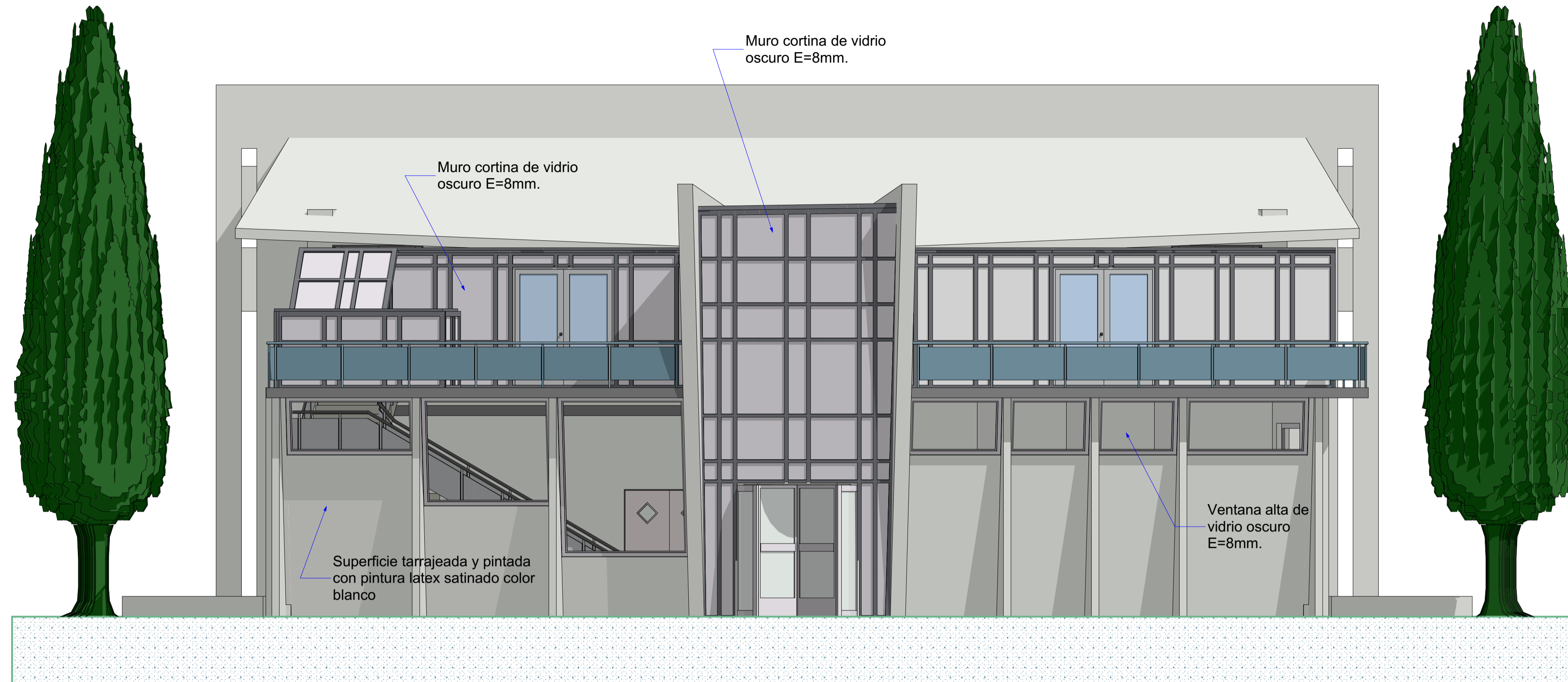
ELEVACION "A1" ESC:1/50
