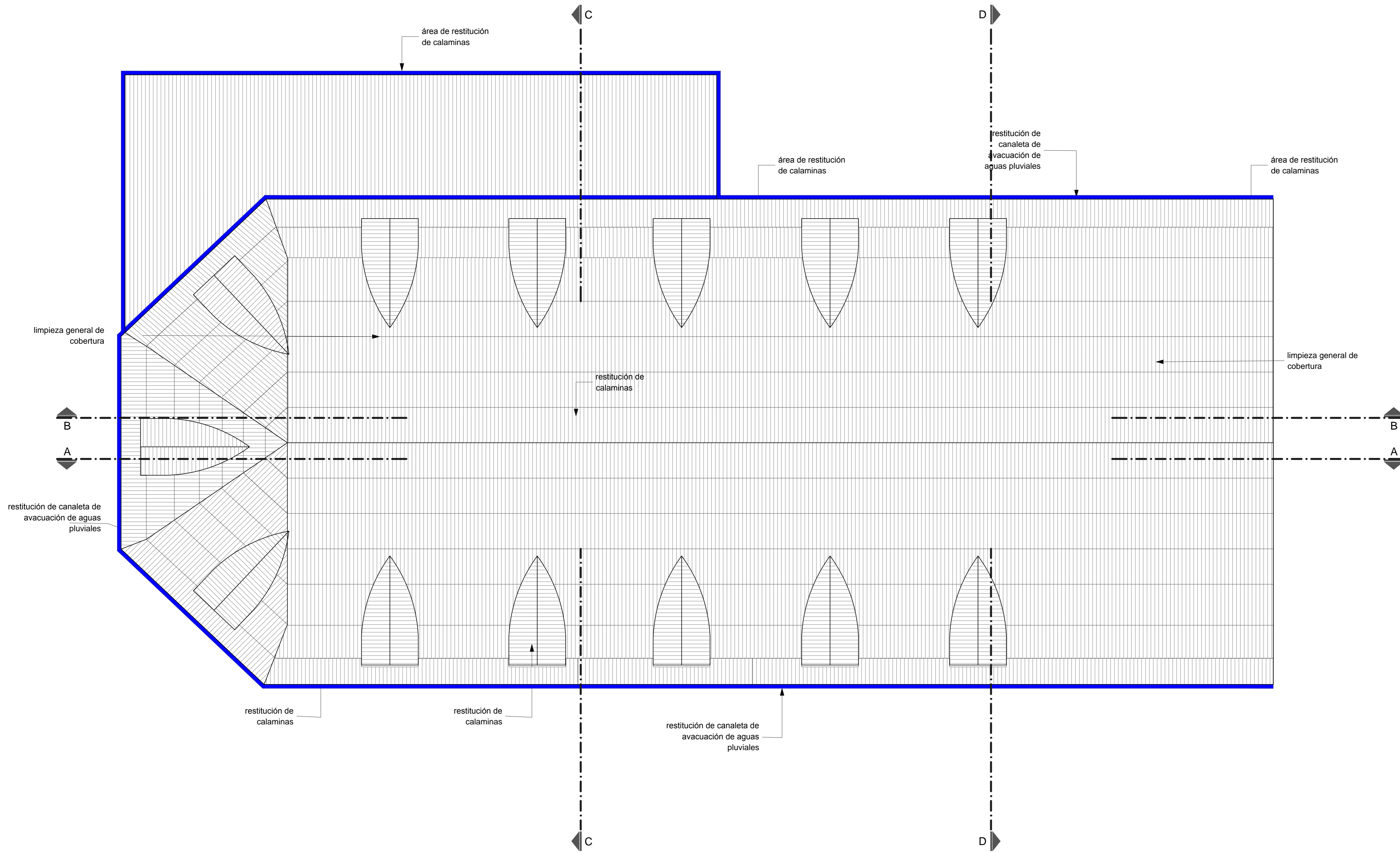
PLANO DE TECHO PROPUESTA DE RESTAURACION ESC 1/50
