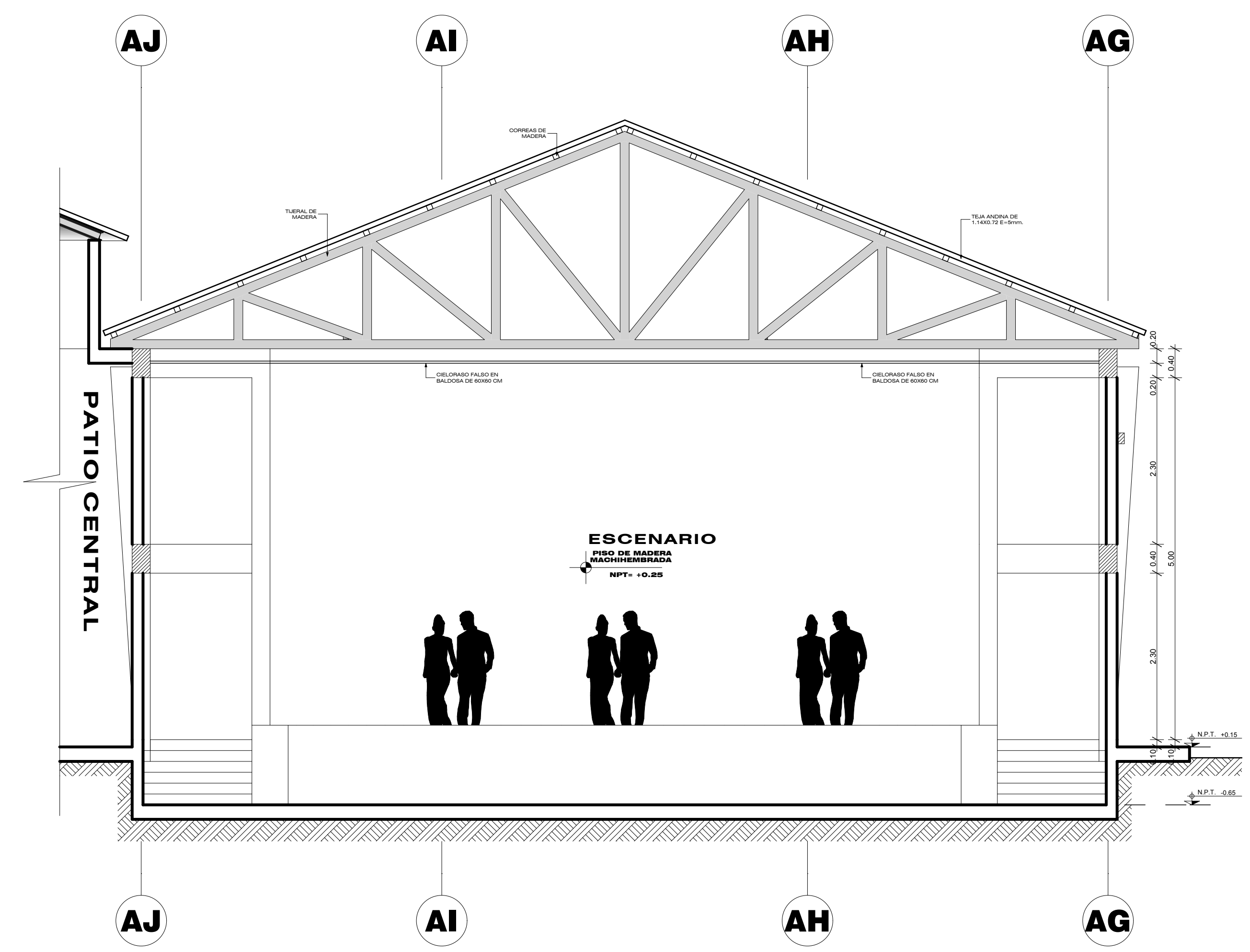
SECCION 0-0 DEL BLOQUE VIII ESCALA 1:50
