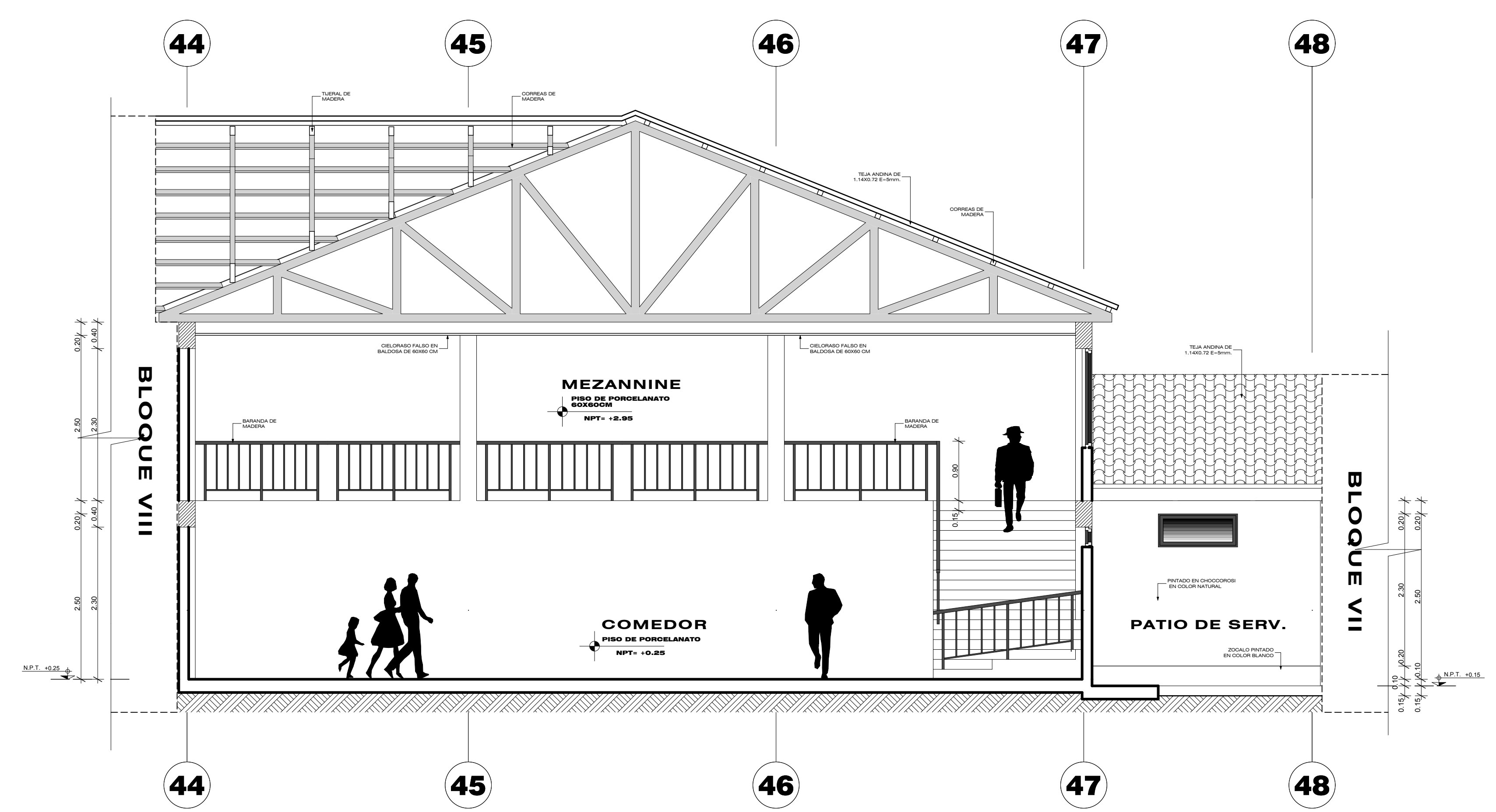
SECCION L-L DEL BLOQUE VI ESCALA 1:50
