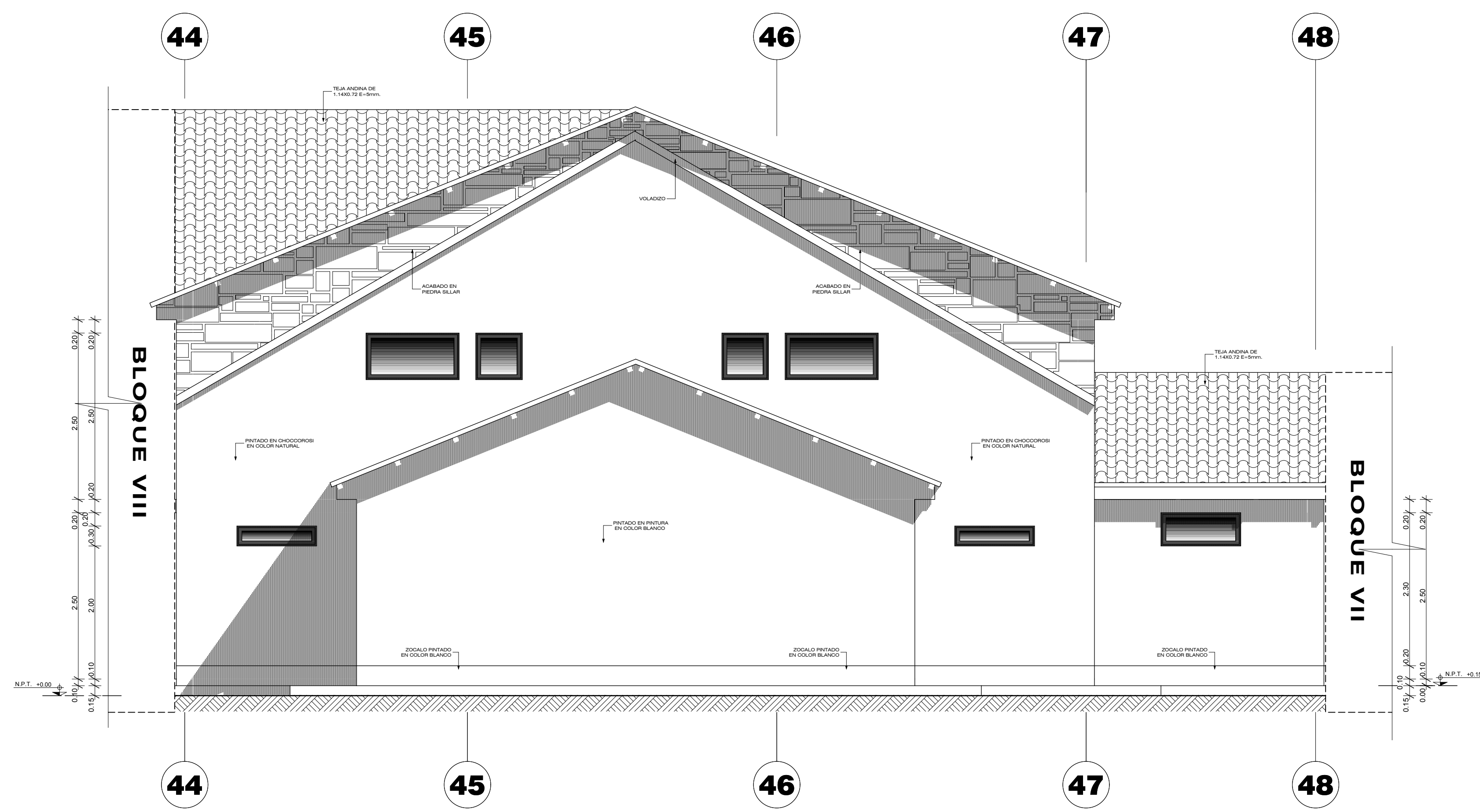
ELEVACION SUR DEL BLOQUE VI ESCALA 1:50
