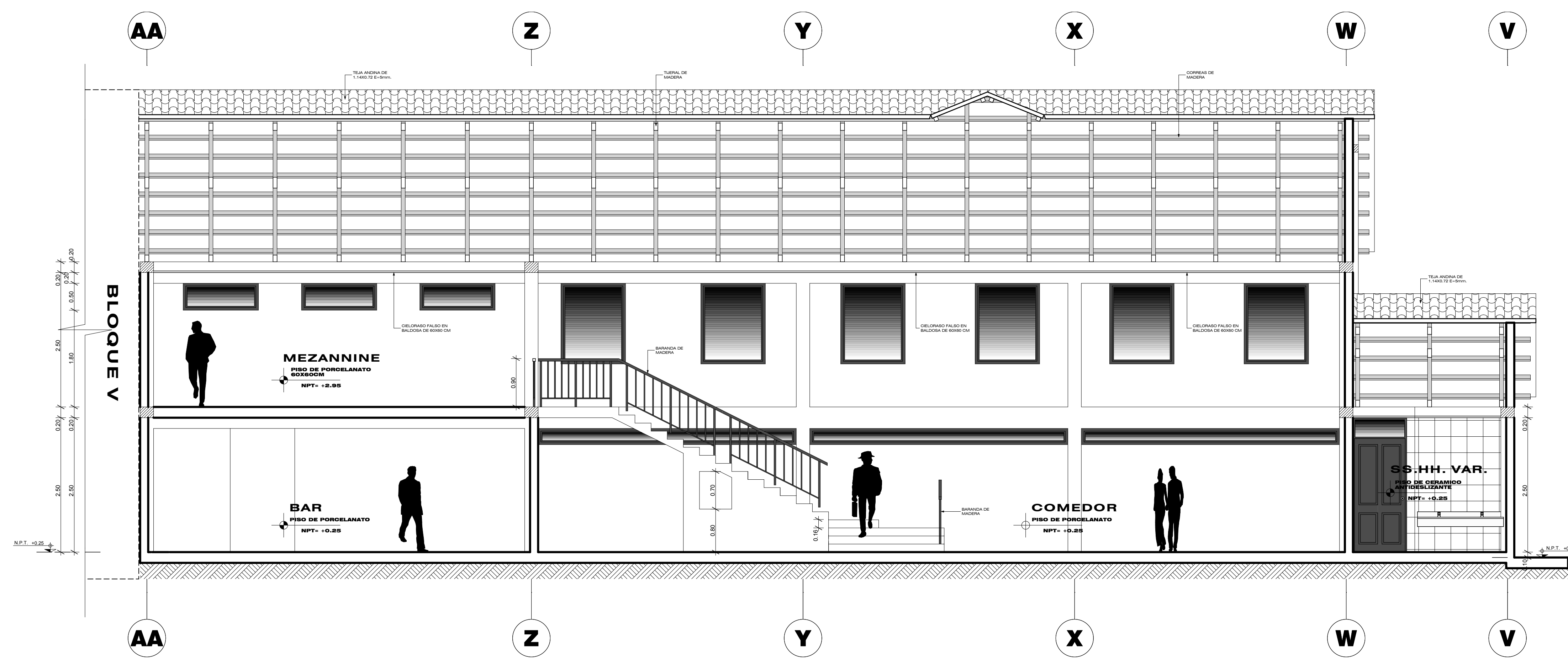
SECCION K-K DEL BLOQUE VI ESCALA 1:50
