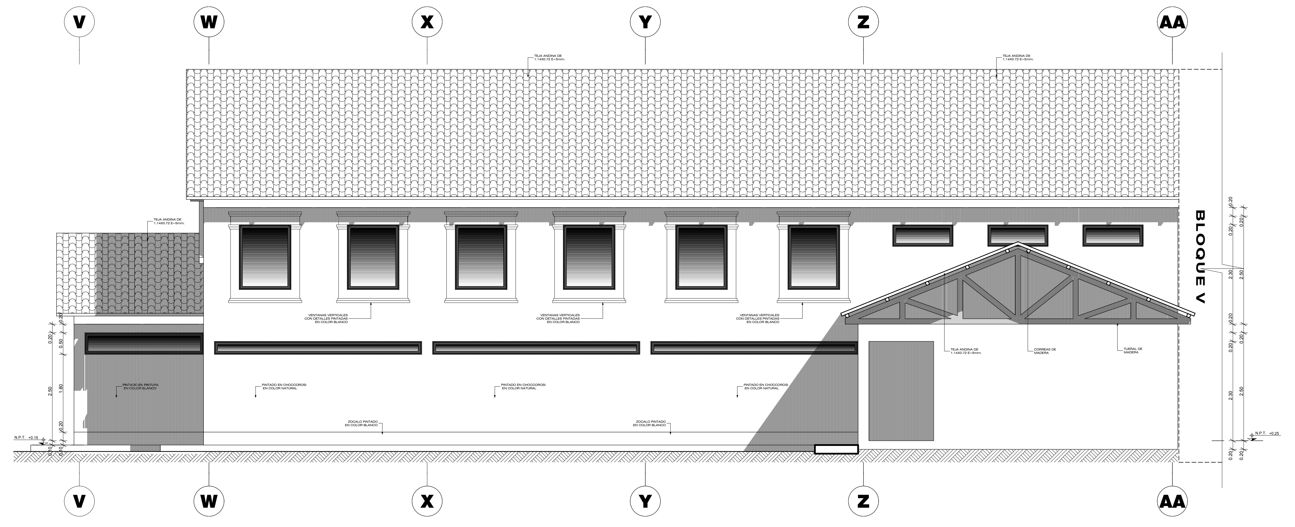
ELEVACION ESTE DEL BLOQUE VI ESCALA 1:50
