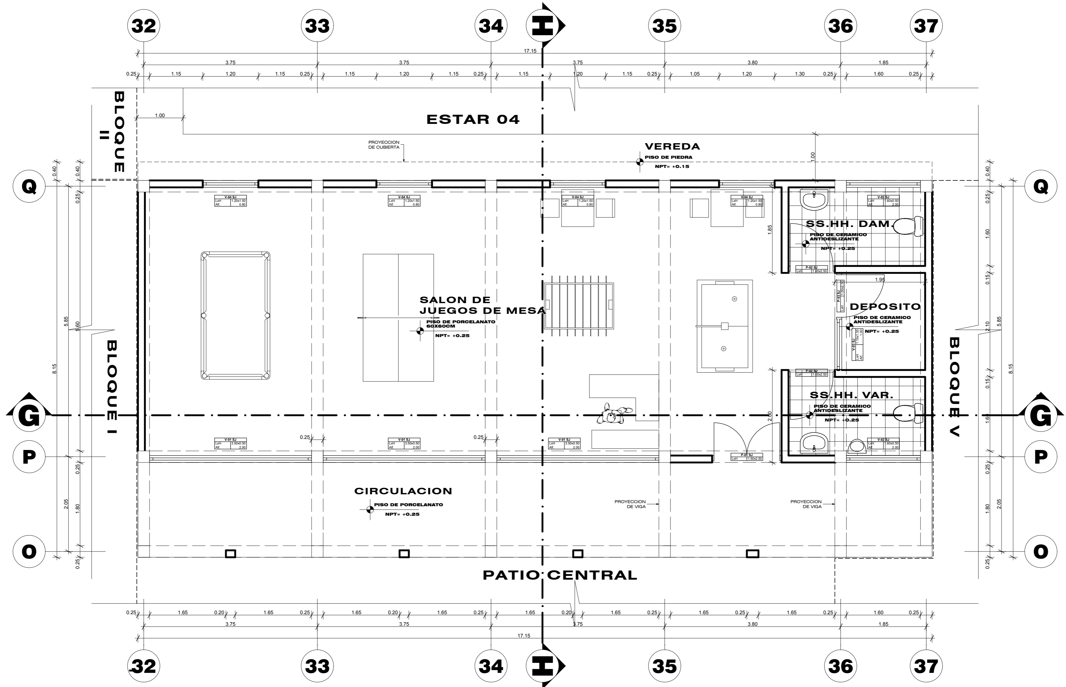
PLANTA DE DISTRIBUCION 1ER NIVEL BLOQUE IV
