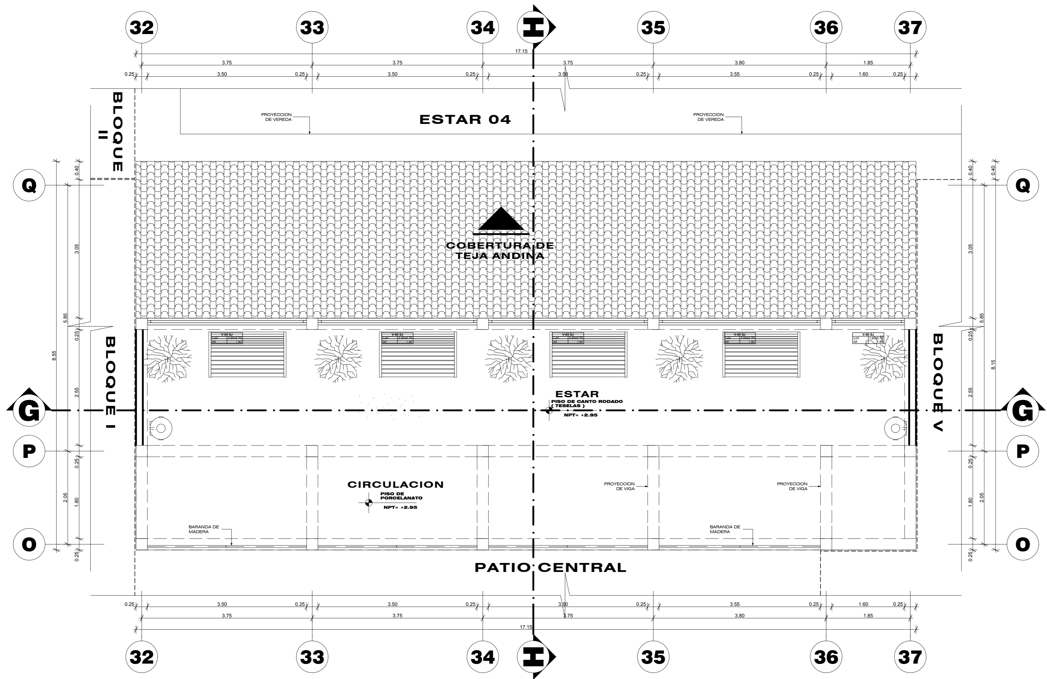
PLANTA DE DISTRIBUCION 2DO NIVEL BLOQUE IV
