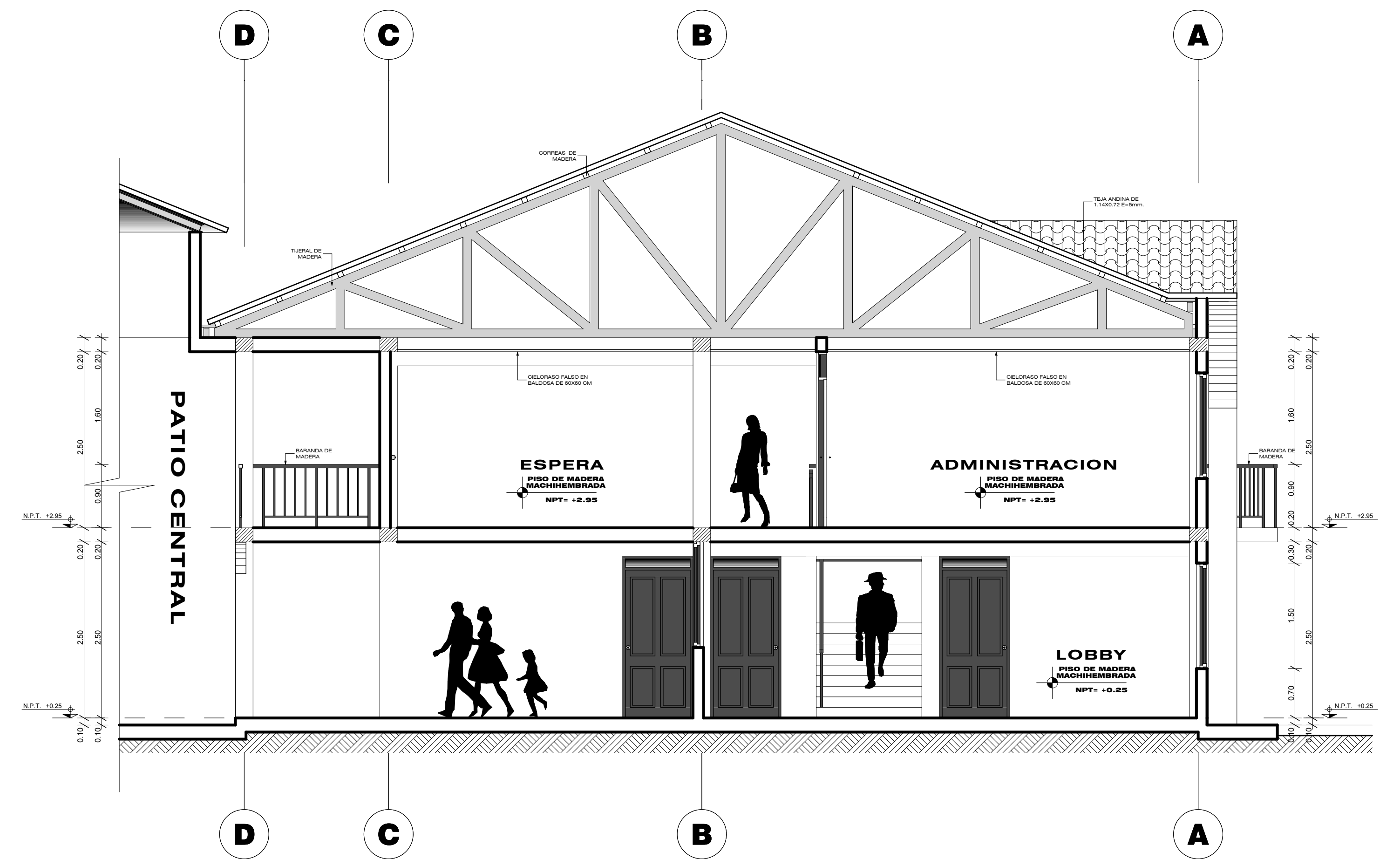
SECCION B-B DEL BLOQUE I ESCALA 1:50
