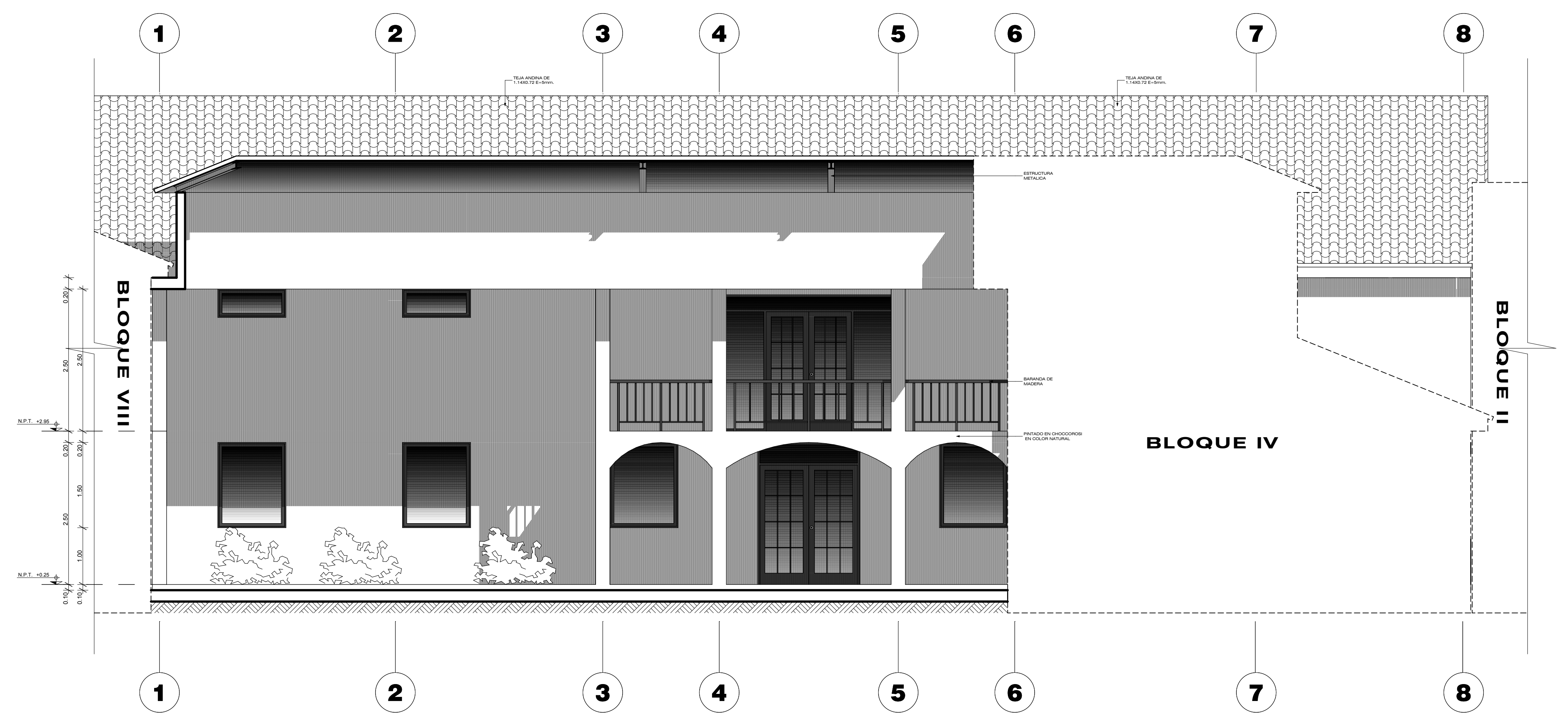
ELEVACION ESTE DEL BLOQUE I ESCALA 1:50
