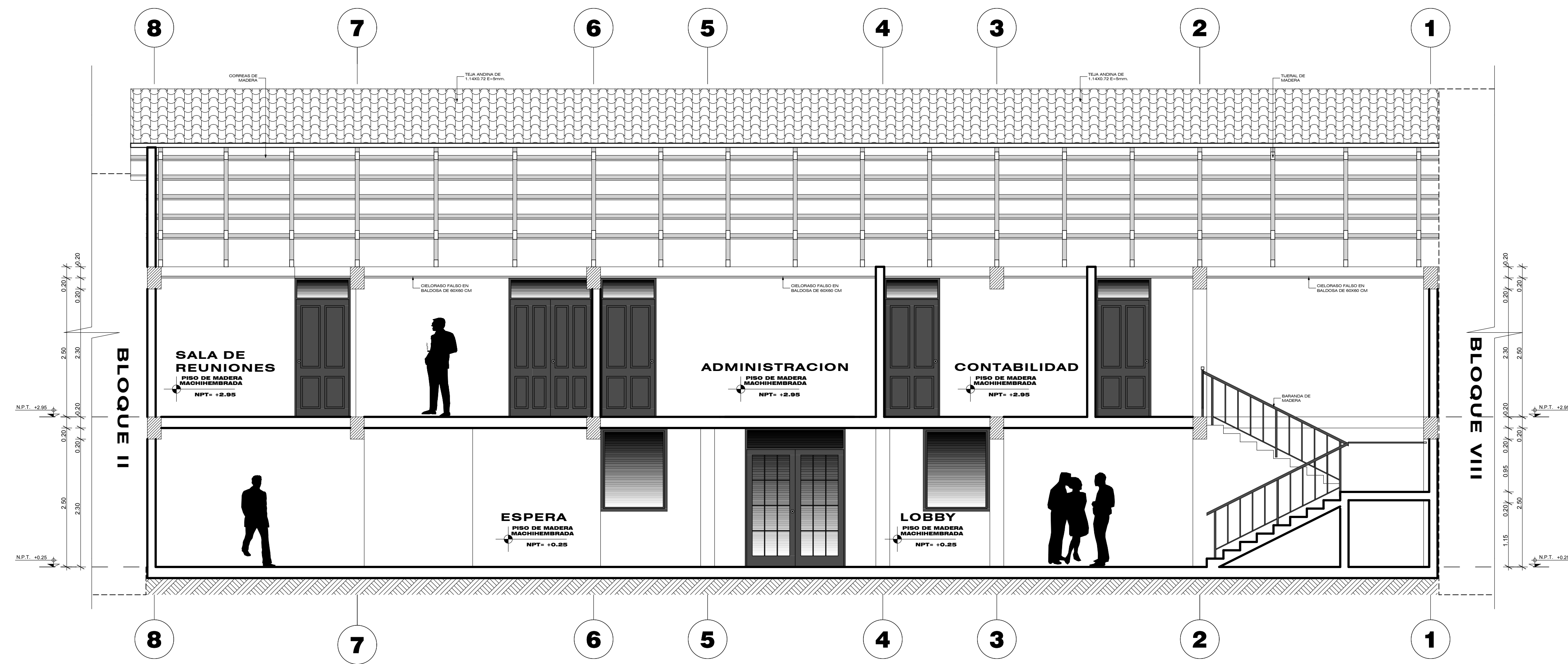
SECCION A-A DEL BLOQUE I ESCALA 1:50
