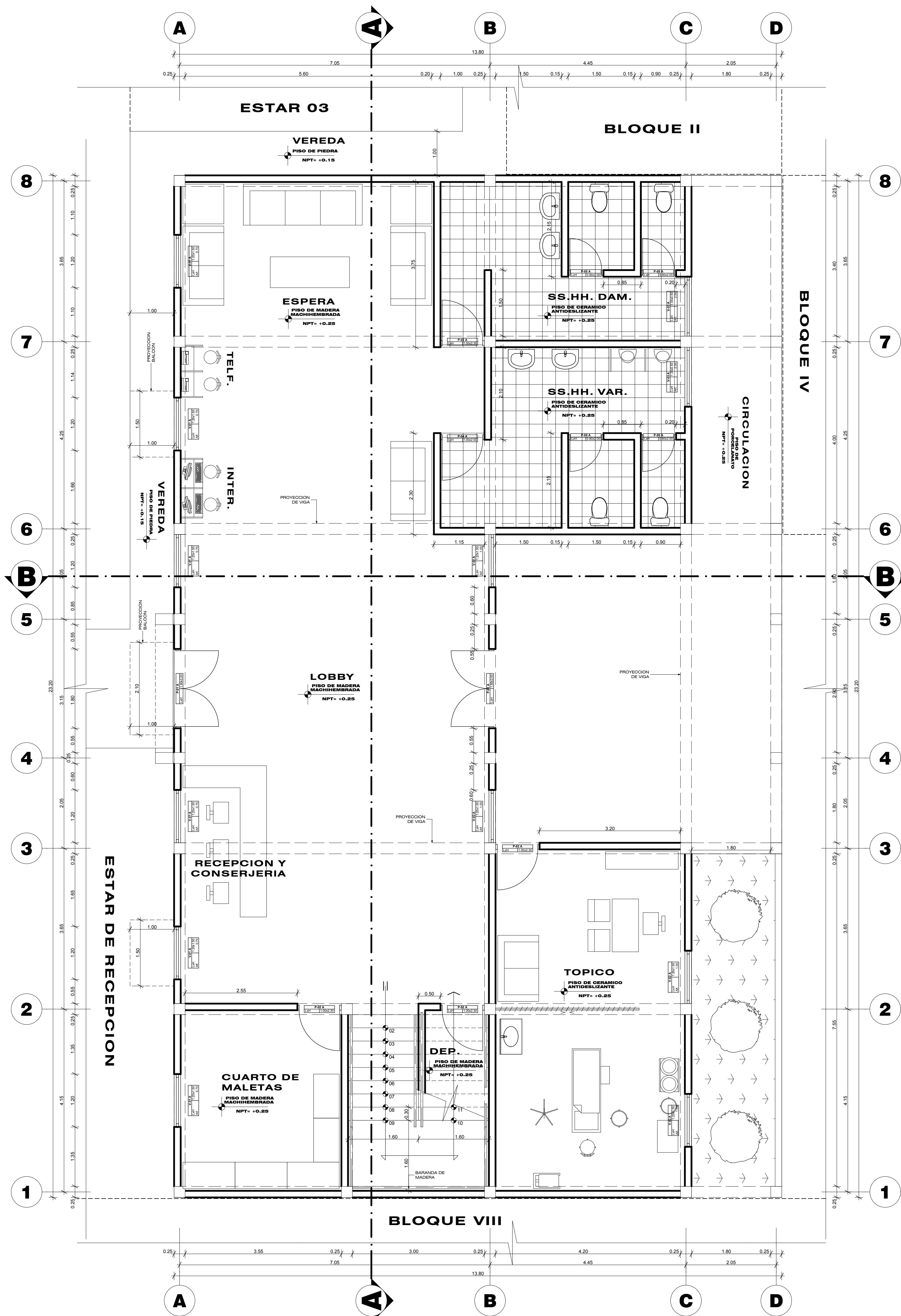
PLANTA DE DISTRIBUCION 1ER NIVEL BLOQUE I
