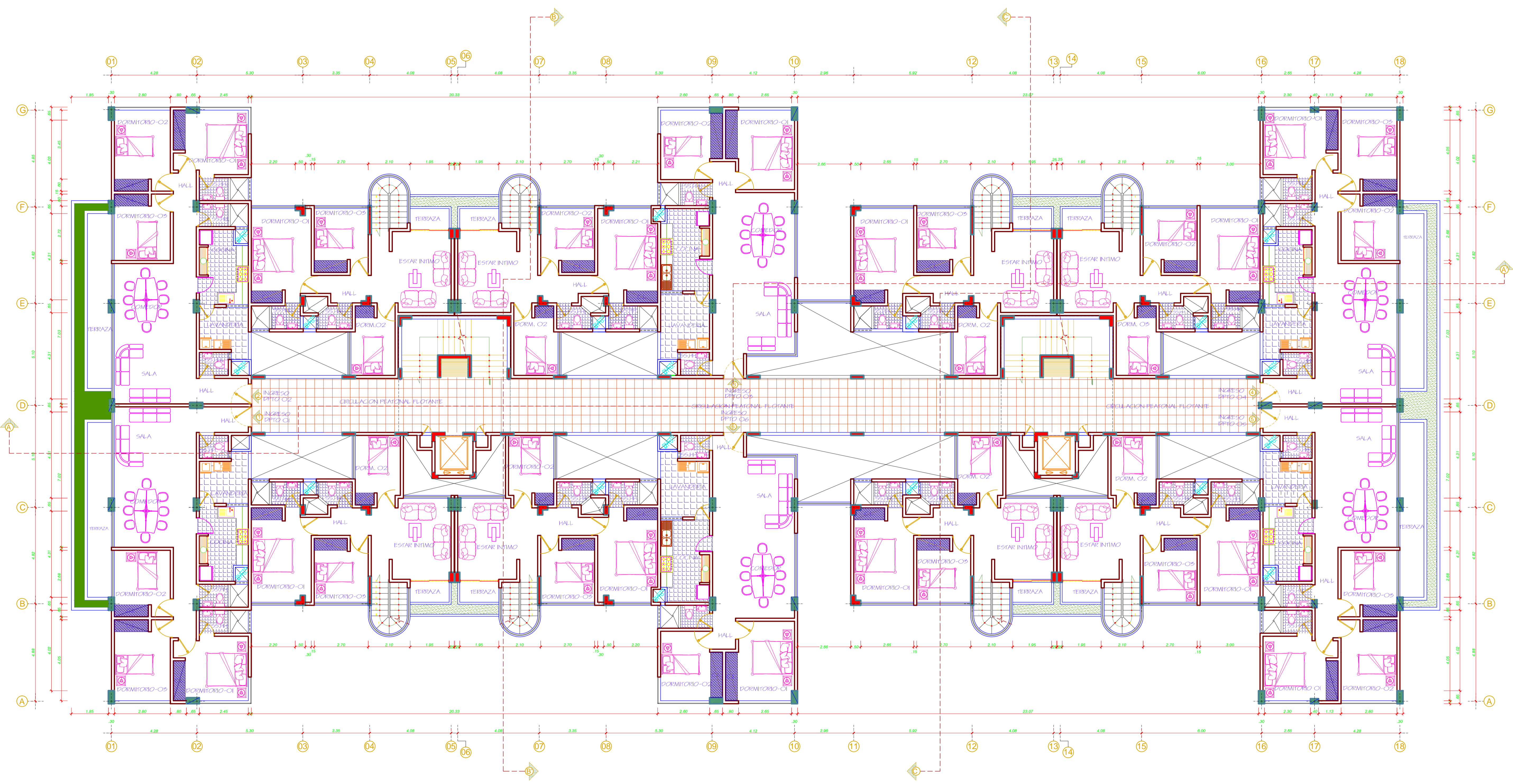
PLANTA: TIPICO 2DO, 4TO, 6TO PISO
