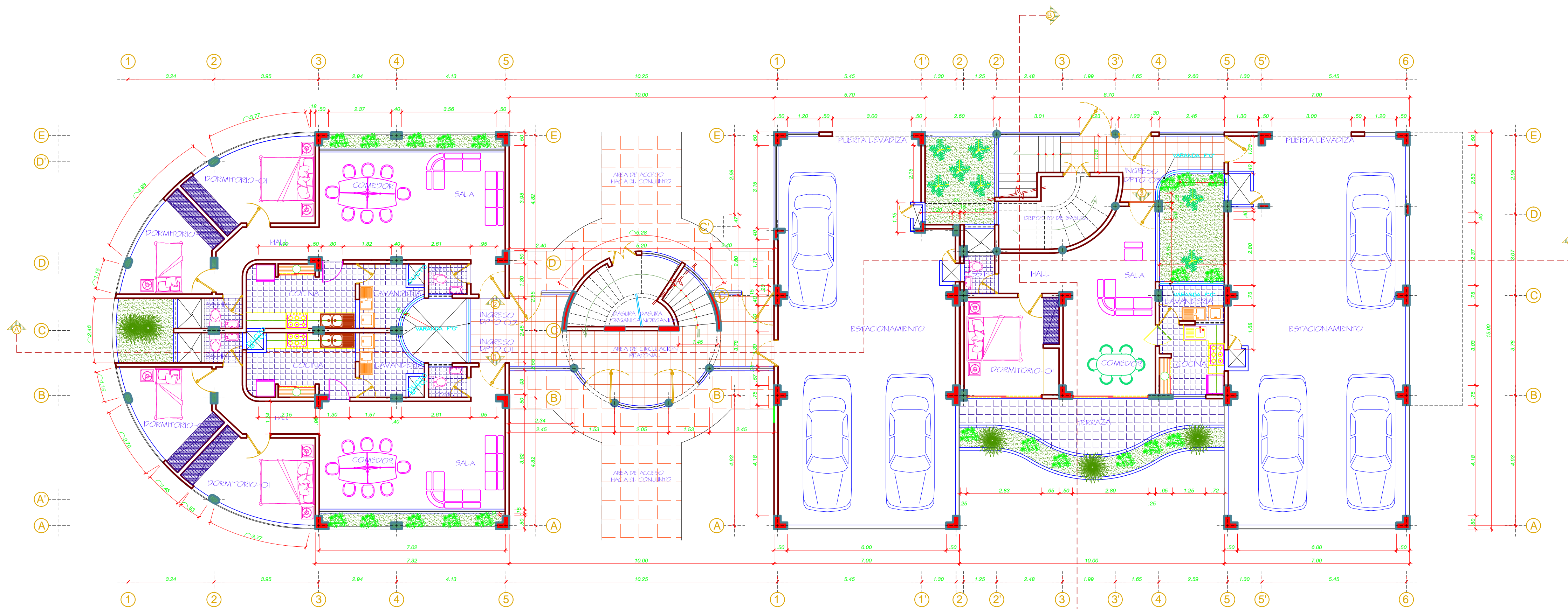
PLANTA: PRIMER PISO N.P.T. PRIMER PISO = ± 0.00 (NIVEL DE VEREDA) ESC: 1/100
