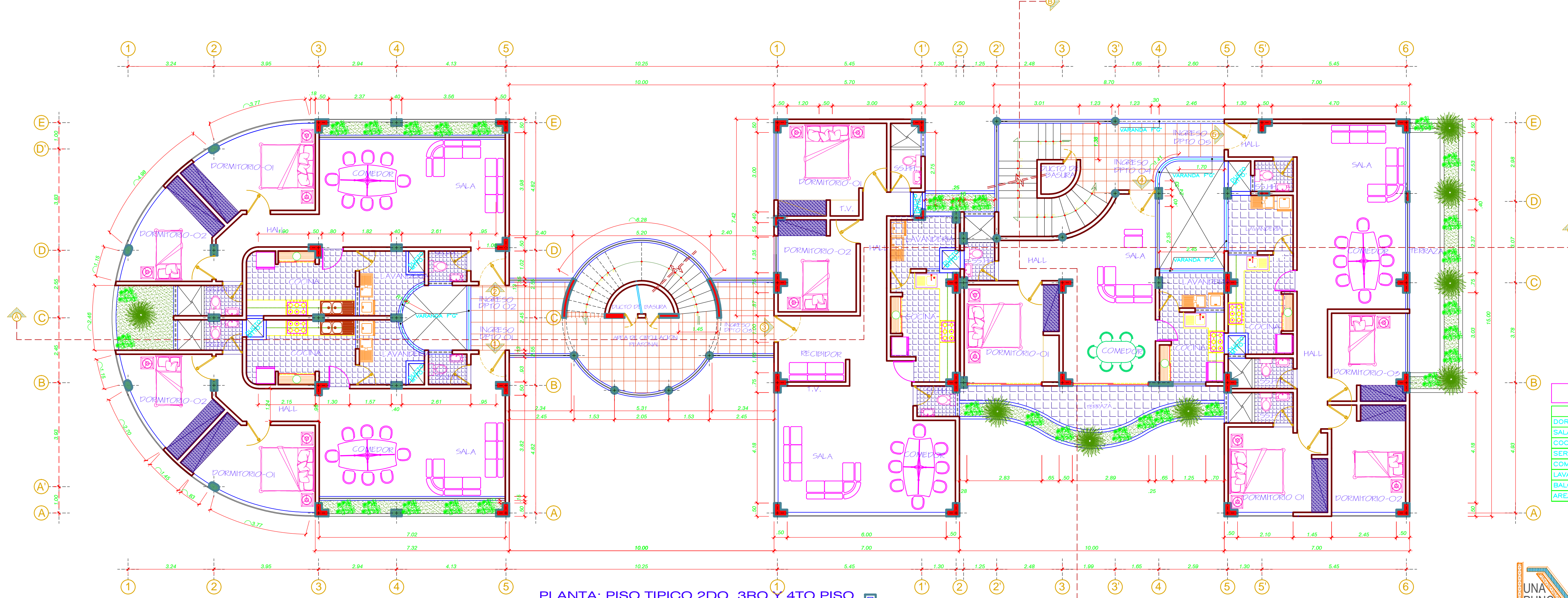
PLANTA: PISO TIPICO 2DO, 3RO Y 4TO PISO N.P.T. SEGUNDO PISO = + 3.06 N.P.T. TERCER PISO = + 6.12 N.P.T. CUARTO PISO = + 9.18 ESC: 1/100
