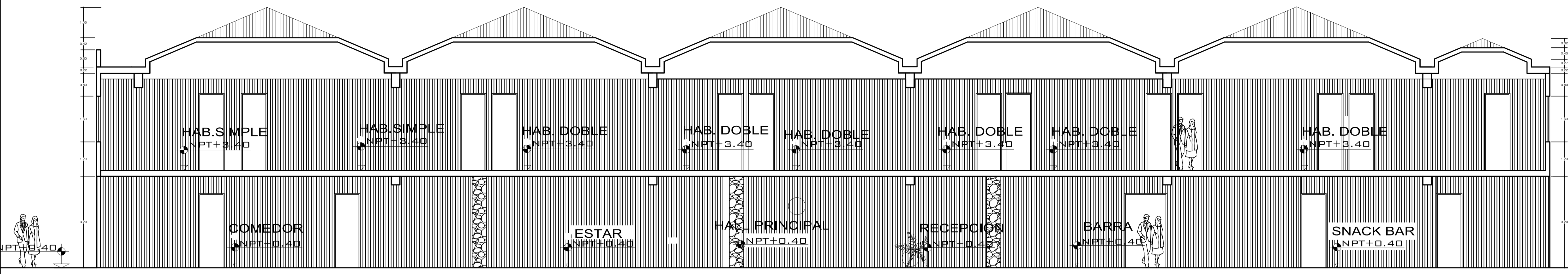
SECCION A-A PRIMER - SEGUNDO NIVEL HOSPEDAJE ESC: 1/75
