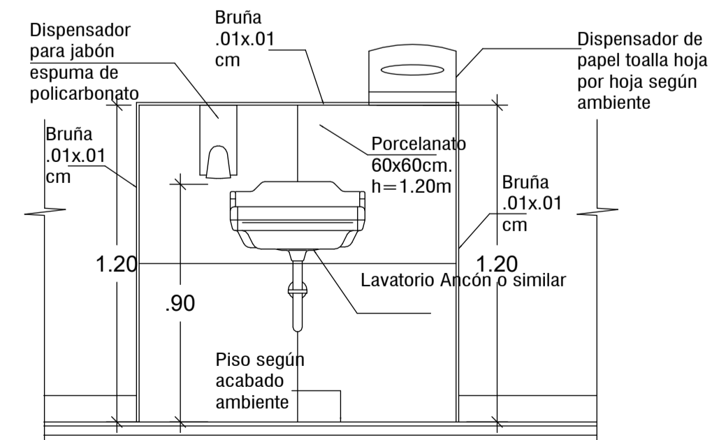
DETALLE MANDIL DE LAVATORIOS EN CONSULTORIOS E INTERNAMIENTO
