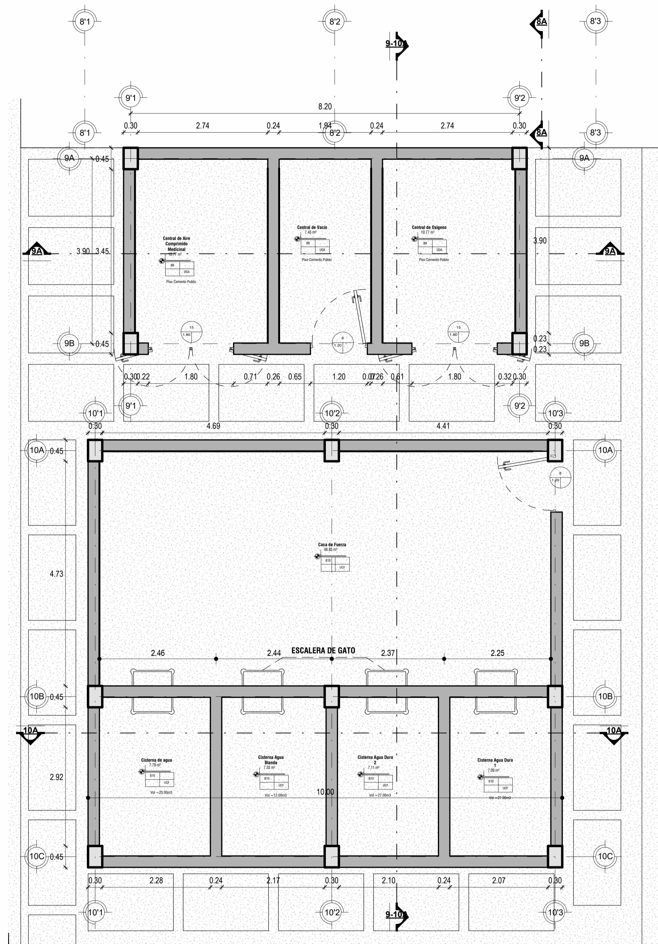
PLANO DISTRIBUCION BLOQUE 09
