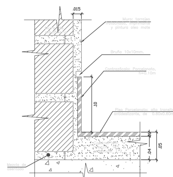
DET.02 ENCUENTRO DEL PISO PORCELANATO CON CONTRAZÓCALO DE PORCELANATO RECTO (PARA MUROS) ESC: 1/2,5
