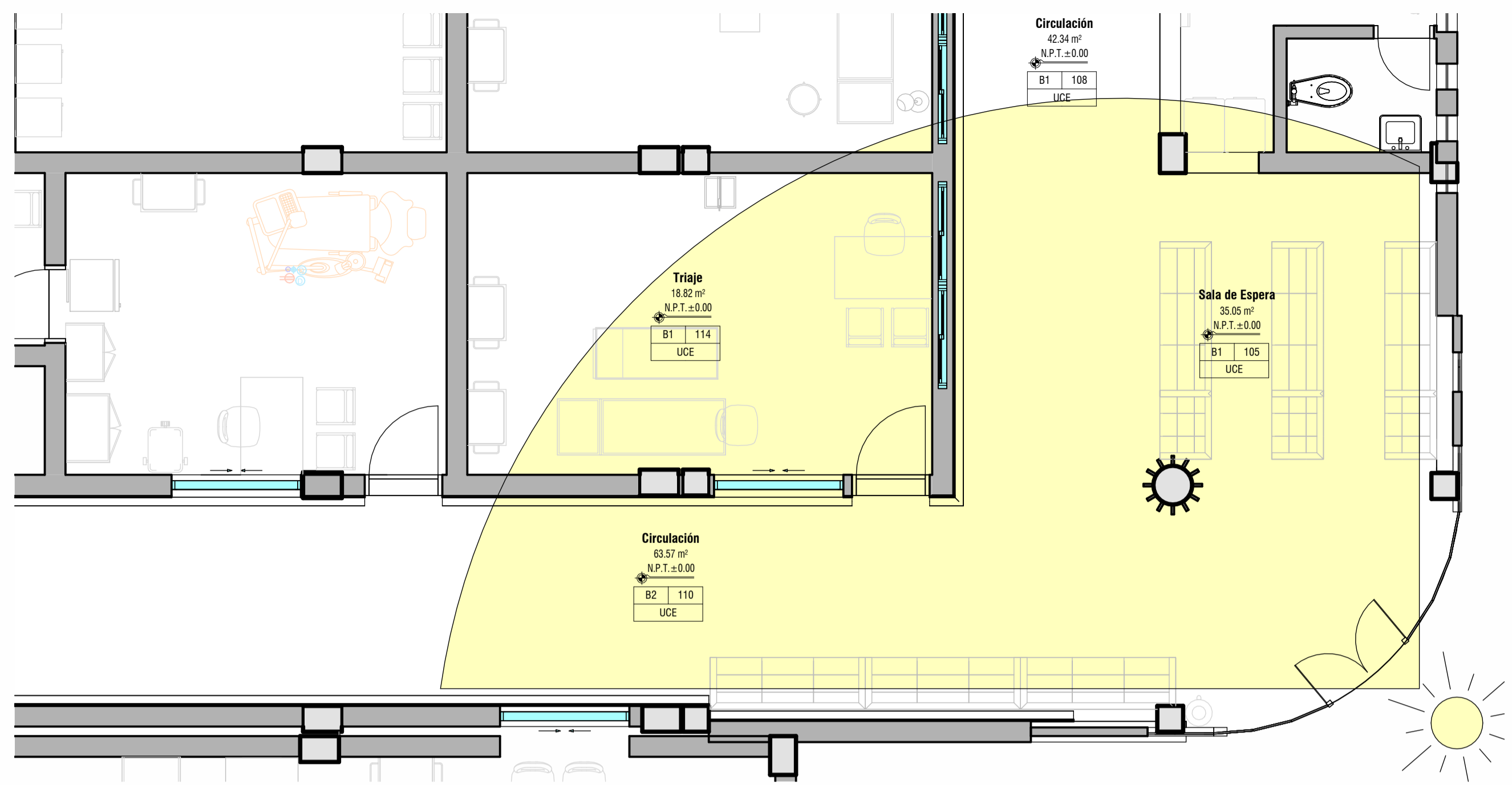
Iluminación 1.0
