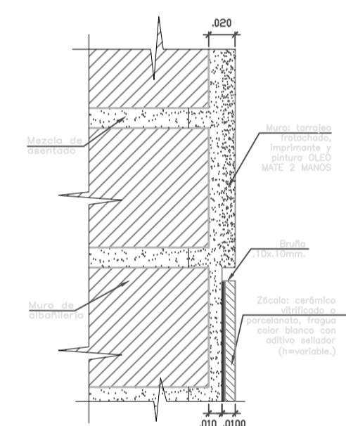
DET.09 ENCUENTRO ZÓCALO CERAMICO CON TARRAJEO Y PINTURA ESC: 1/2,5
