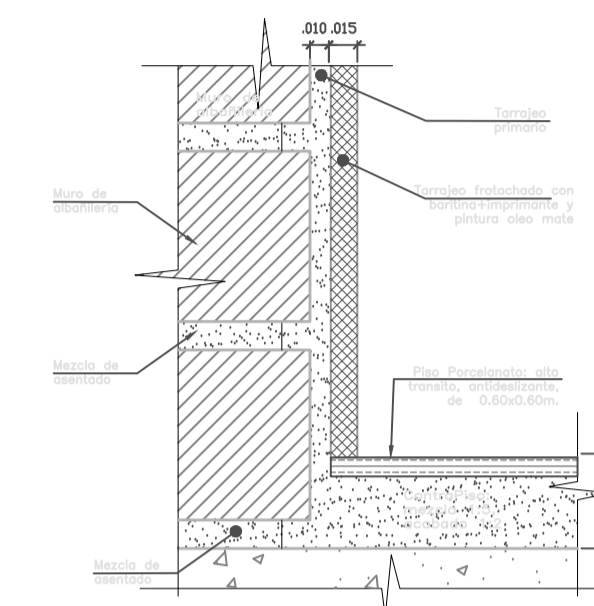
DET.05 ENCUENTRO DEL PISO DE PORCELANATO CON TARRAJEO CON BARRINA ESC: 1/2,5
