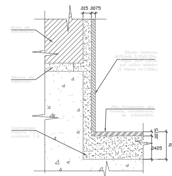
DET.04 ENCUENTRO DEL PISO DE PORCELANATO CON ZÓCALO DE CERAMICO ESC: 1/2,5
