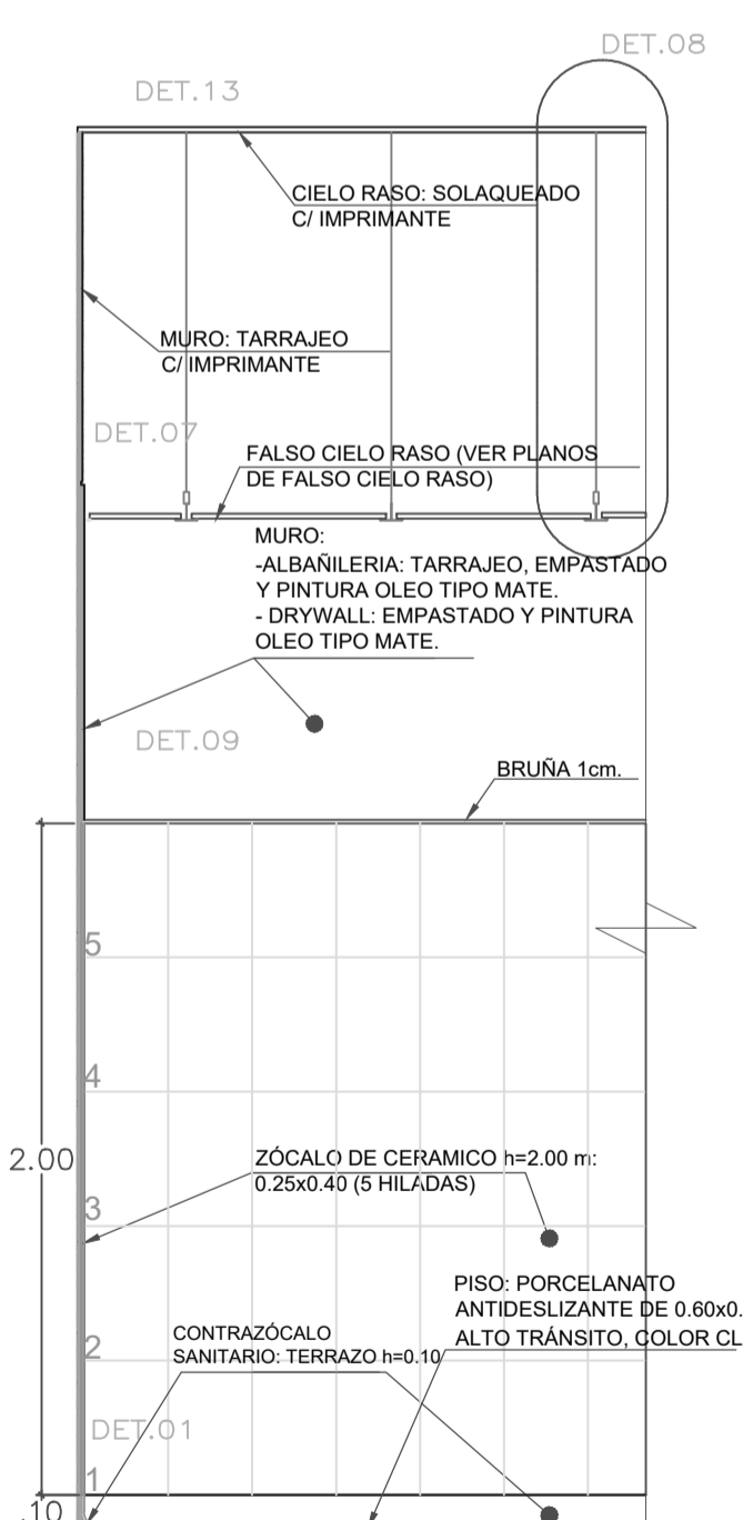
DETALLE DE ACABADO DE INT. RESIDUOS SÓLIDOS - A.I. RESIDUOS SÓLIDOS- ALM. I. DE RESIDUOS SÓLIDOS- INT. RESIDUOS SÓLIDOS.
