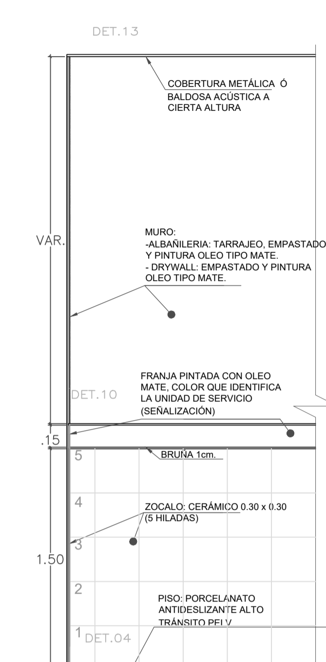
DETALLE DE ACABADO DE CORREDOR TECNICO
