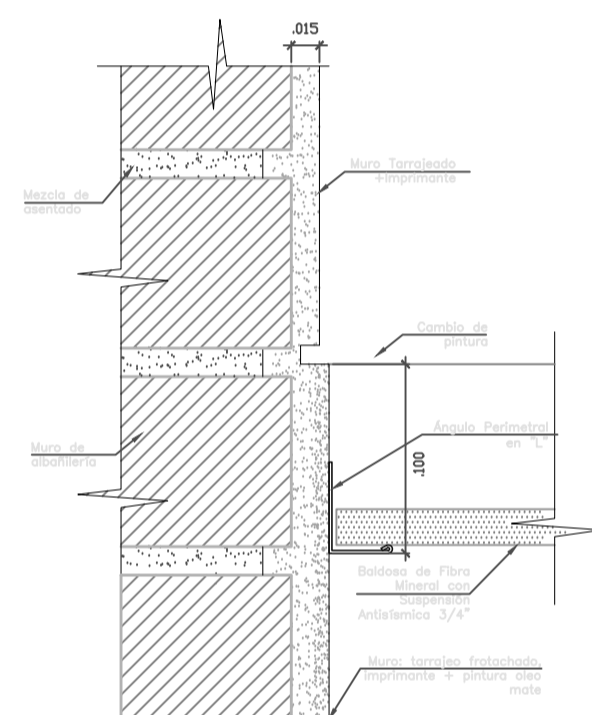
DET.07 ENCUENTRO MURO DE 2cm Y FALSO CIELO RASO (Baldosa de fibra mineral) ESC: 1/2,5
