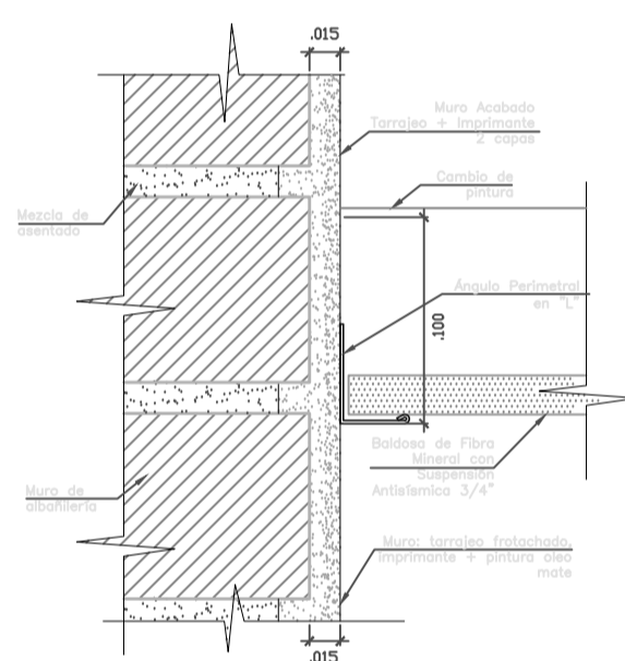
DET.06 ENCUENTRO MURO DE 1,5cm Y FALSO CIELO RASO (Baldosa de fibra mineral) ESC: 1/2,5
