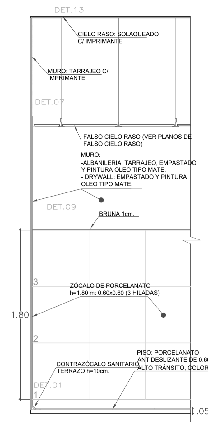
DETALLE DE ACABADO DE TOMA DE MUESTRAS
