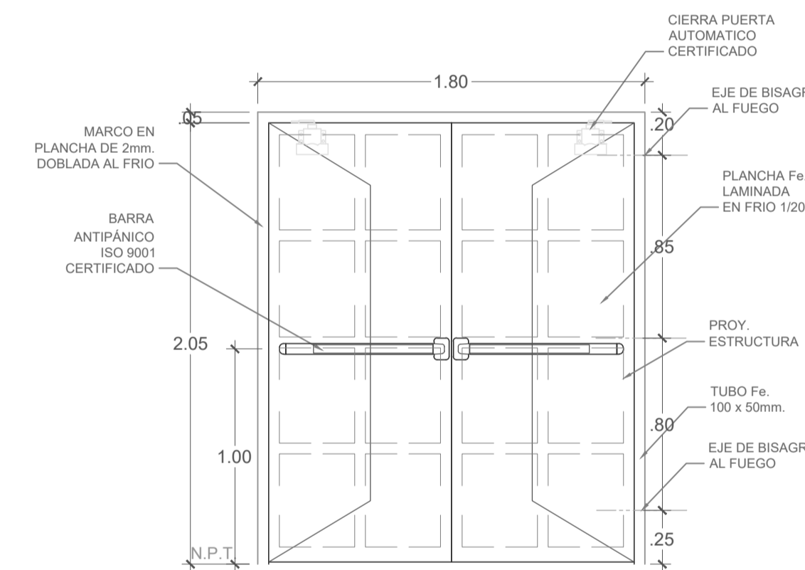
Pa-03 (1.80 x 2.10) ESC.:1/25
