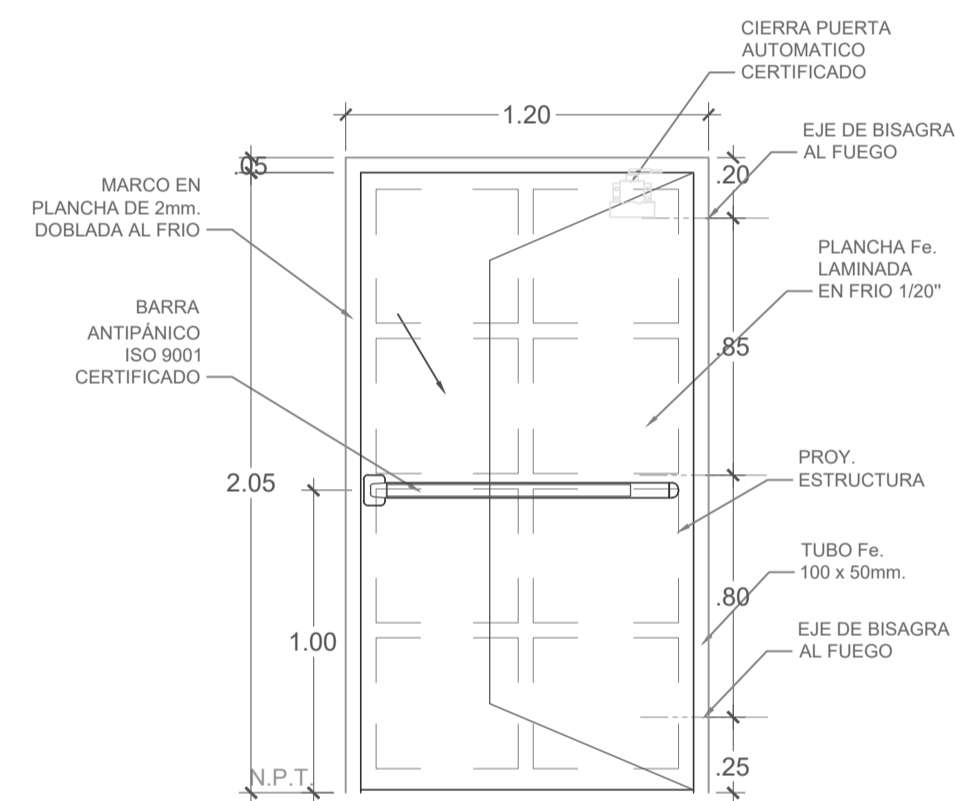
Pa-01 (1.20 x 2.10) ESC.:1/25
