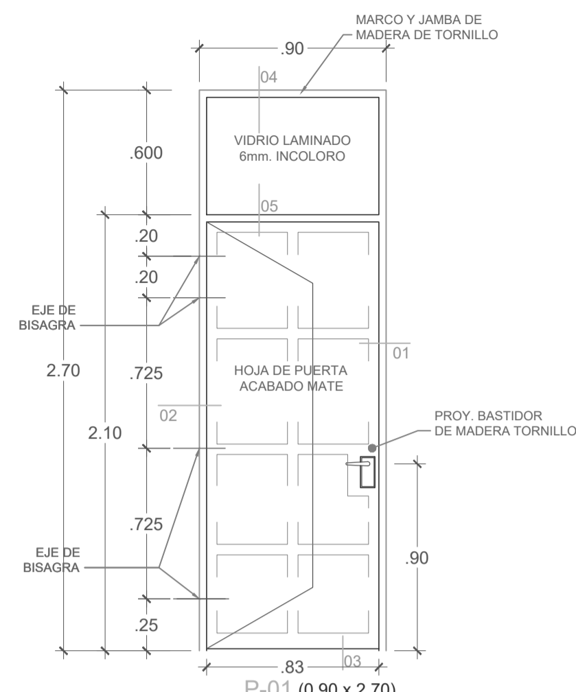
P-01 (0.90 x 2.70) ESC.:1/25
