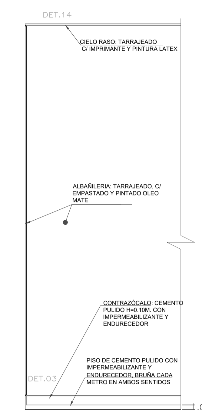
DETALLE DE ACABADO DE UPS CASA DE FUERZA II- CUARTO CLOSET II.EE 02- GRUPO ELECTROGENO PARA SUB ESTACION ELÉCTRICA- SUB ESTACION ELÉCTRICA- GEN. BAJA TENSIÓN/C. TÉCNICO- DE EQ. BIOMEDICOS/IT. MANTENIMIENTO Y PINTURA
