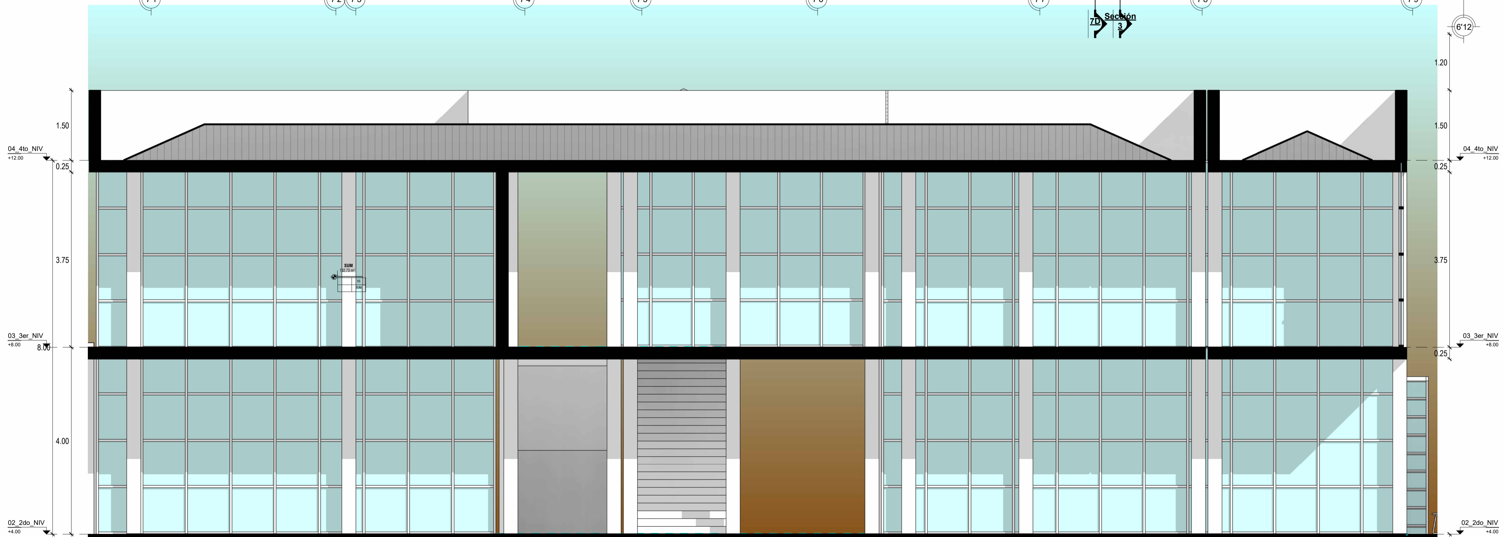
SECCION 7A-7A
