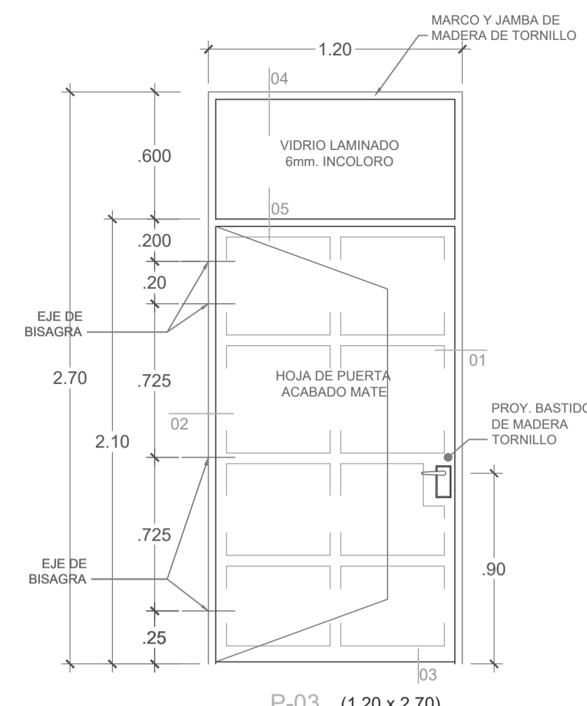
P-03 (1.20 x 2.70) ESC.:1/25
