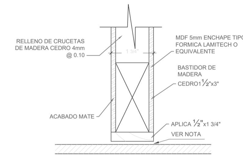
CORTE 03 ESC.:1/25
