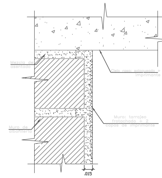
DET.13 ENCUENTRO MURO CON CIELO RASO ESC: 1/2,5
