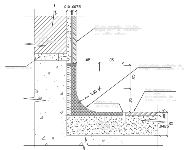
DET.01 ENCUENTRO DE PISO CERAMICO CON ZÓCALO DE CERAMICO Y CONTRAZÓCALO SANITARIO DE CERAMICO (PARA MUROS) ESC: 1/2,5
