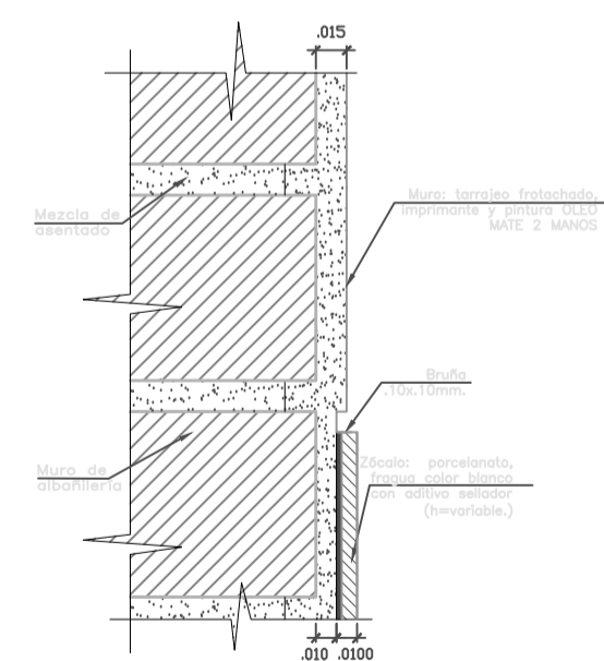
DET.12 ENCUENTRO ZÓCALO CERAMICO CON TARRAJEO Y PINTURA ESC: 1/2,5
