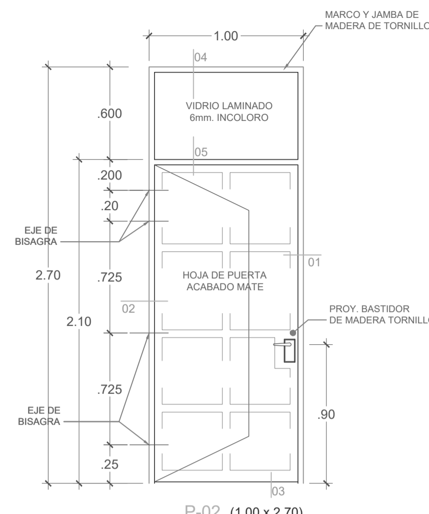
P-02 (1.00 x 2.70) ESC.:1/25
