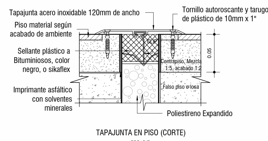
TAPAJUNTA EN PISO (CORTE)
