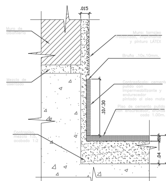
DET.03 ENCUENTRO PISO DE CEMENTO PULIDO CON CONTRAZÓCALO DE CEMENTO ESC: 1/2,5
