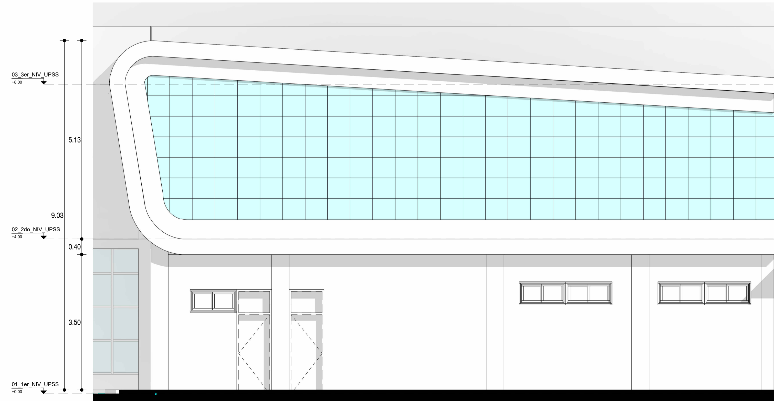
Elevación B3 1 : 50
