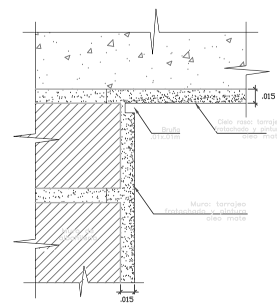
DET.14 ENCUENTRO MURO CON CIELO RASO ESC: 1/2,5
