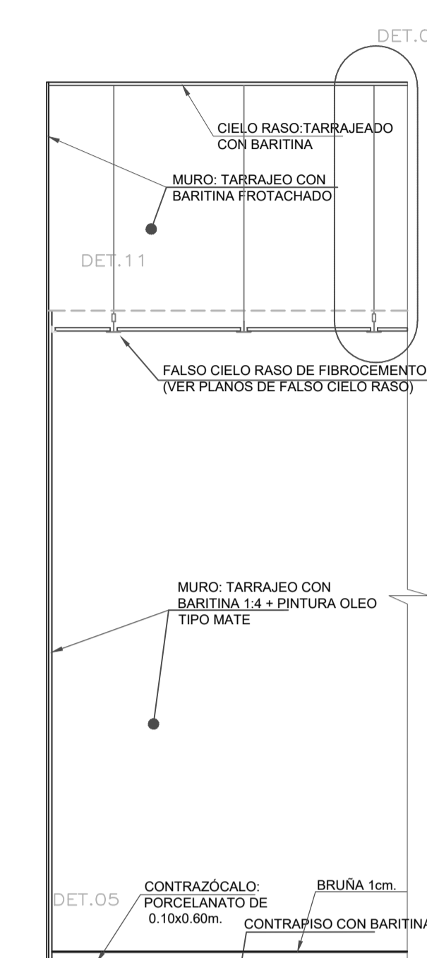
DETALLE DE ACABADO DE SOPORTE RADIOLOGÍA
