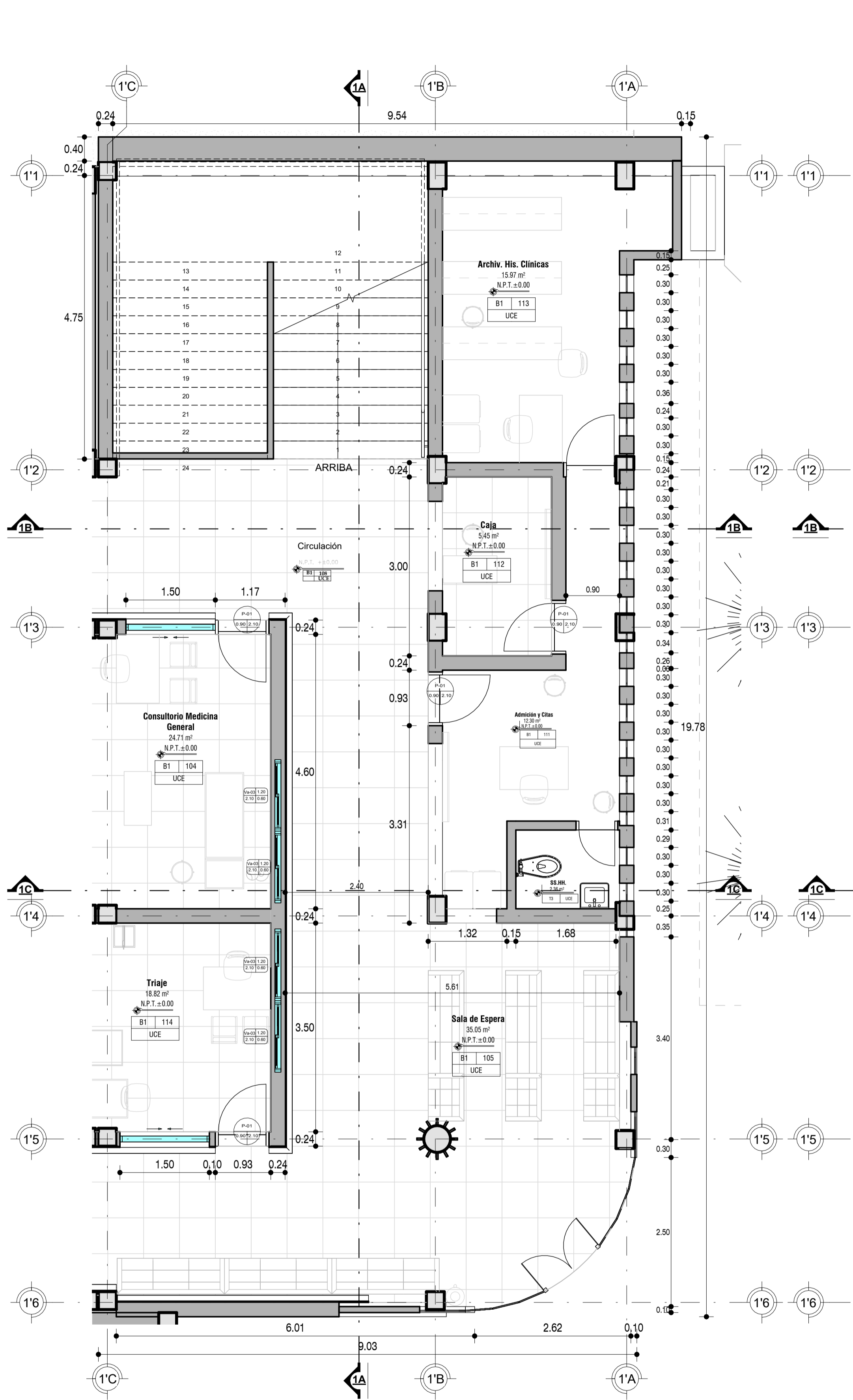
01_1er_Niv_Bloque 01
