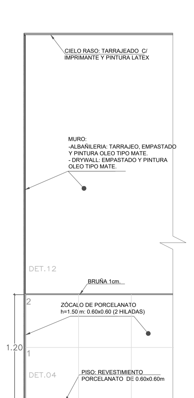
DETALLE DE ACABADO DE BAÑOS DE GUARDIANIA
