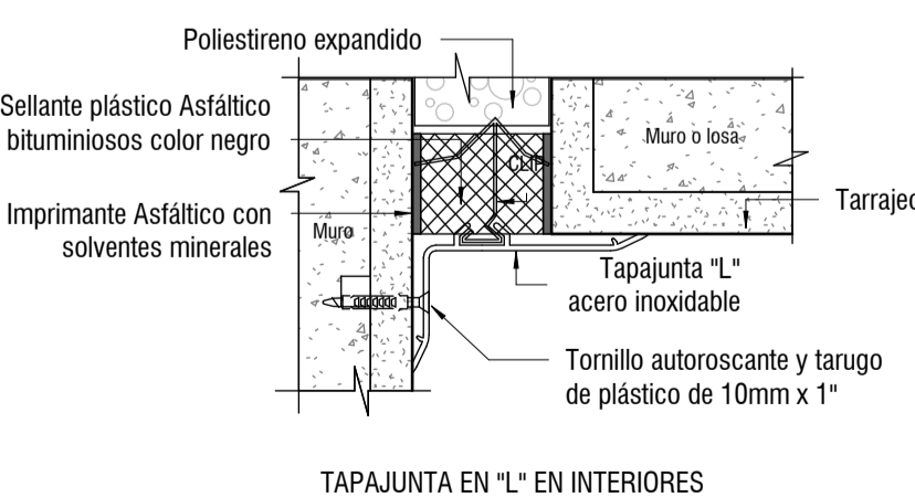
TAPAJUNTA EN 'L' EN INTERIORES ESC: 5/8
