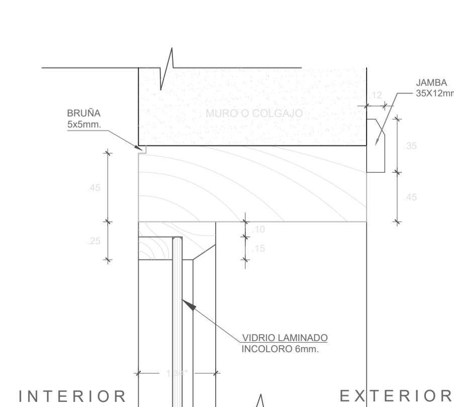
CORTE 04 ESC.:1/25
