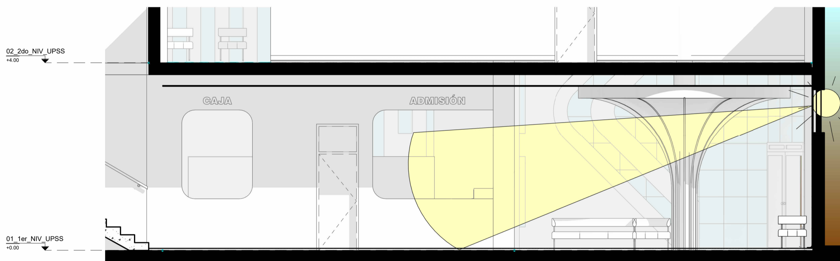
Sección Iluminación 1.0
