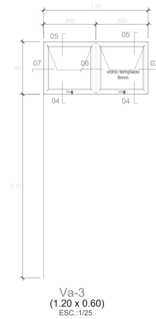
VENTANA DE ALUMINIO CON CRISTAL
