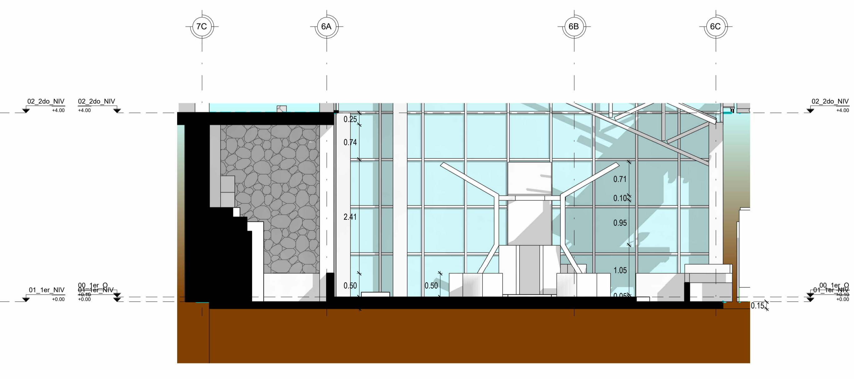
SECCION JC 1 : 50
