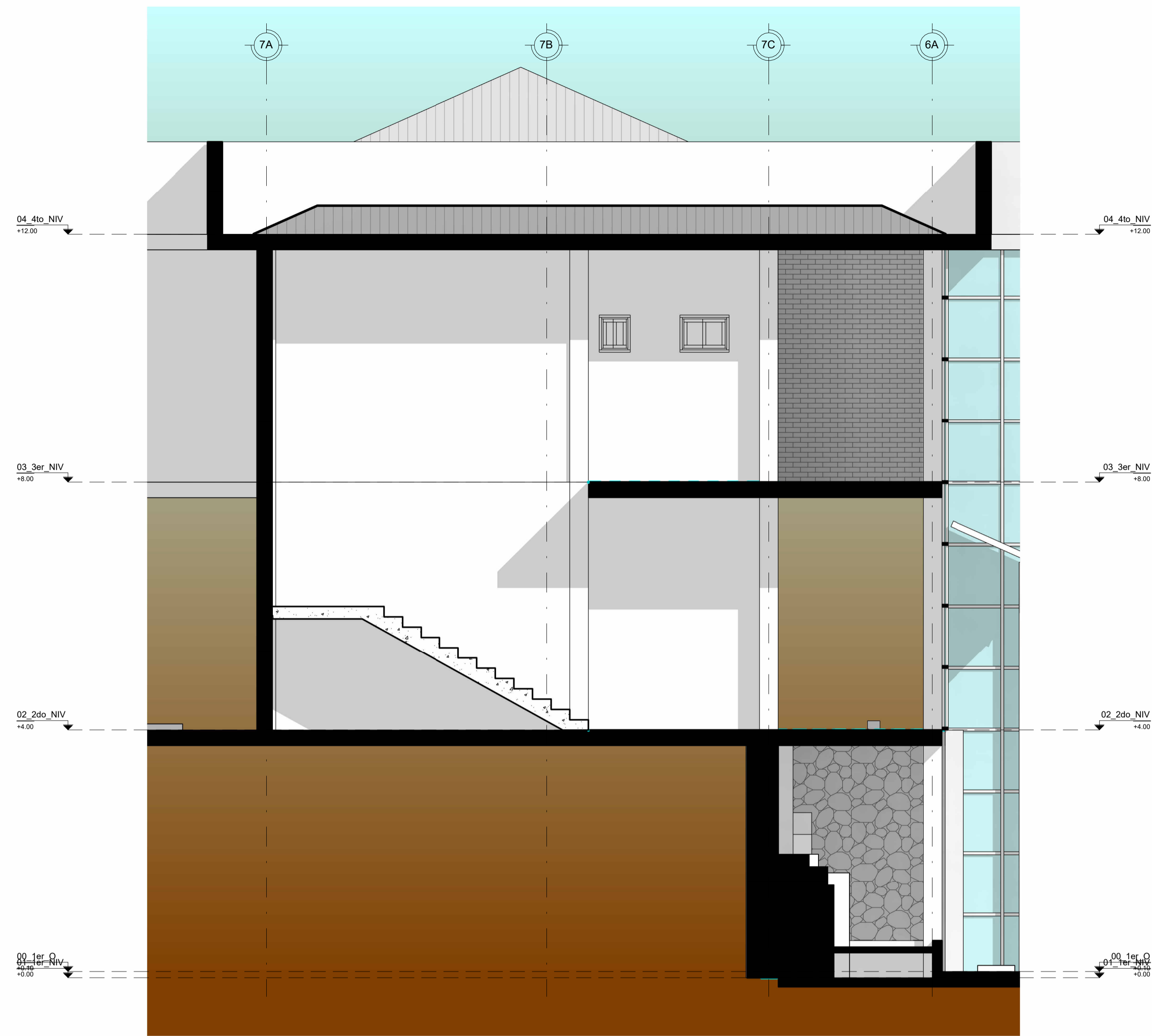
SECCION 7C
