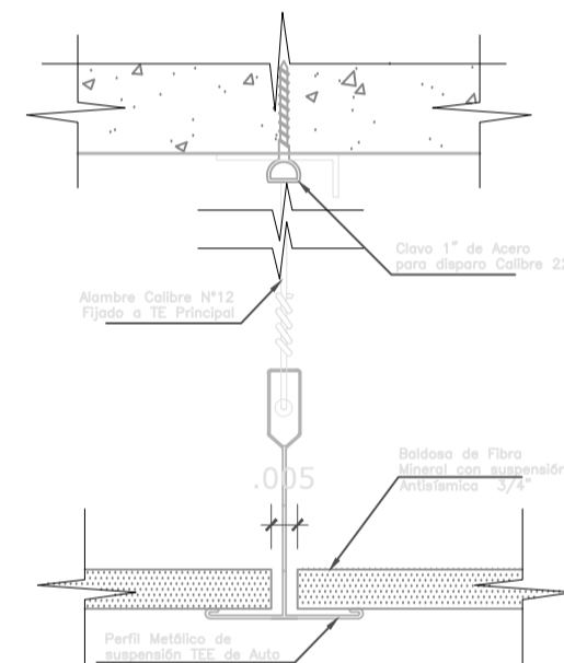
DET.08 ENCUENTRO MURO Y FALSO CIELO RASO (Baldosa de fibra mineral) ESC: 1/2,5
