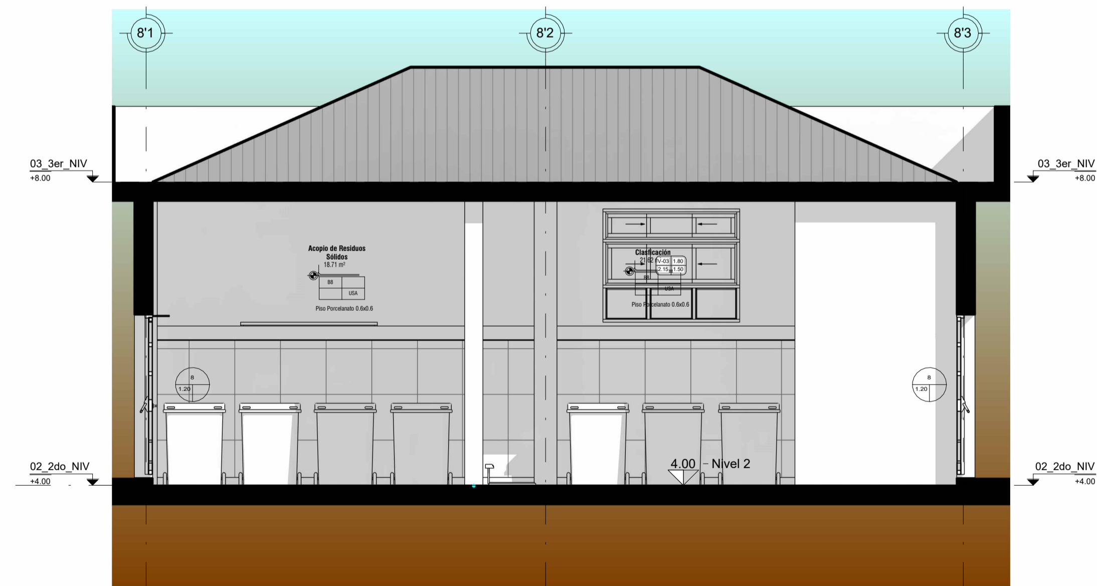
SECCION 8B
