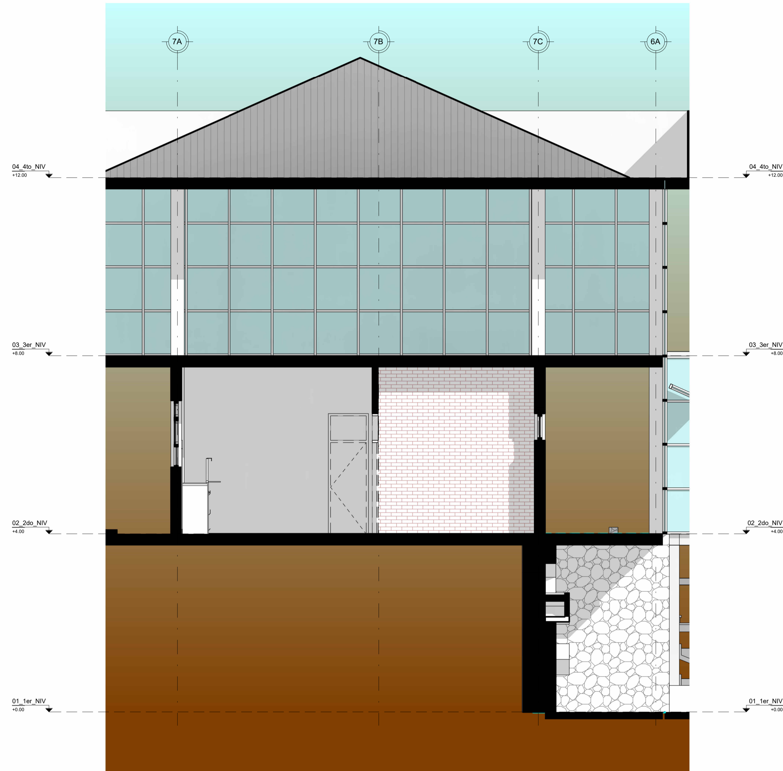
SECCION 7D
