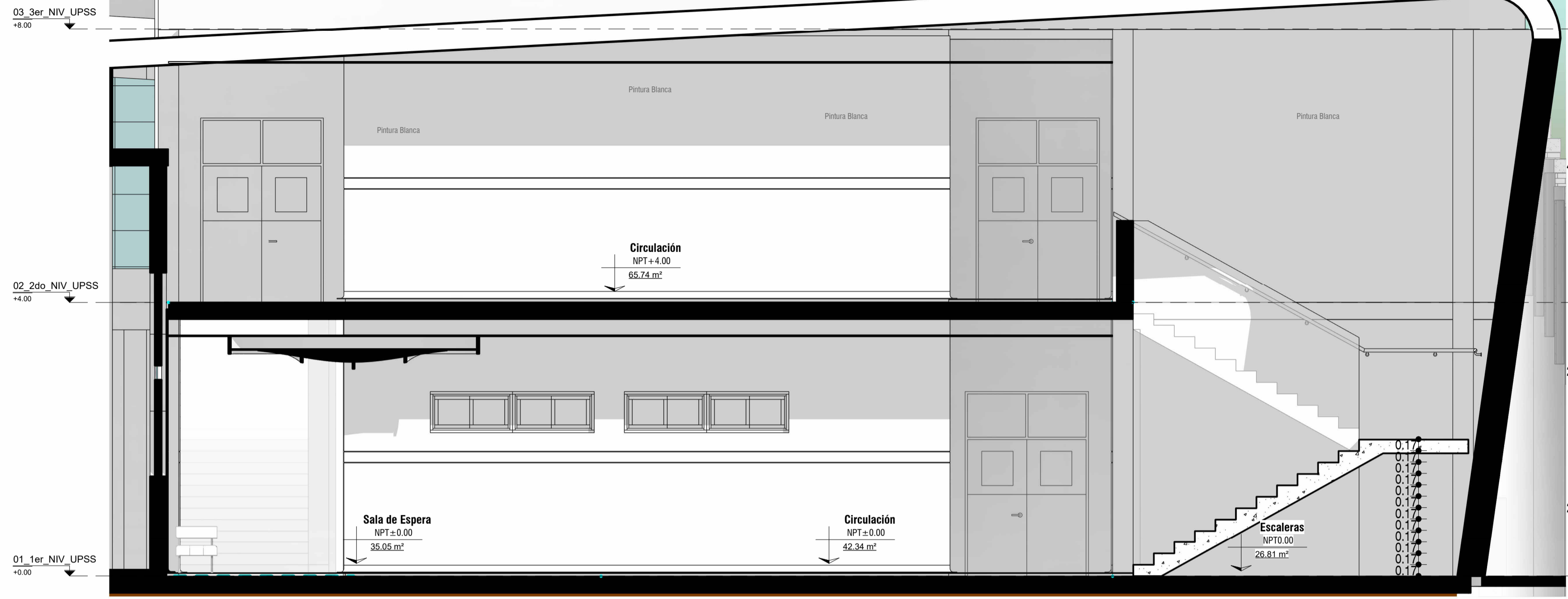
1A - 1A
