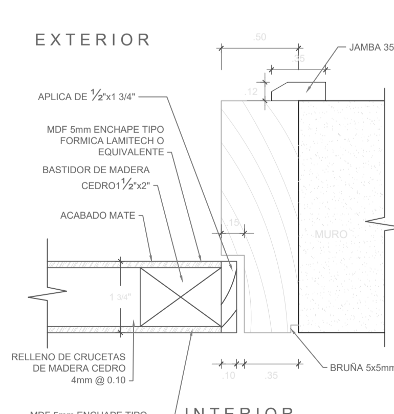
CORTE 01 ESC.:1/25
