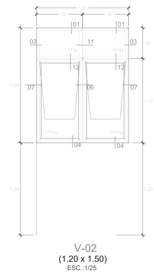
VENTANA DE ALUMINIO CON CRISTAL
