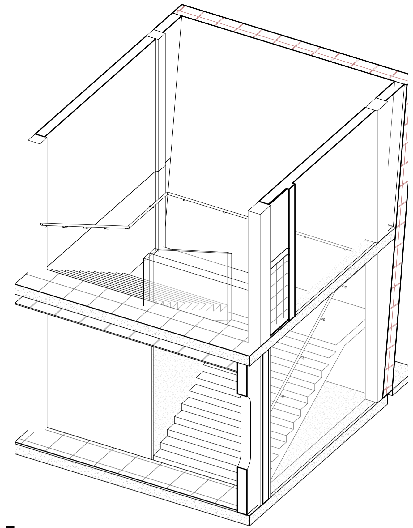
Isométrico gradas
