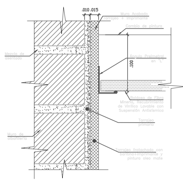
DET.11 ENCUENTRO MURO CON BARRINA Y FALSO CIELO RASO FIBROCEMENTO ESC: 1/2,5
