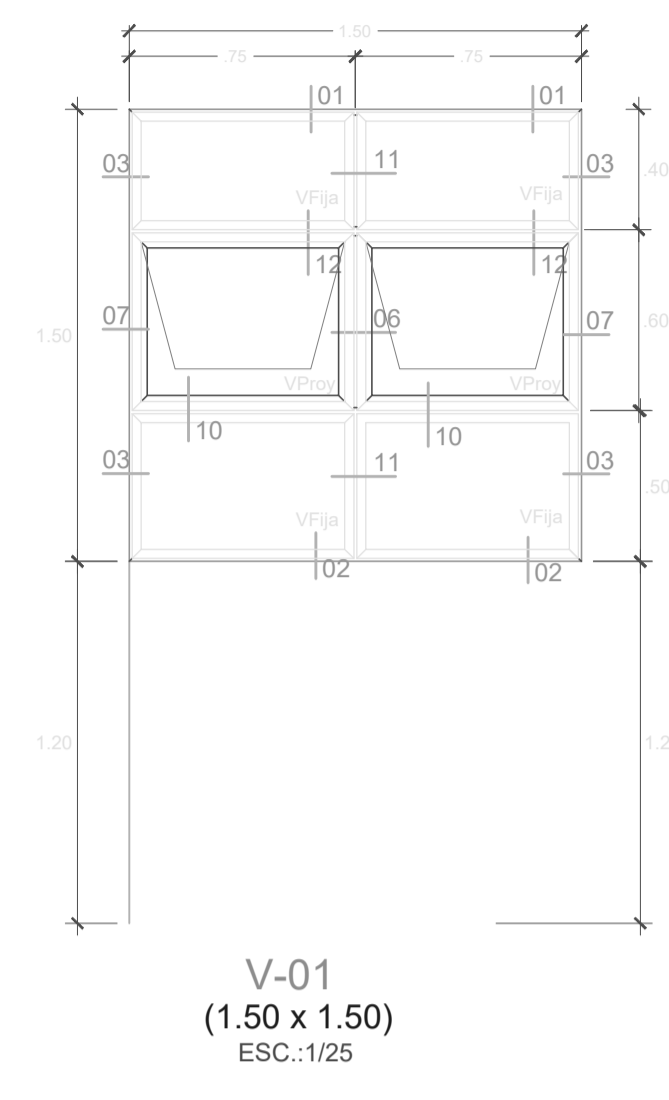
VENTANA DE ALUMINIO CON CRISTAL
