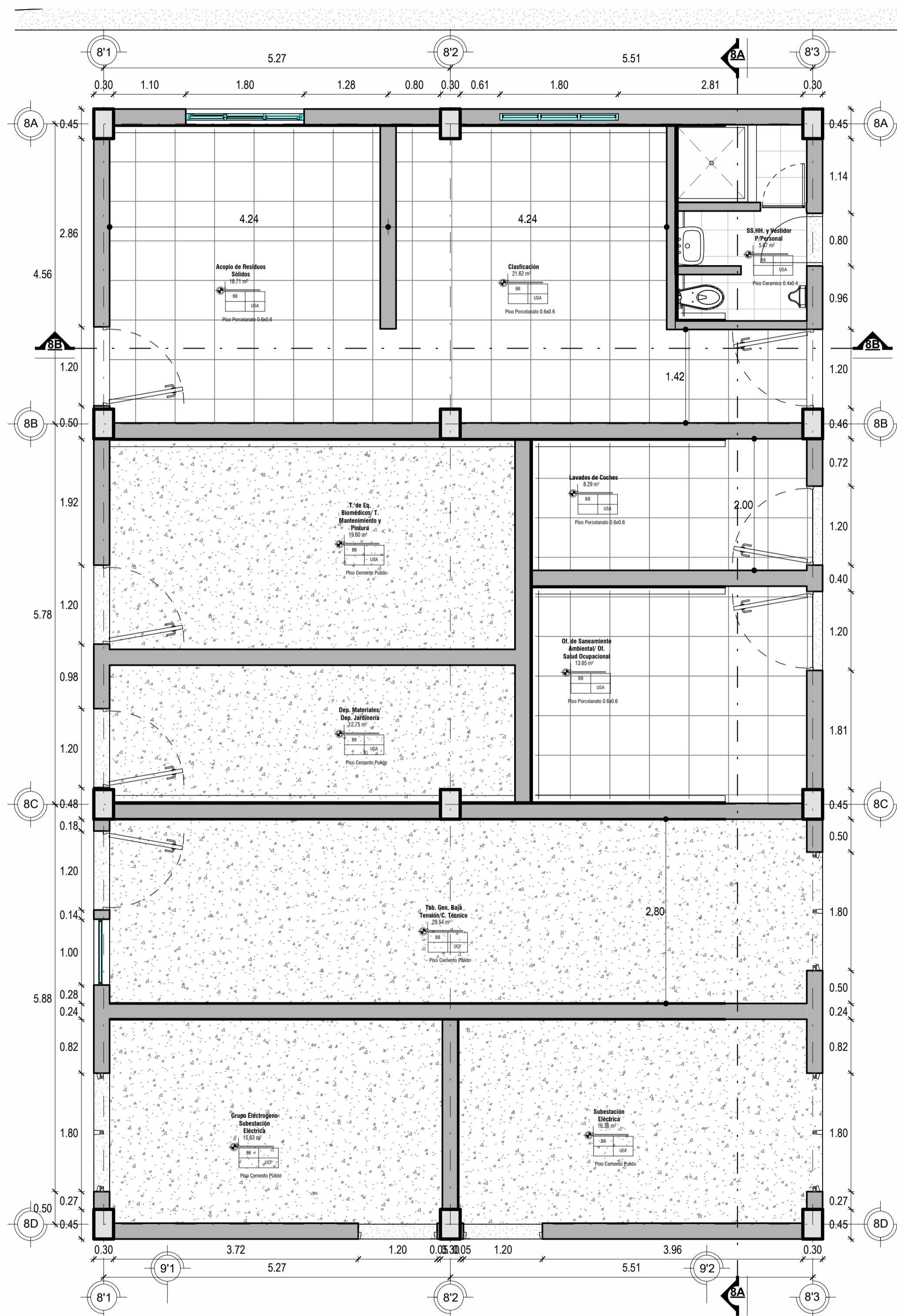
PRIMER NIVEL_BLOQUE 08
