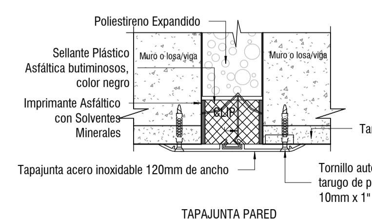
TAPAJUNTA PARED ESC: 1/2,5
