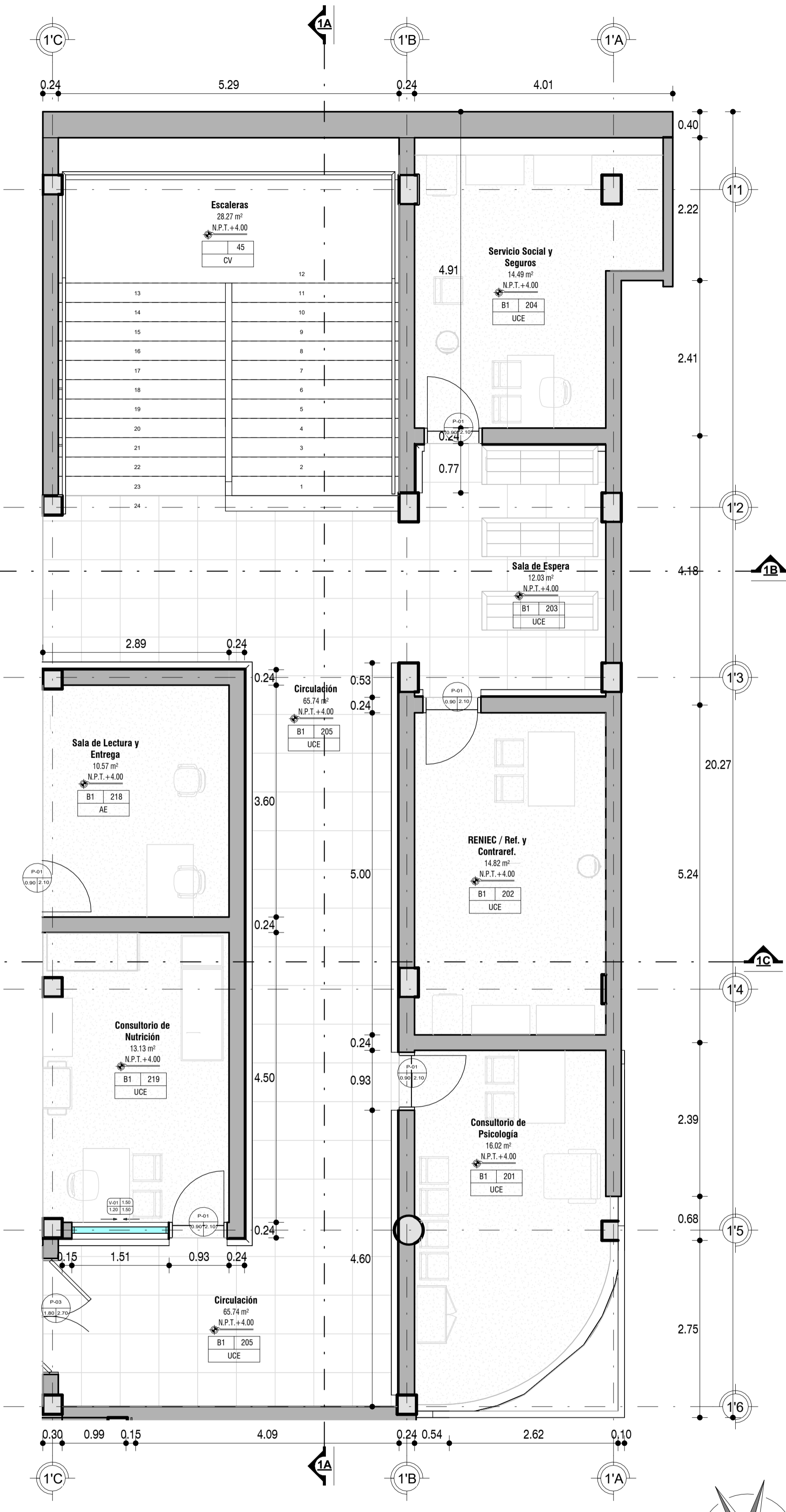
02_2do_Niv_Bloque 01
