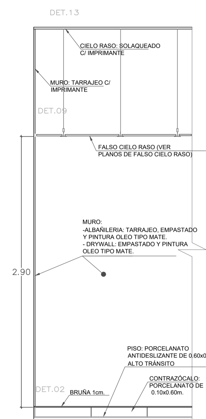
DETALLE DE ACABADO DE ADMINISTRACION Y ALMACÉN
