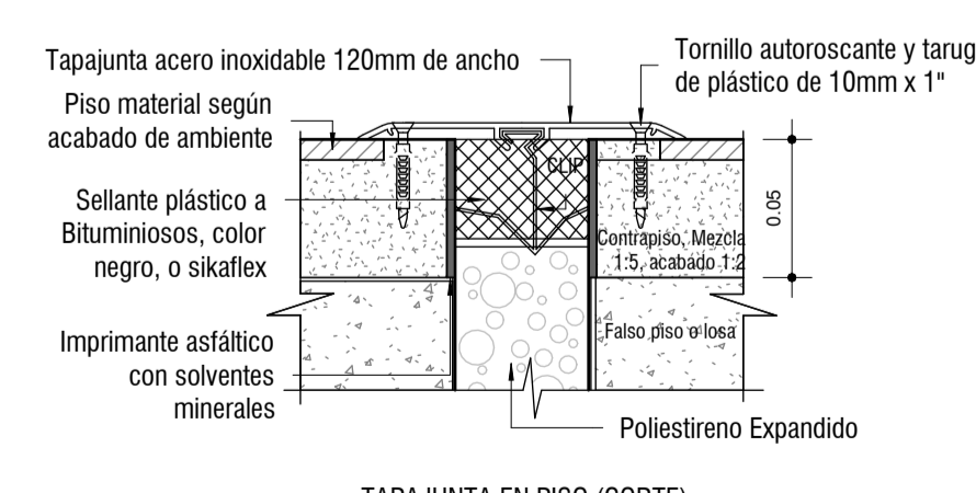
TAPAJUNTA EN PISO (CORTE) ESC: 5/8
