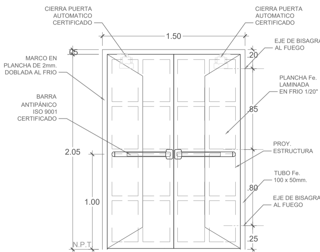
Pa-02 (1.50 x 2.10) ESC.:1/25
