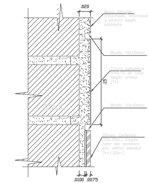
DET.10 ENCUENTRO DE ZÓCALO PORCELANATO CON MURO ACABADO Y BANDA SEÑALETICA (PARA MUROS) ESC: 1/2,5
