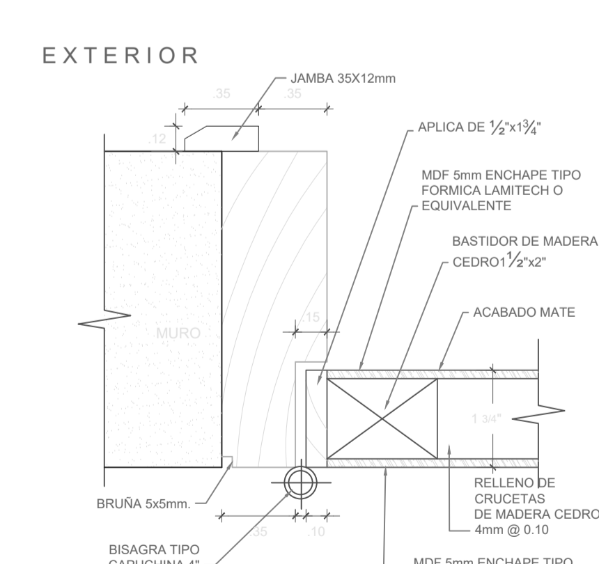
CORTE 02 ESC.:1/25
