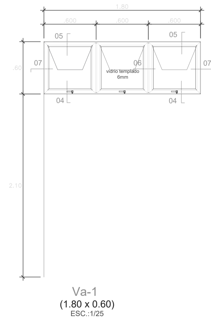
VENTANA DE ALUMINIO CON CRISTAL
