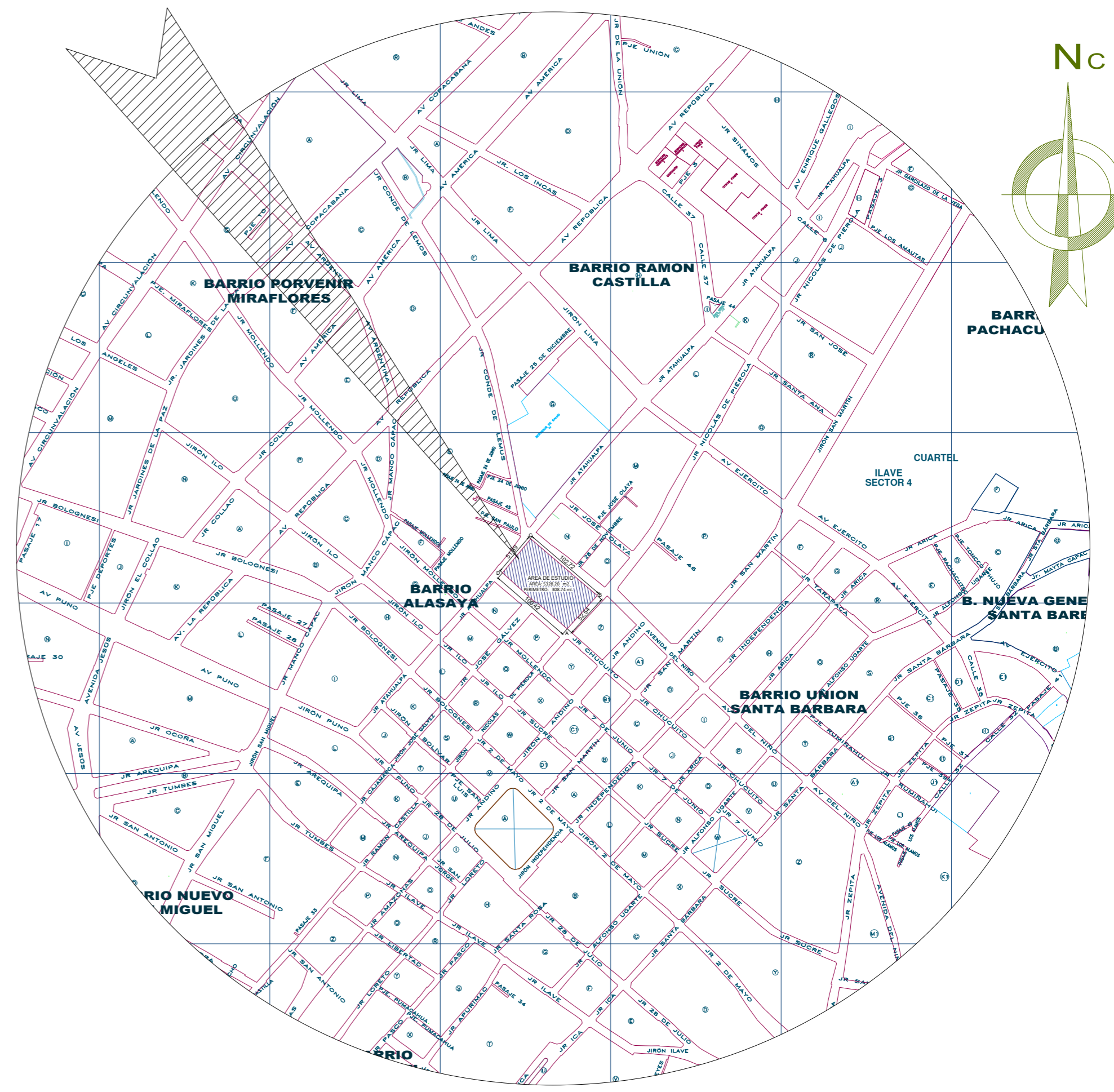
Plano de Ubicación ESC: 1 / 5000
