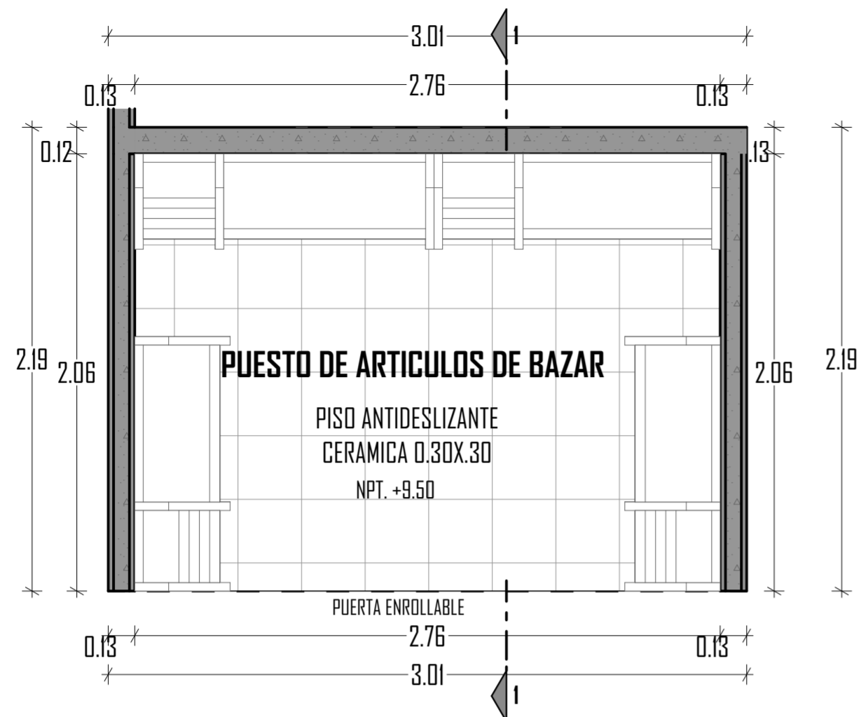
D-18 PUESTO DE ARTICULOS DE BAZAR Esc: 1:25
