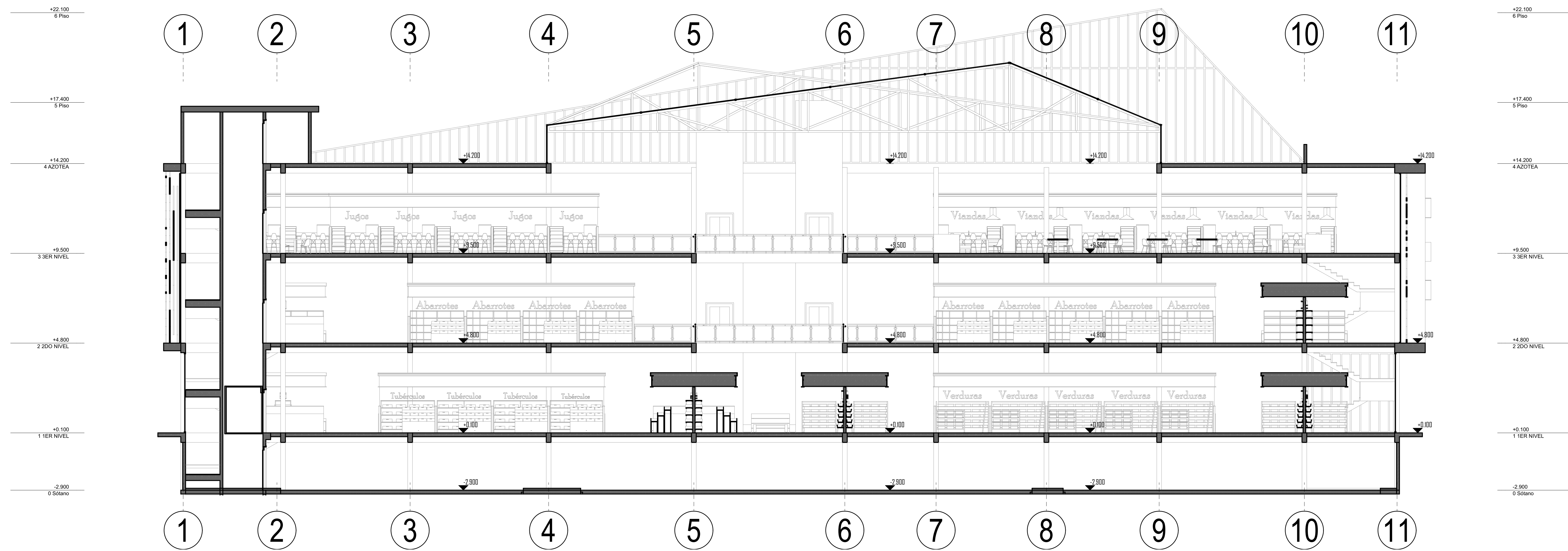
SECCION 1-1
