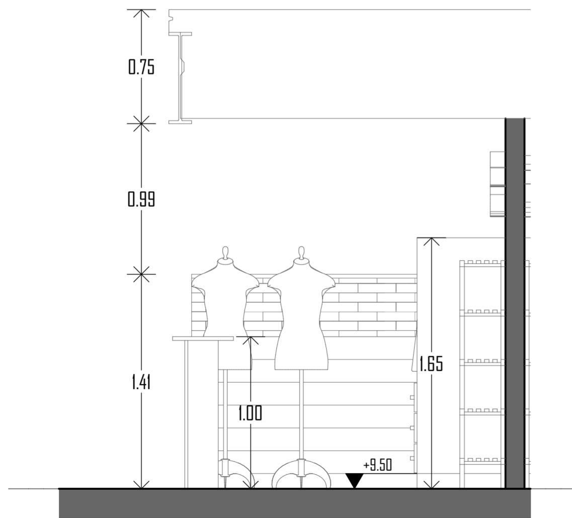
S14 SECCION 1-1 Esc: 1:25
