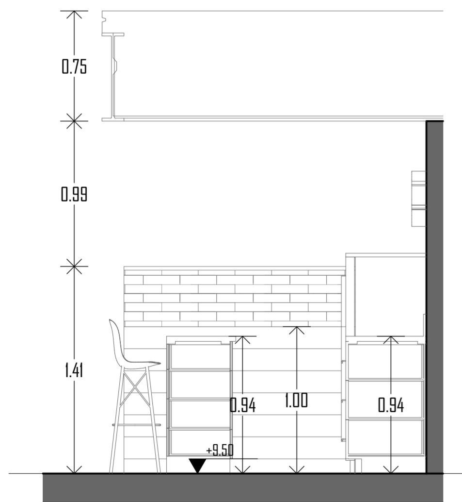
S12 SECCION 1-1 Esc: 1:25
