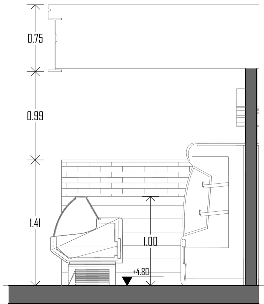
S8 SECCION 1-1 Esc: 1:25
