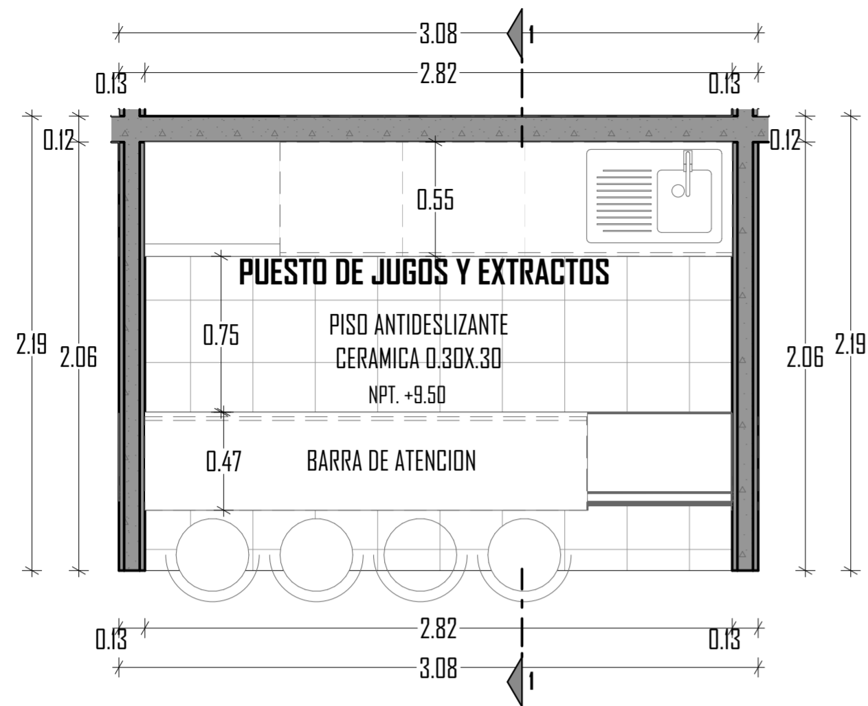
D-12 PUESTO DE JUGOS Y EXTRACTOS Esc: 1:25
