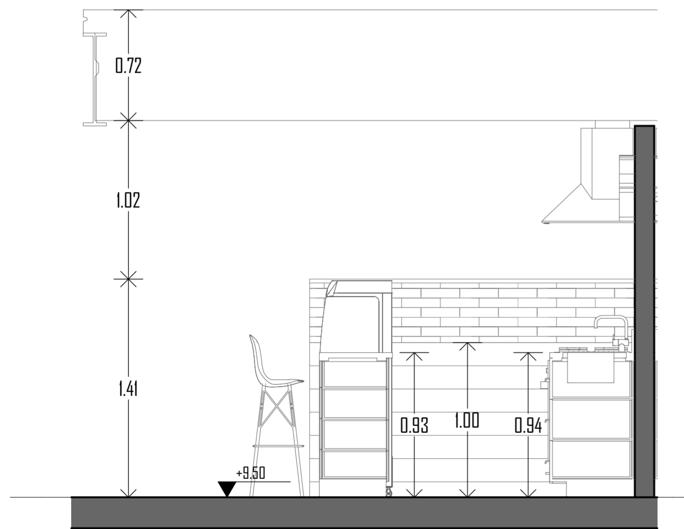
S11 SECCION 1-1 Esc: 1:25
