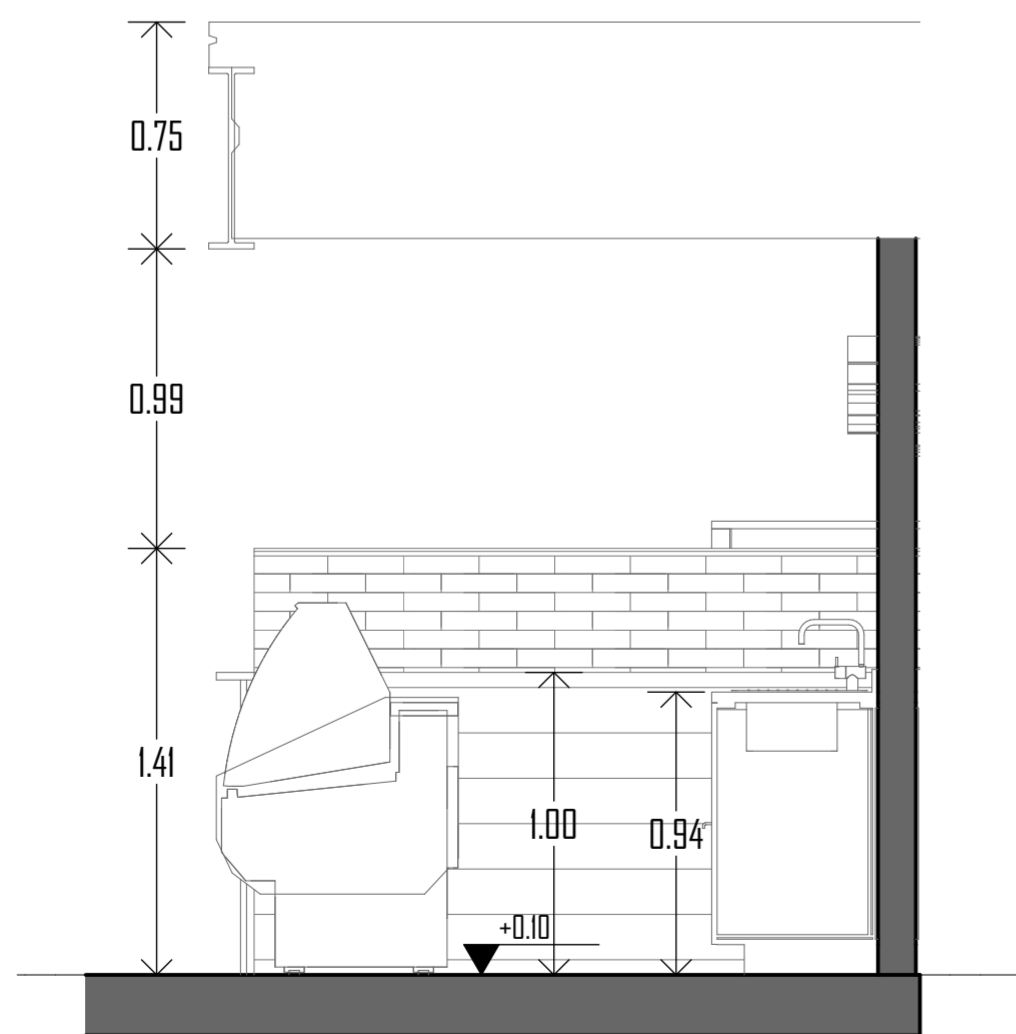
S2 SECCION 1-1 Esc: 1:25
