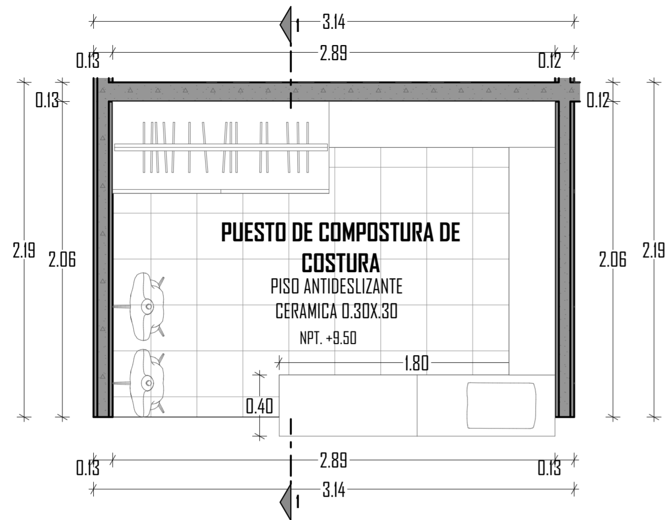
D-14 PUESTO DE COMPOSTURA DE COSTURA Esc: 1:25
