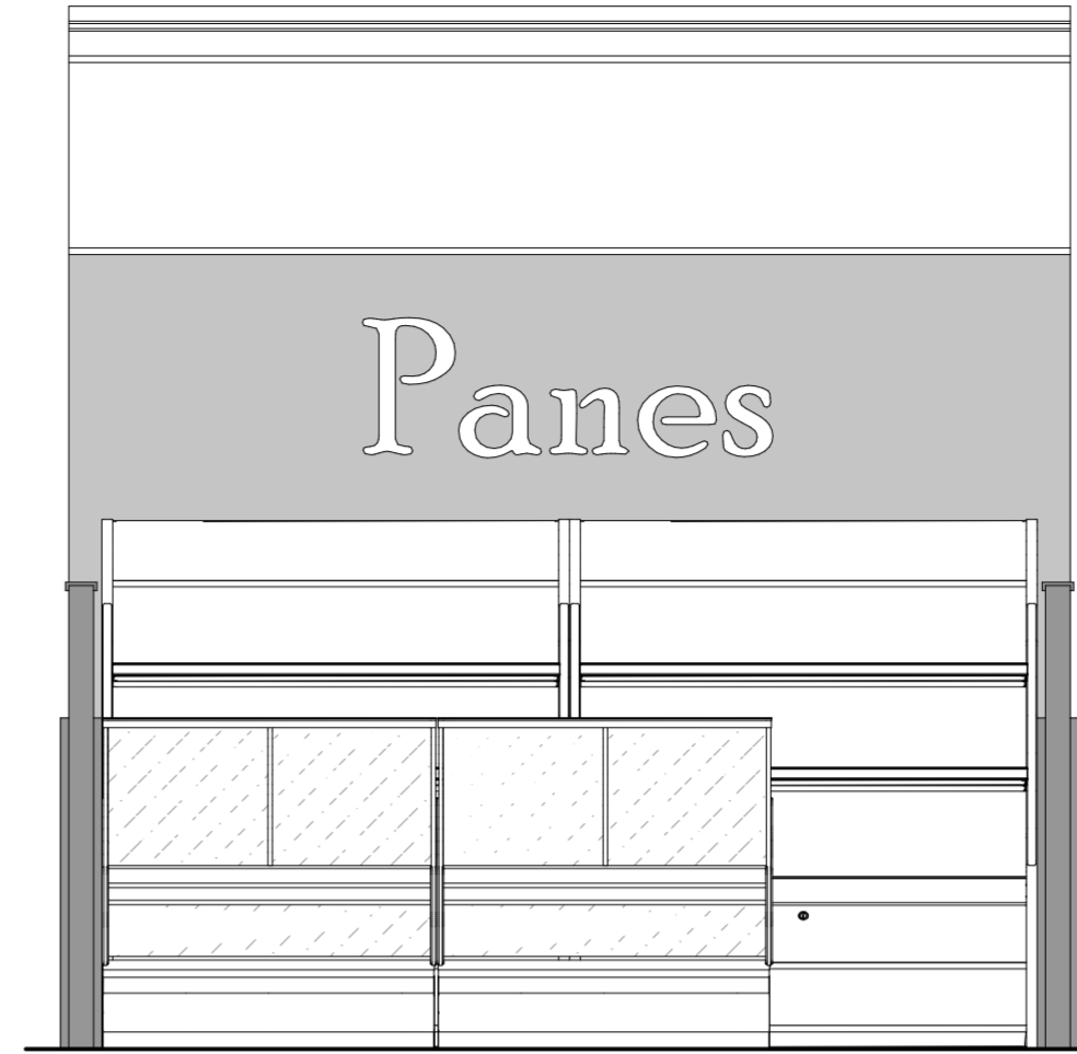
D-26 ELEVACIÓN Esc: 1:25
