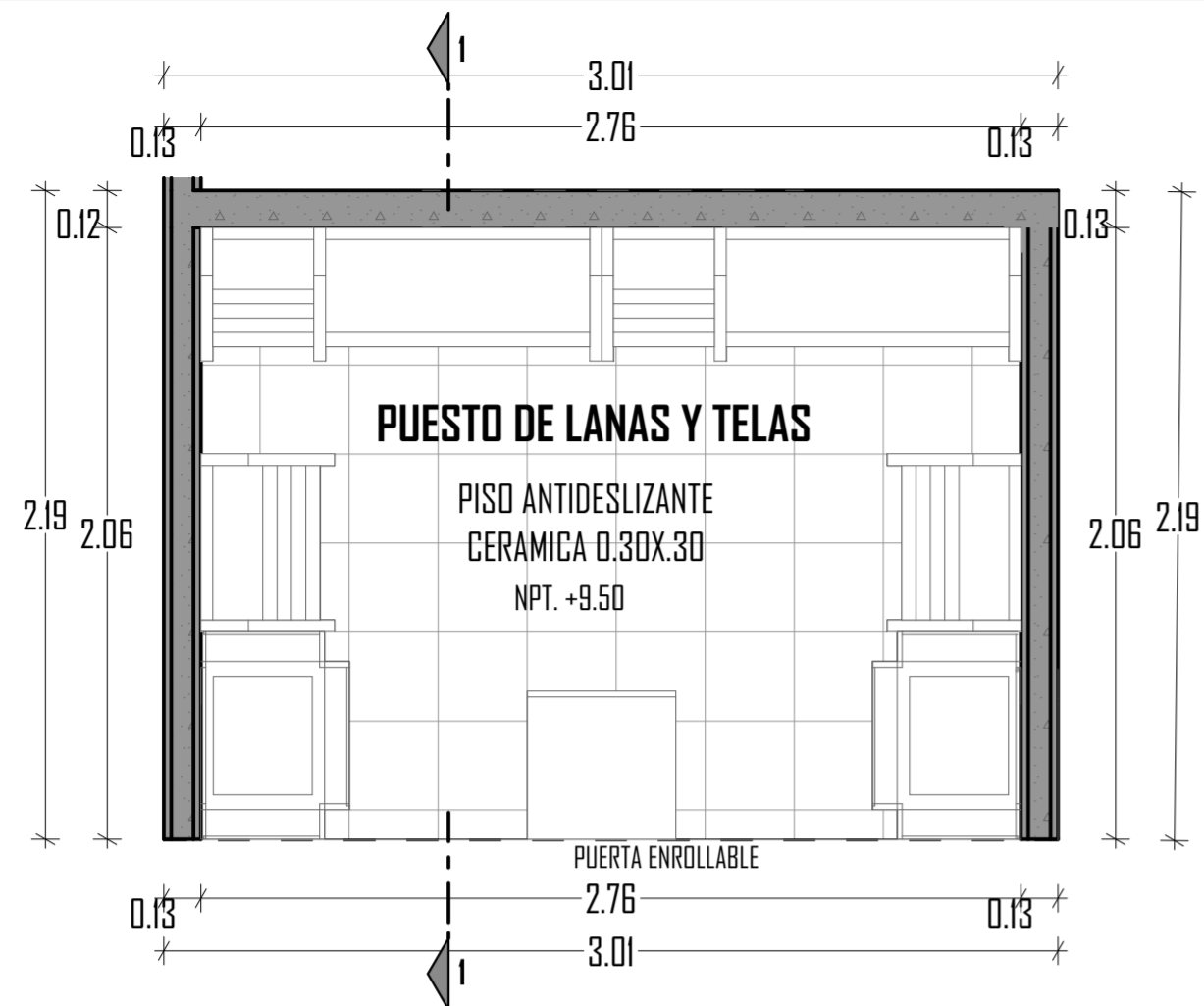
D-16 PUESTO DE LANAS Y TELAS Esc: 1:25
