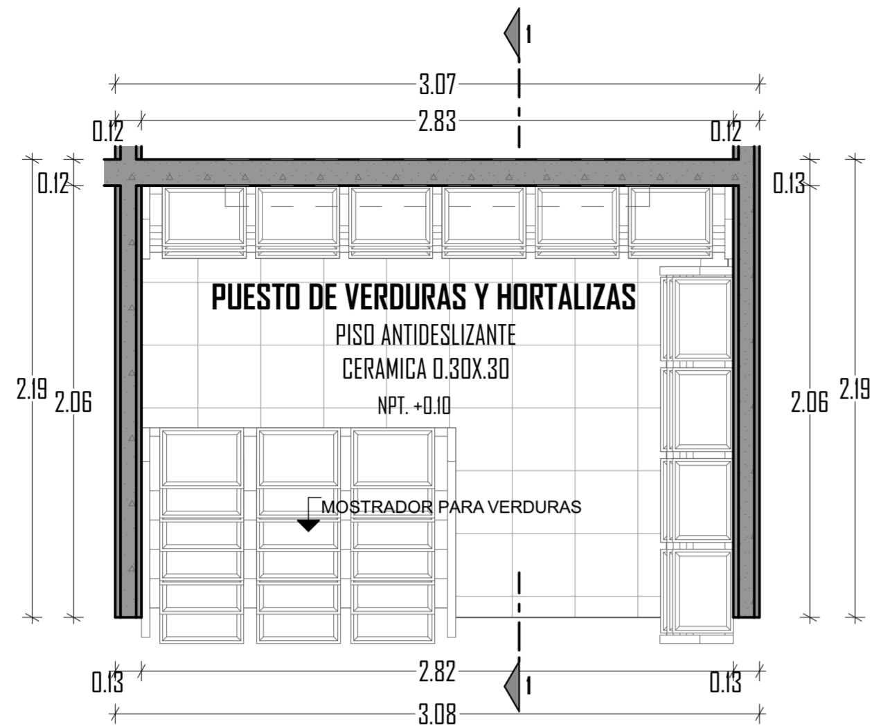
D-03 PUESTO DE VERDURAS Y HORTALIZAS Esc: 1:25
