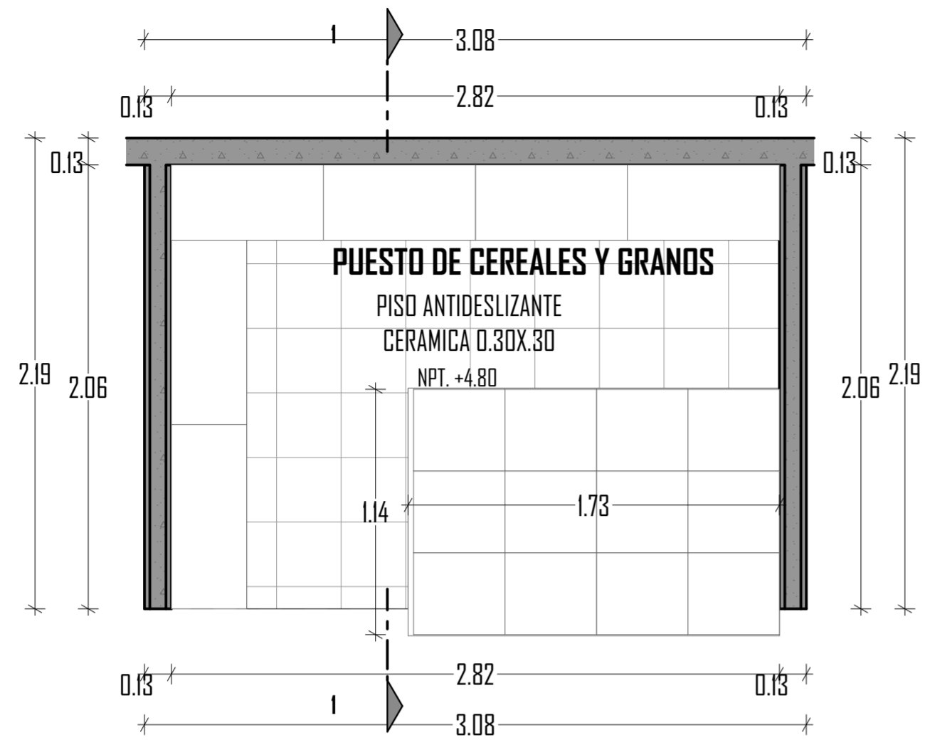
D-09 PUESTO DE CEREALES, GRANOS Esc: 1:25
