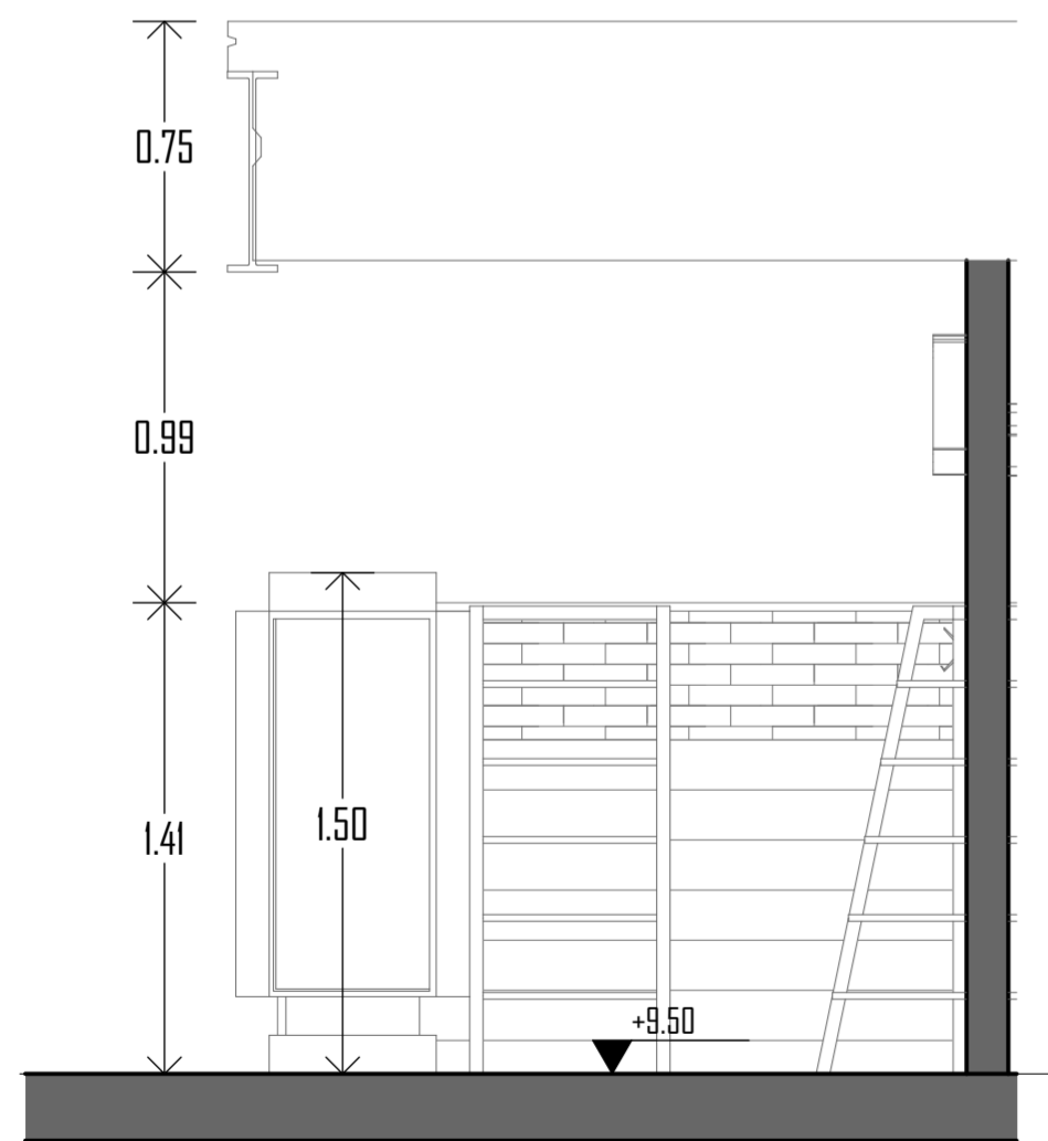
S16 SECCION 1-1 Esc: 1:25
