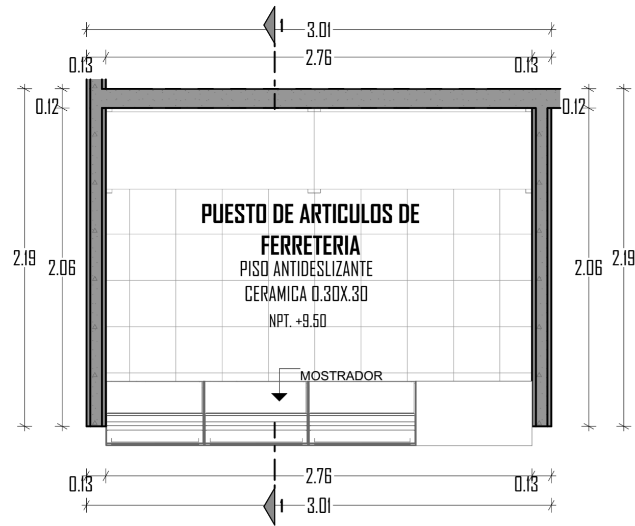
D-13 PUESTO DE ARTICULOS DE FERRETERIA Esc: 1:25
