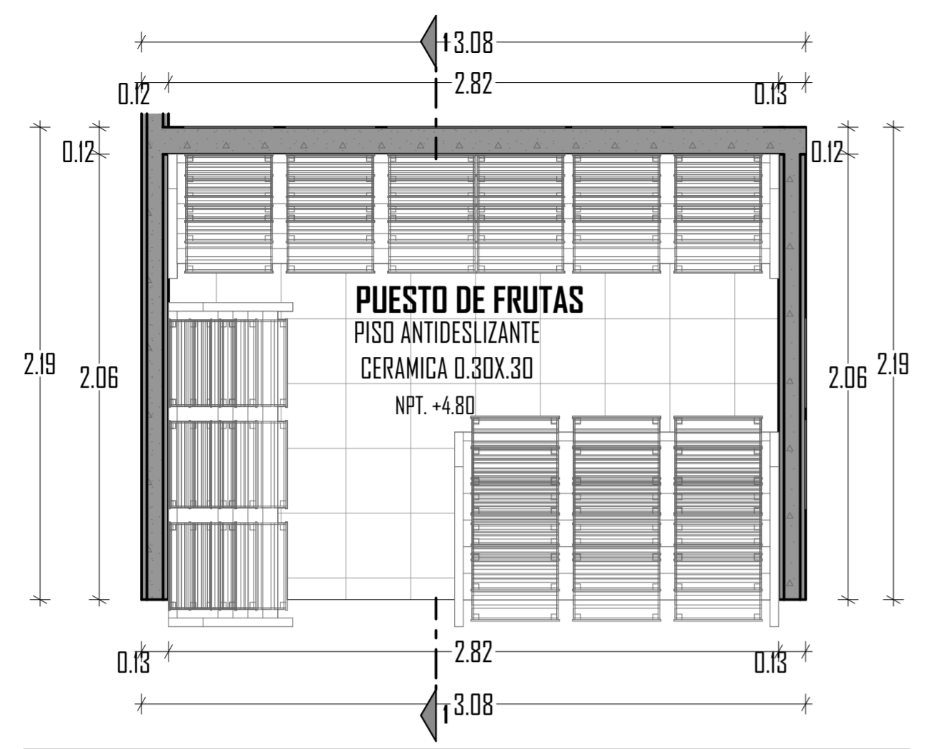
D-07 PUESTO DE FRUTAS Esc: 1:25
