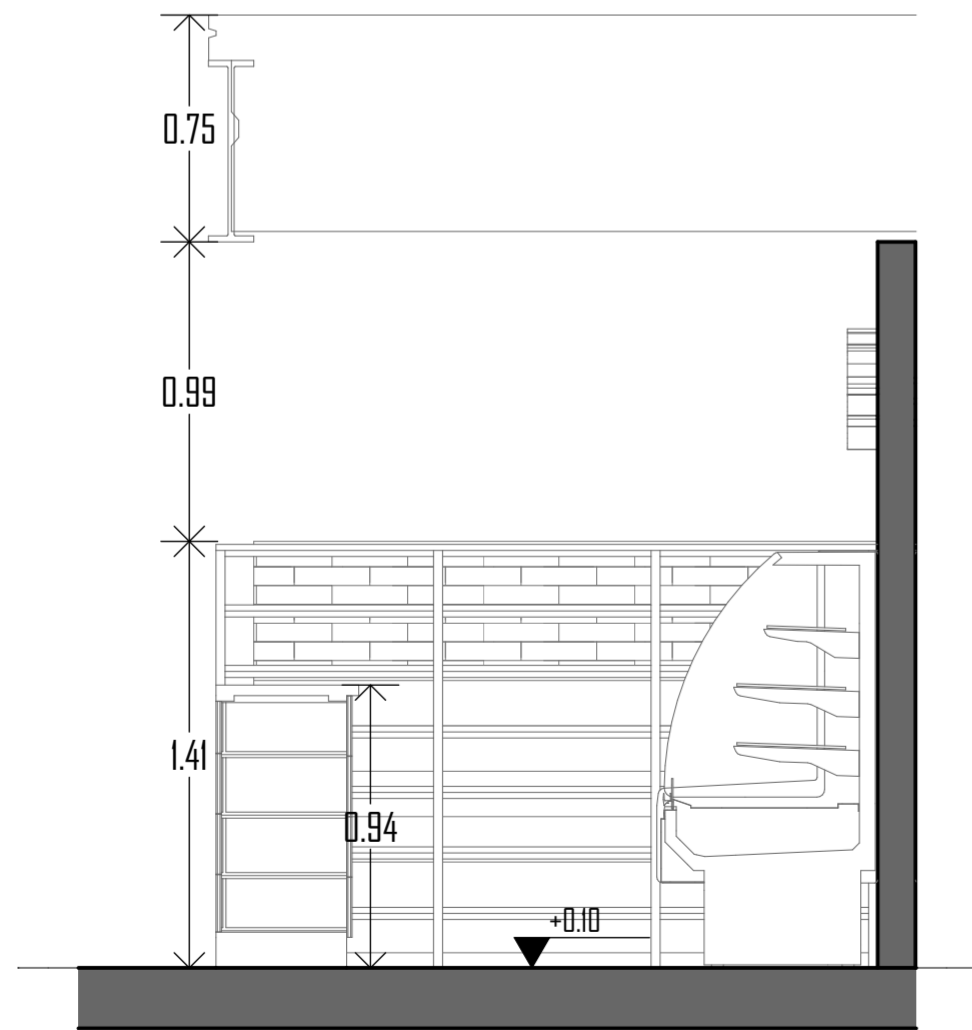
S5 SECCION 1-1 Esc: 1:25
