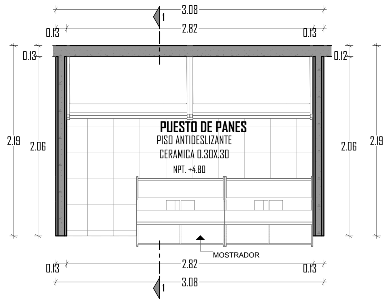
D-08 PUESTO DE PANES Esc: 1:25
