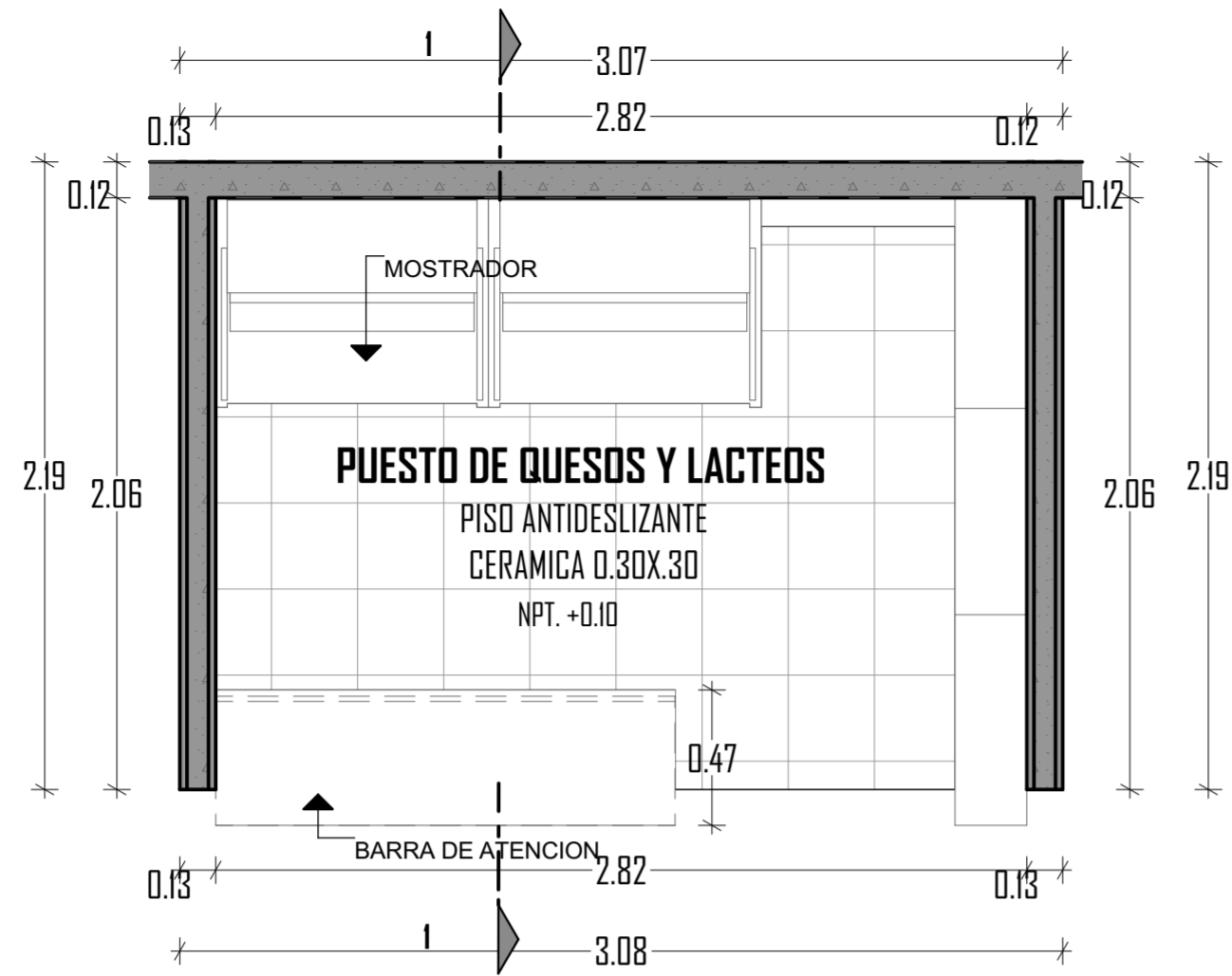
D-05 PUESTO DE QUESOS Y LÁCTEOS Esc: 1:25
