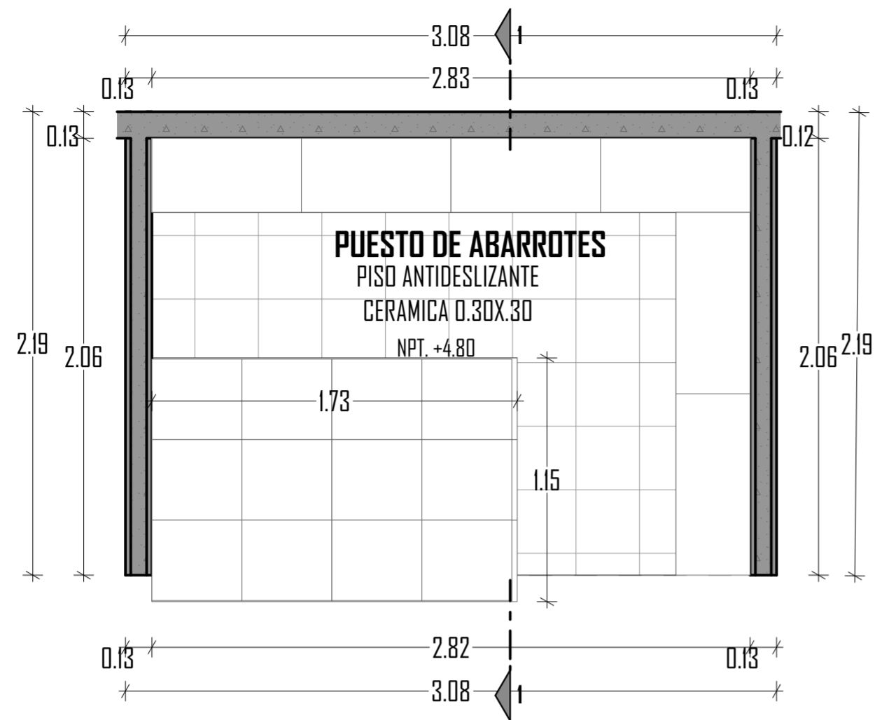
D-06 PUESTO DE ABARROTOS Esc: 1:25
