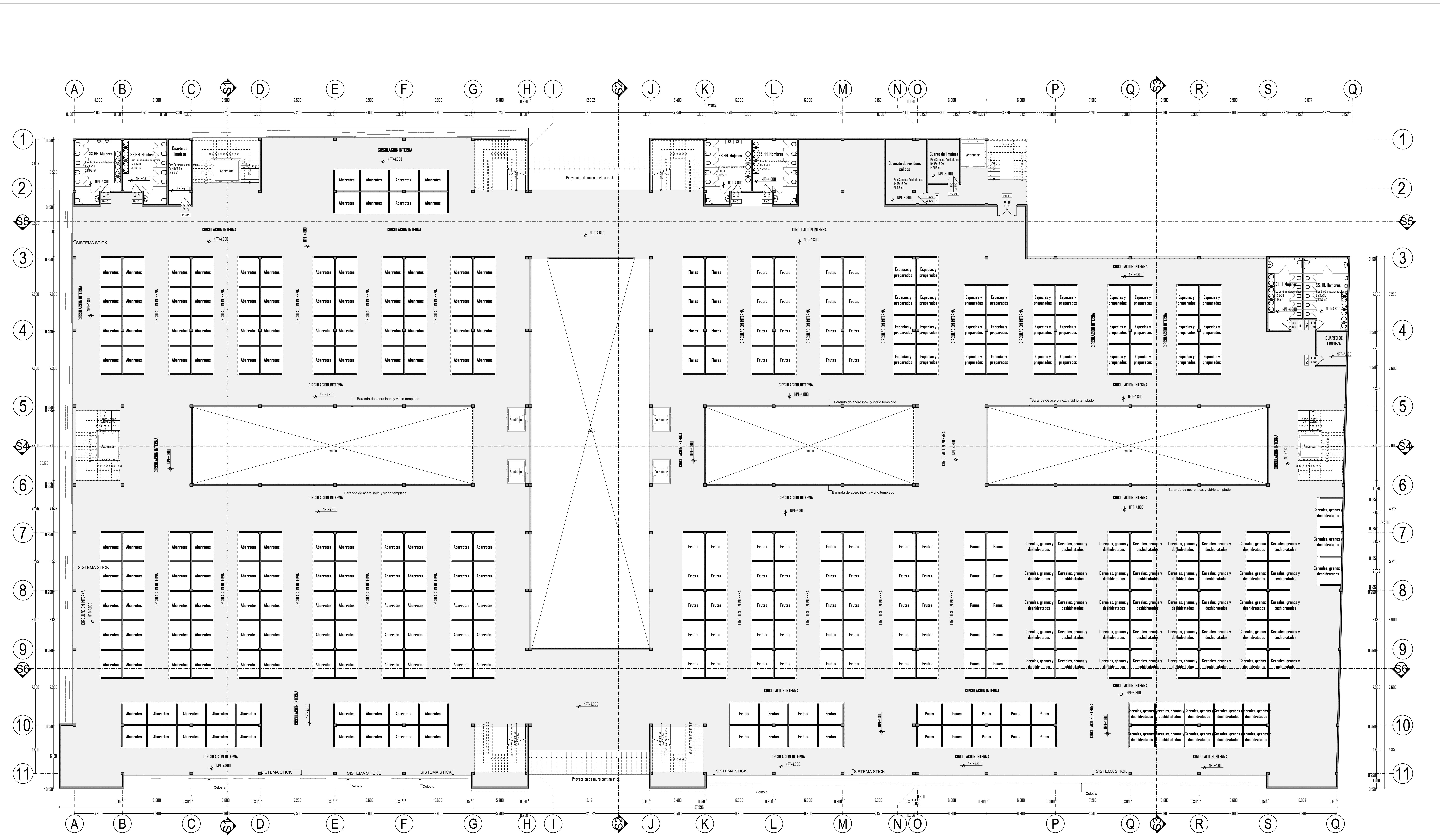
2. 2DO NIVEL
