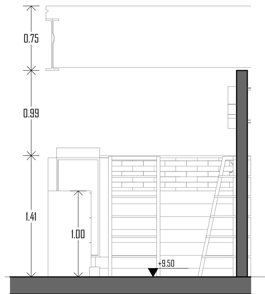
S17 SECCION 1-1 Esc: 1:25
