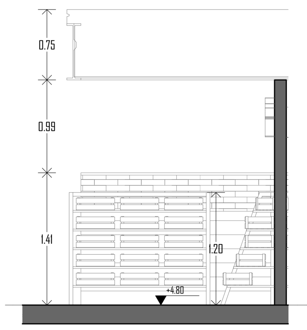
S7 SECCION 1-1 Esc: 1:25
