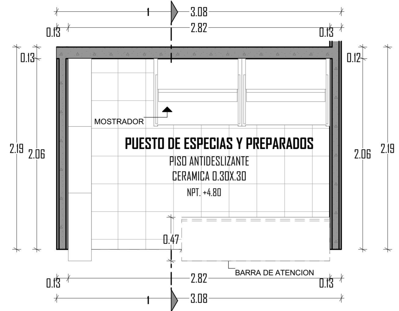
D-10 PUESTO DE ESPECIAS Y PREPARADOS Esc: 1:25
