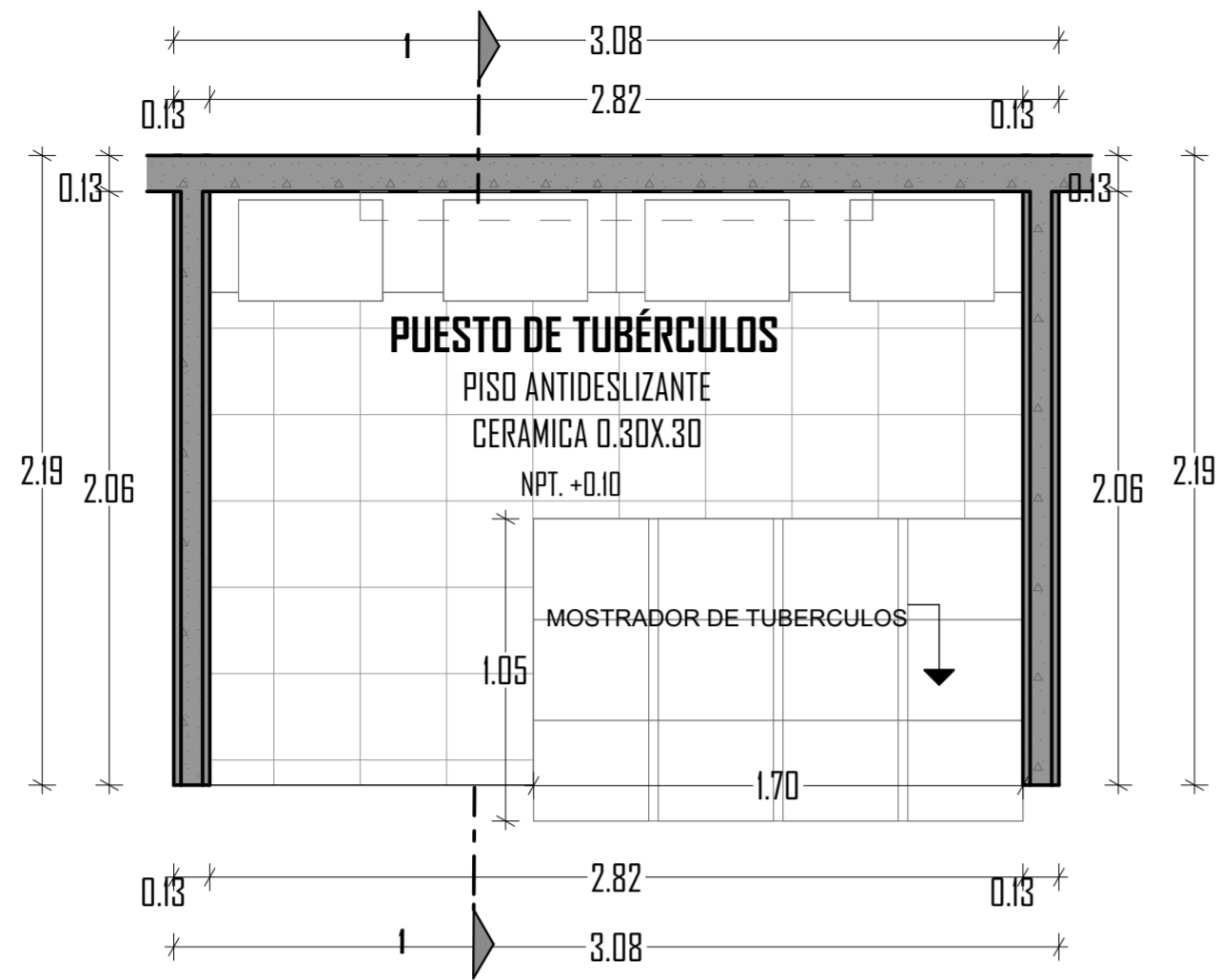
D-04 PUESTO DE TUBÉRCULOS Esc: 1:25
