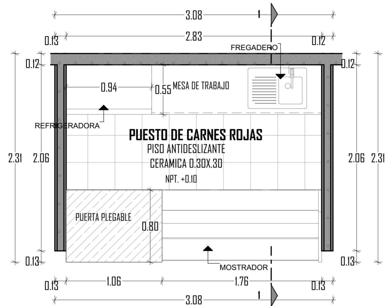
D-02 PUESTO DE CARNES ROJAS Esc: 1:25
