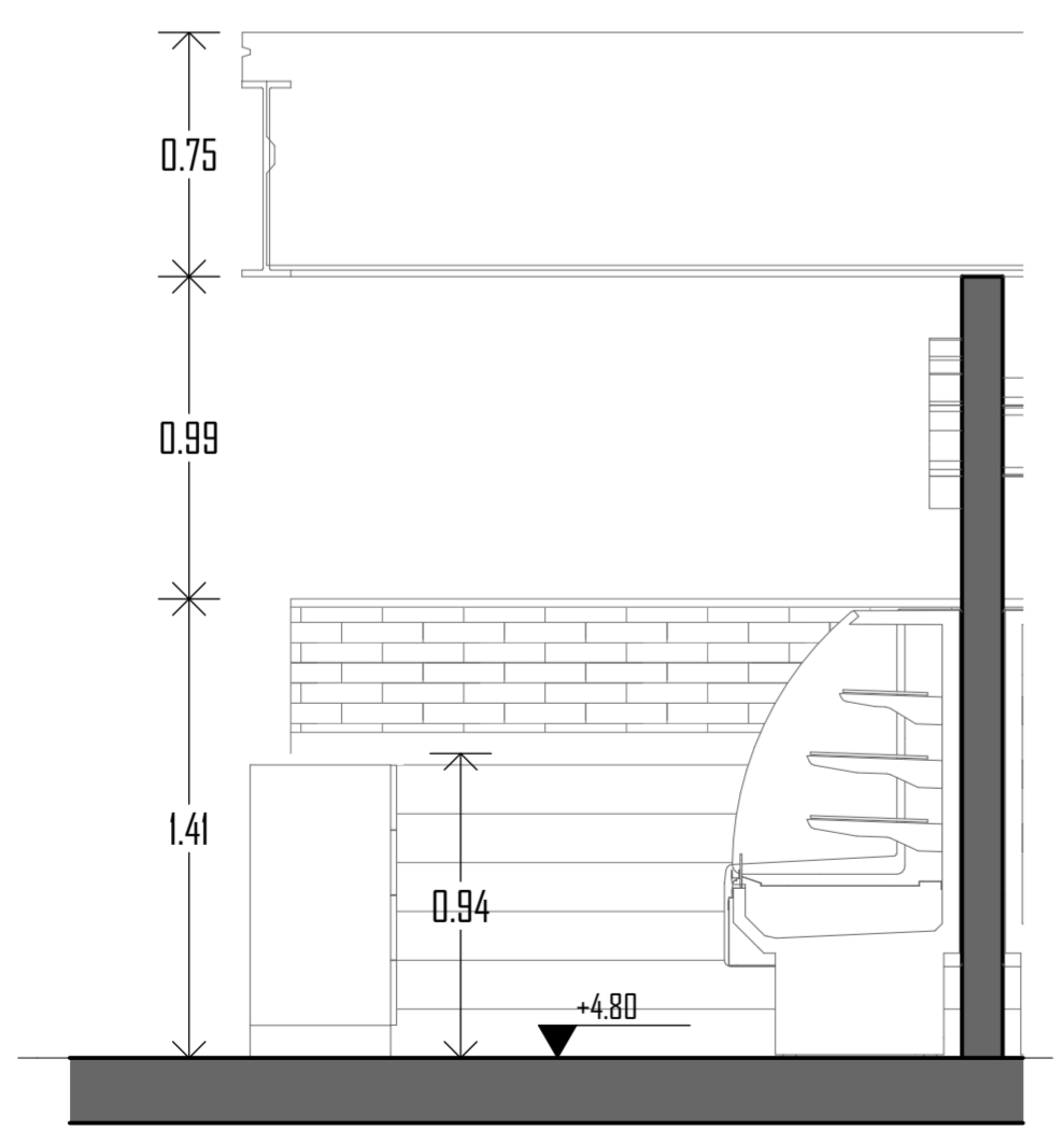
S10 SECCION 1-1 Esc: 1:25
