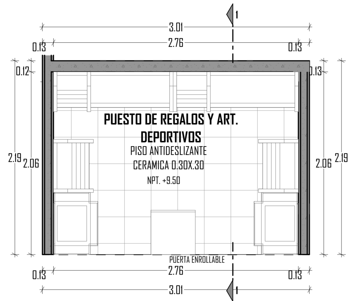
D-17 PUESTO DE REGALOS Y ART. DEPORTIVOS Esc: 1:25
