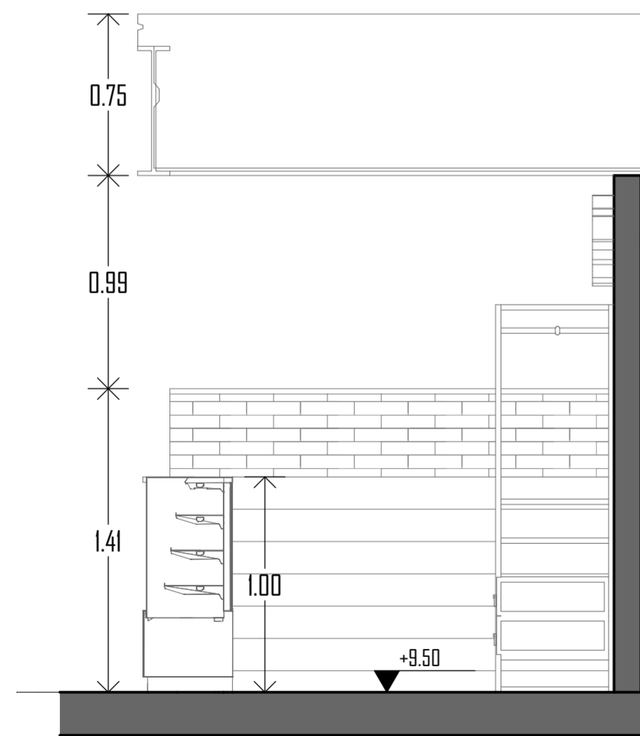
S13 SECCION 1-1 Esc: 1:25
