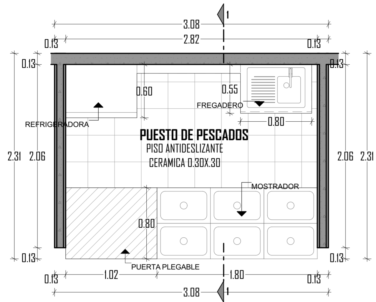
D-01 PUESTO DE PESCADOS Esc: 1:25
