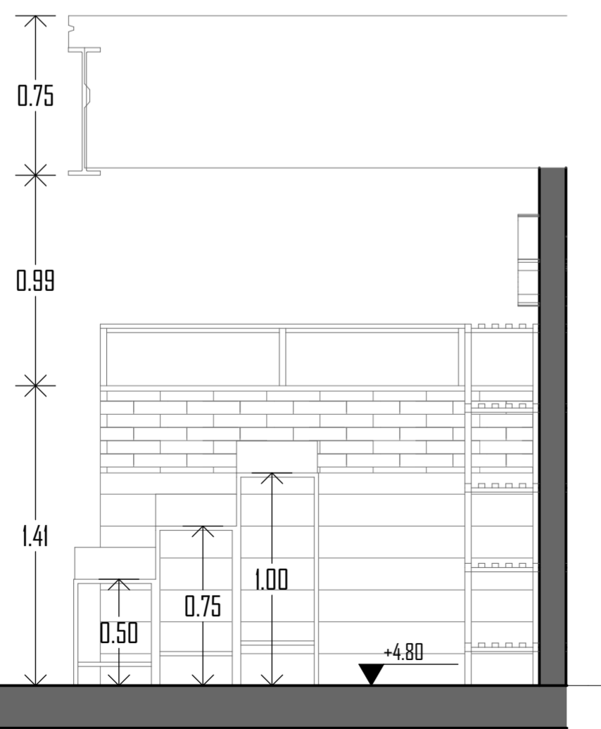
S6 SECCION 1-1 Esc: 1:25
