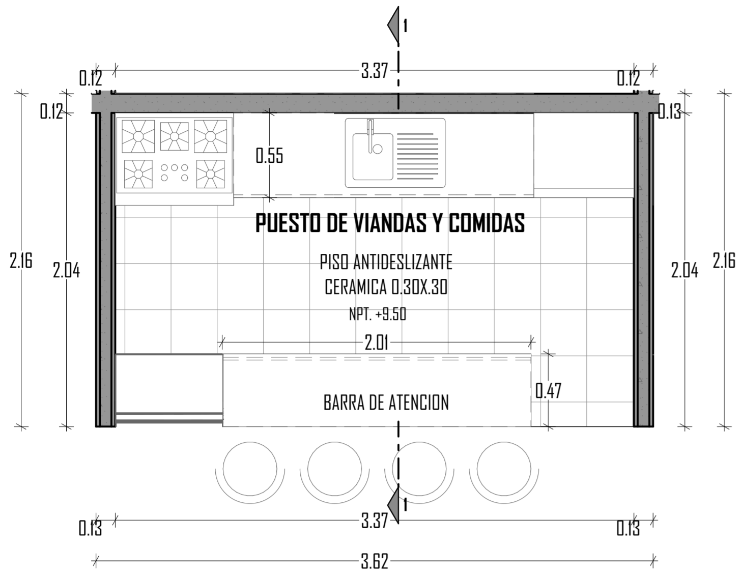
D-11 PUESTO DE VIANDAS Y COMIDAS Esc: 1:25
