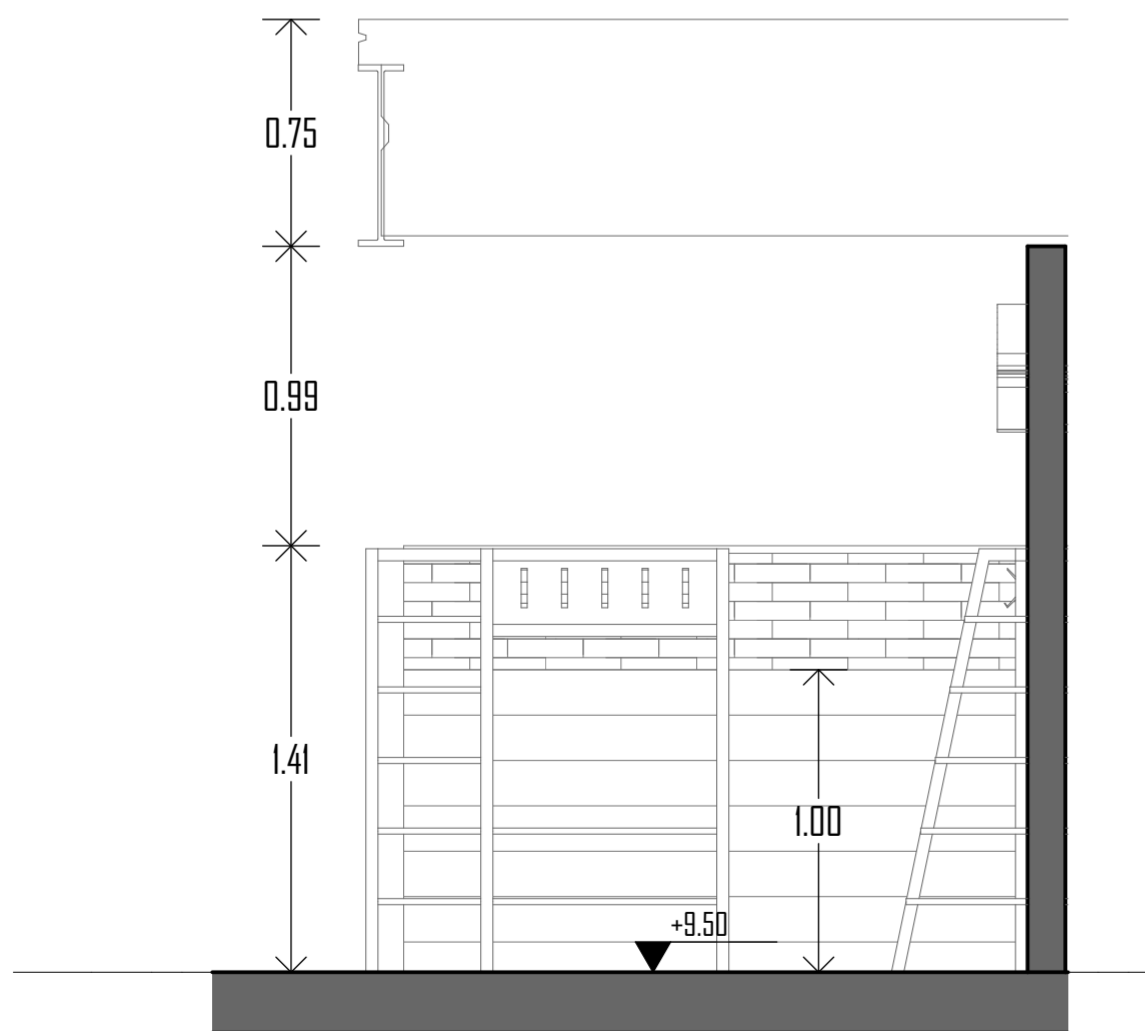
S18 SECCION 1-1 Esc: 1:25
