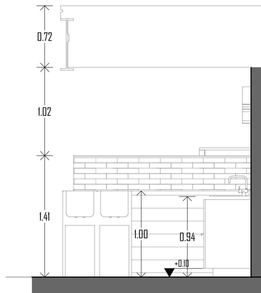
S1 SECCION 1-1 Esc: 1:25
