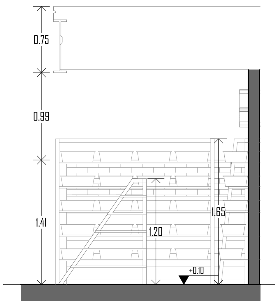
S3 SECCION 1-1 Esc: 1:25
