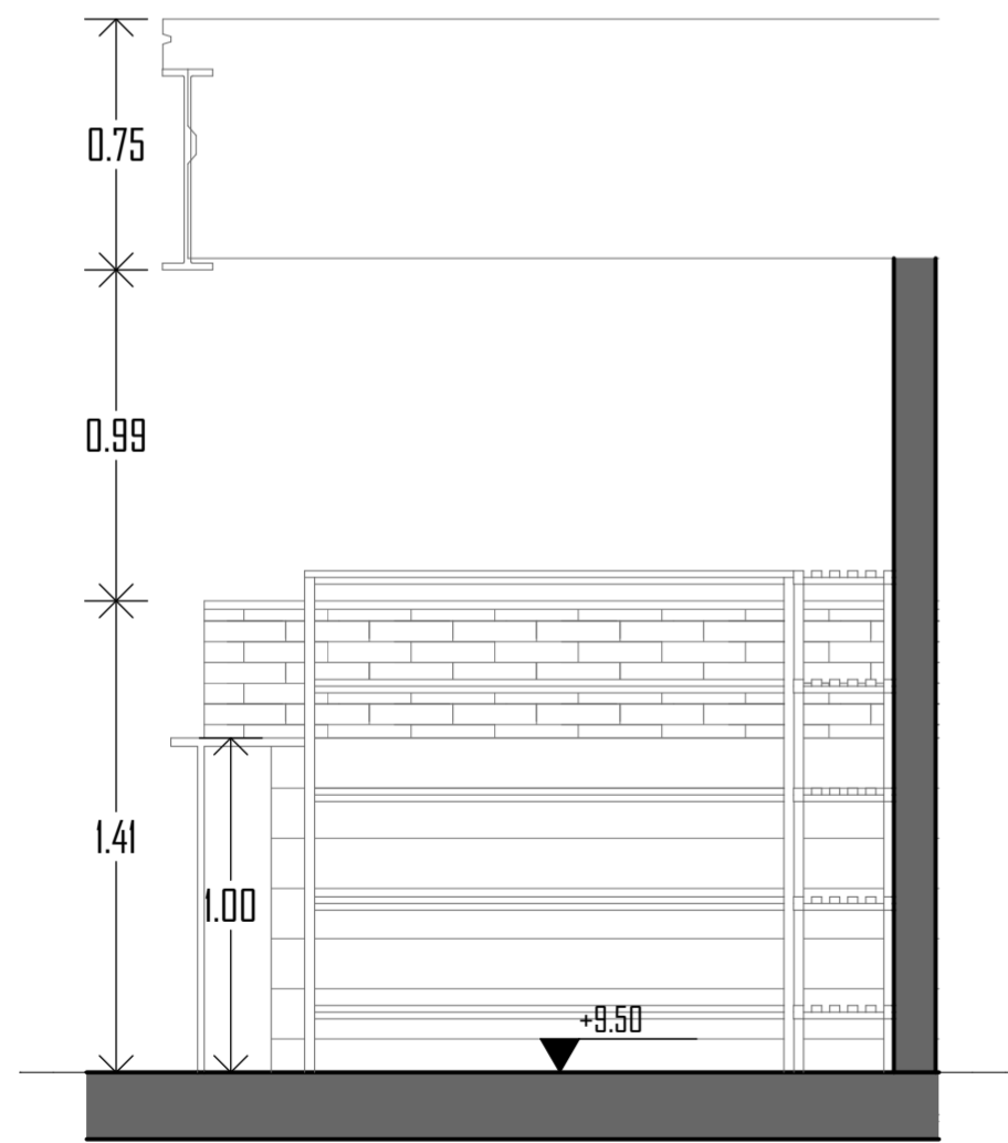
S15 SECCION 1-1 Esc: 1:25
