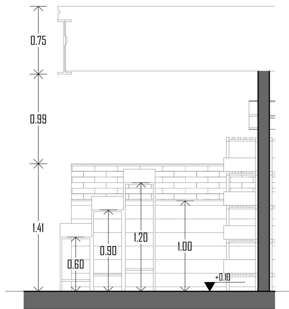
S4 SECCION 1-1 Esc: 1:25
