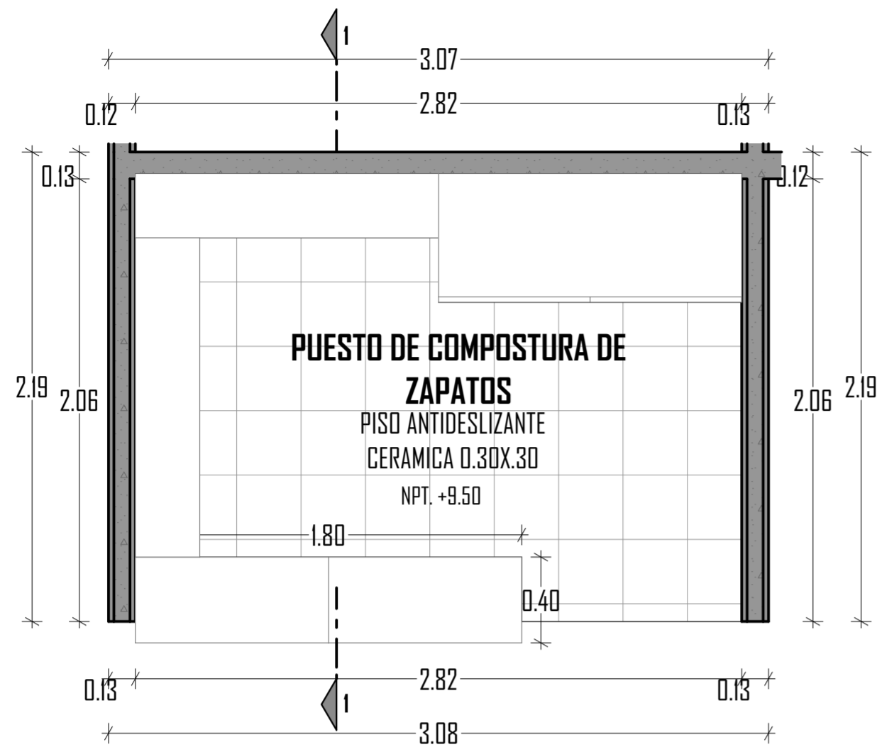
D-15 PUESTO DE COMPOSTURA DE ZAPATOS Esc: 1:25
