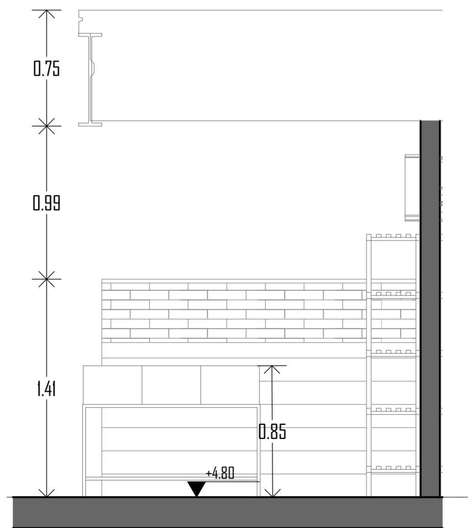
S9 SECCION 1-1 Esc: 1:25
