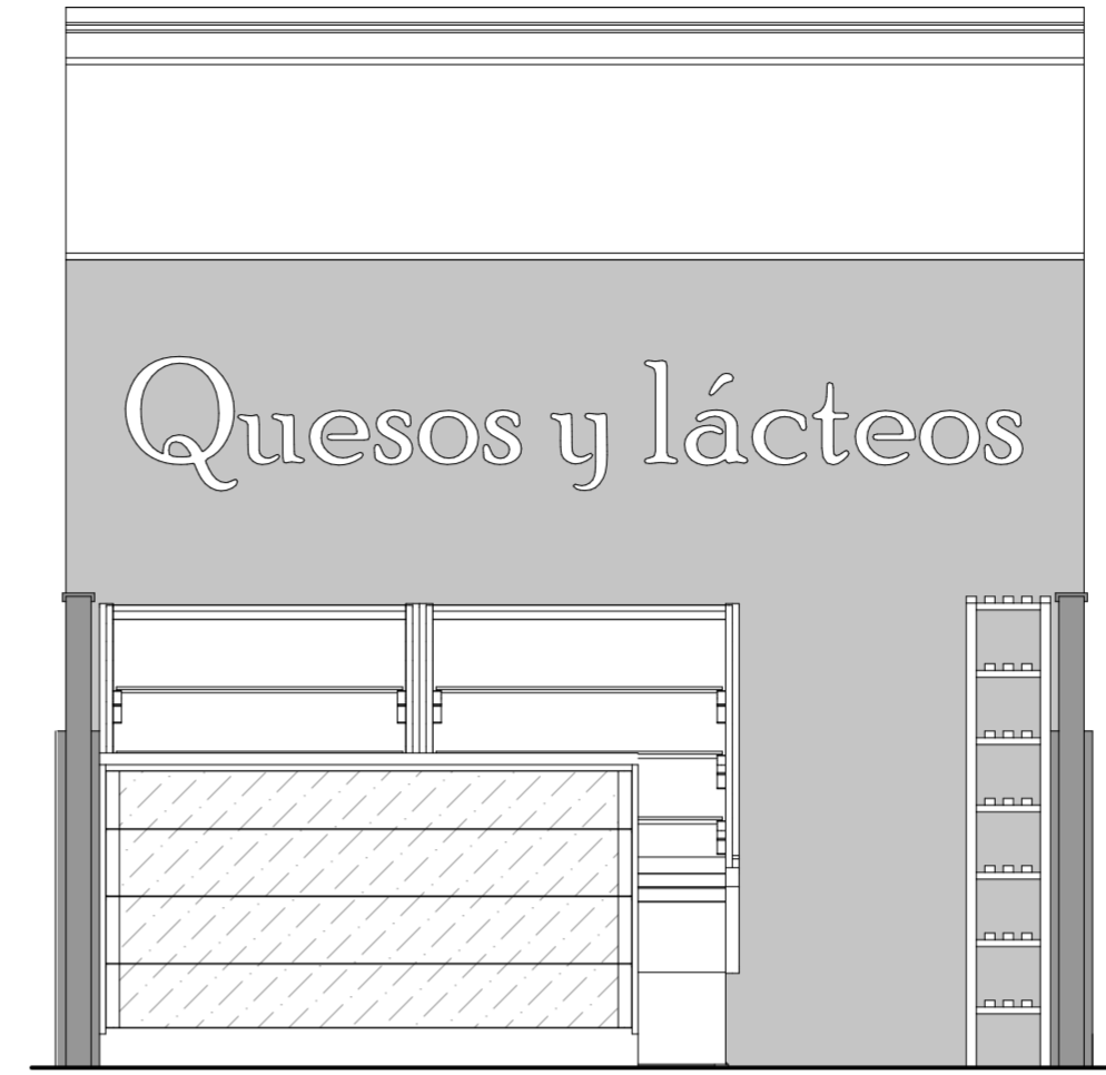
D-23 ELEVACIÓN Esc: 1:25
