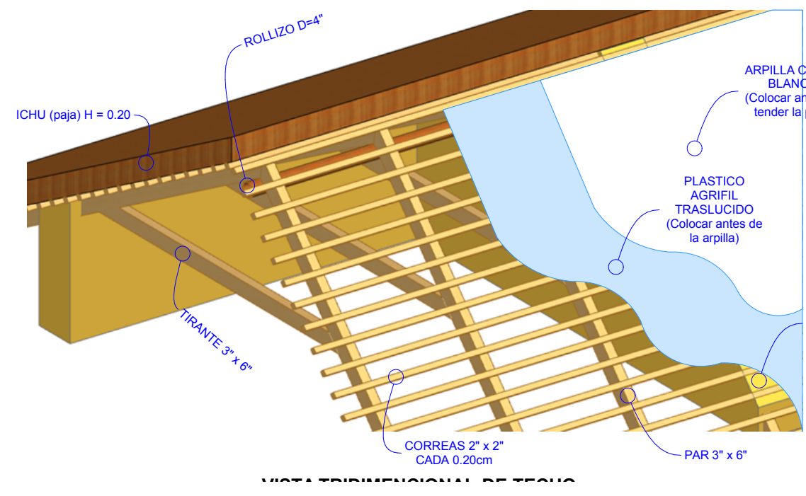
DETALLE DE LA ESTRUCTURA DE LA CUBIERTA
