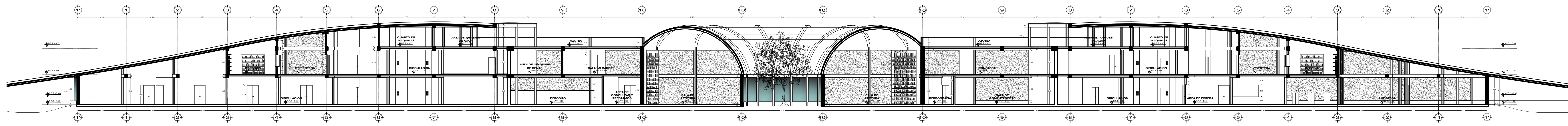
SECCION A - A ESC: 1/200
