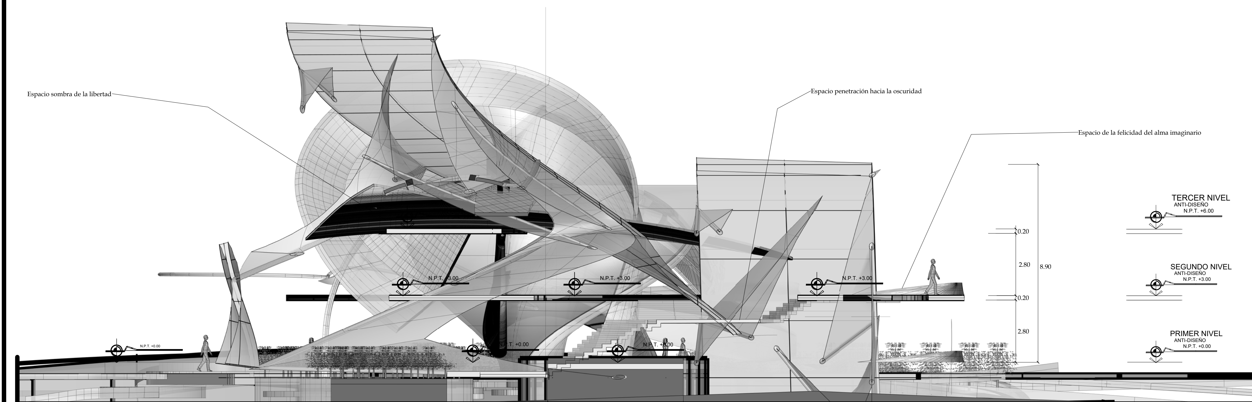
CORTE B-B'
