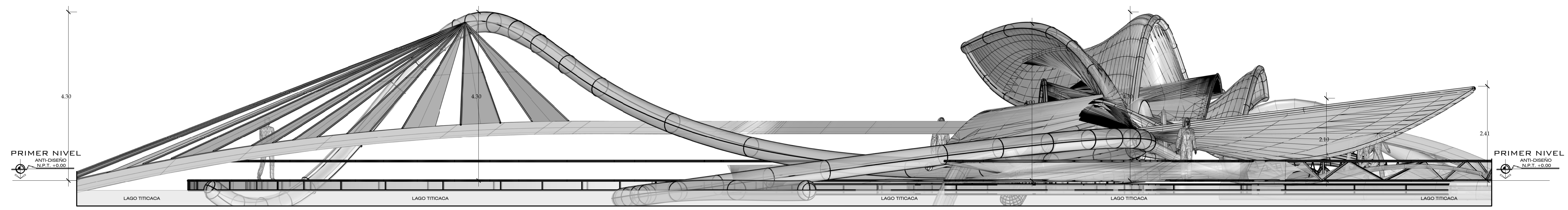
ELEVACION SUR ESC: 1/50
