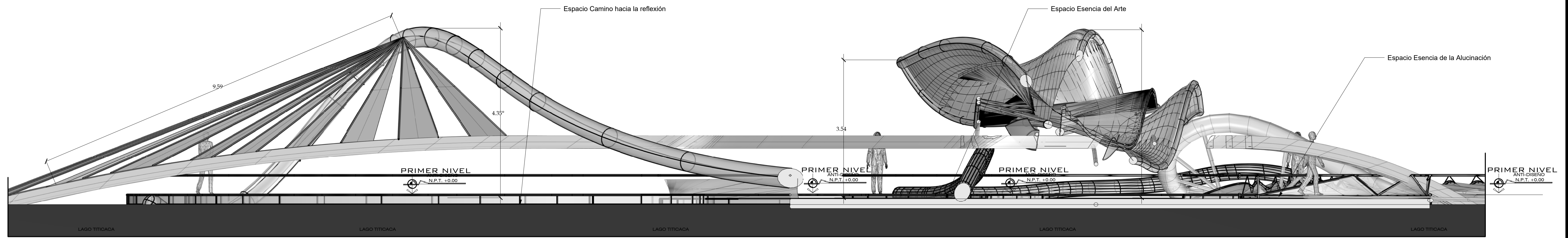
CORTE X-X ESC: 1/50
