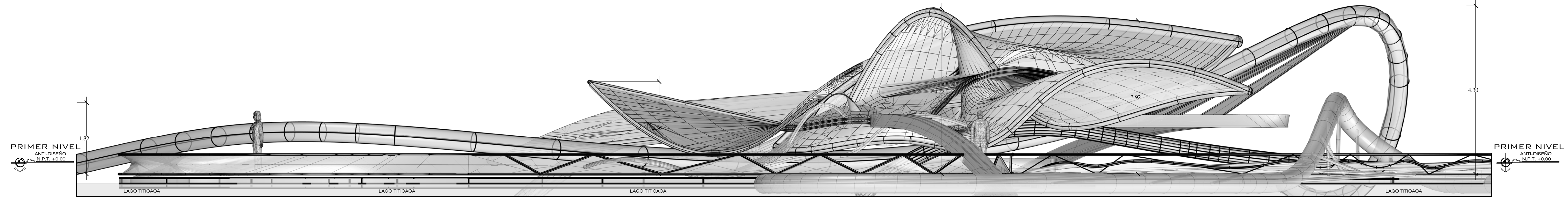
ELEVACION ESTE ESC: 1/50
