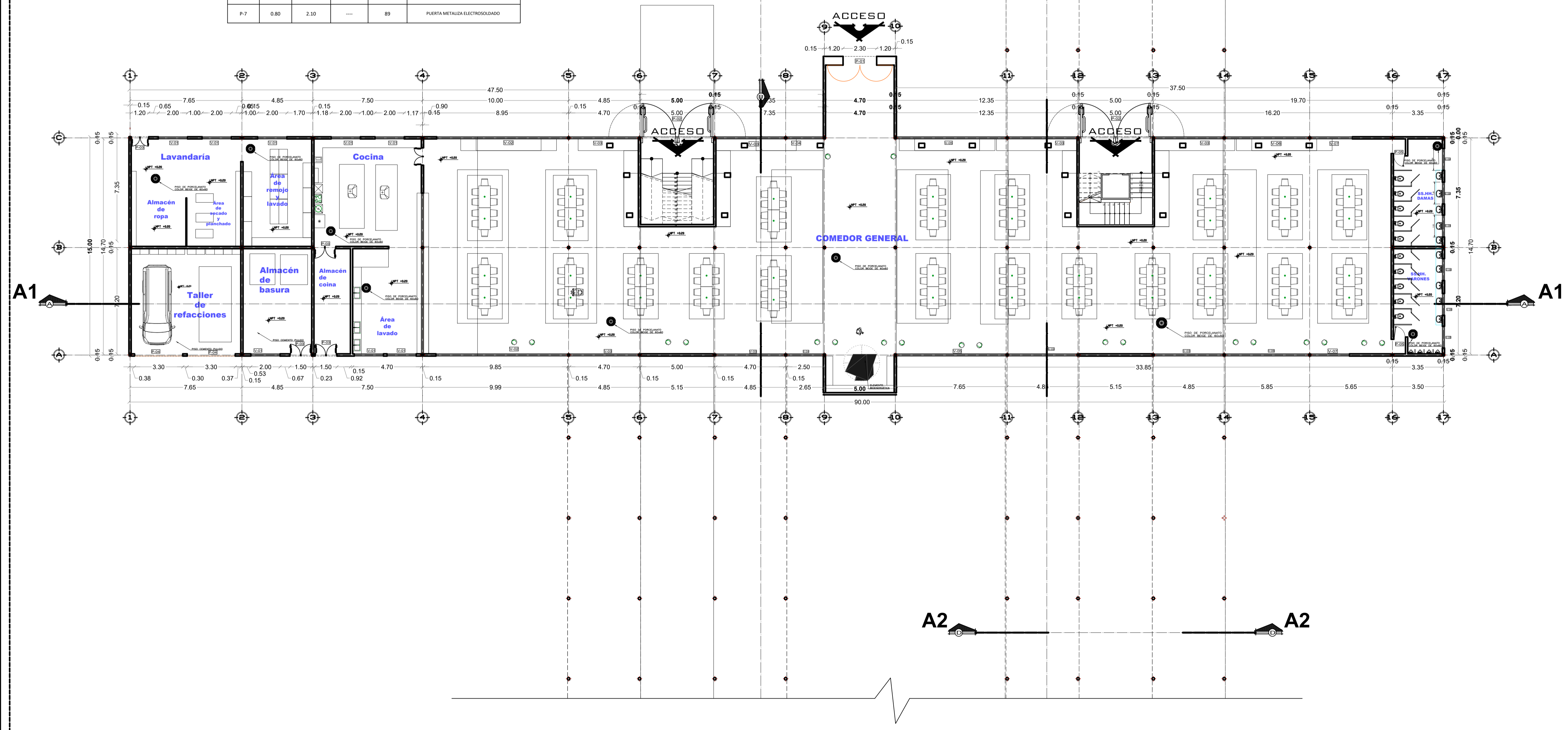
PRIMERA PLANTA - COMEDOR Y ACCESOS A RESIDENCIAS Esc : 1 / 150
