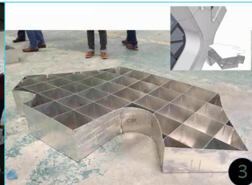
● ENSAMBLE DE PIEZAS PARA LOS NODOS ESTRUCTURALES
