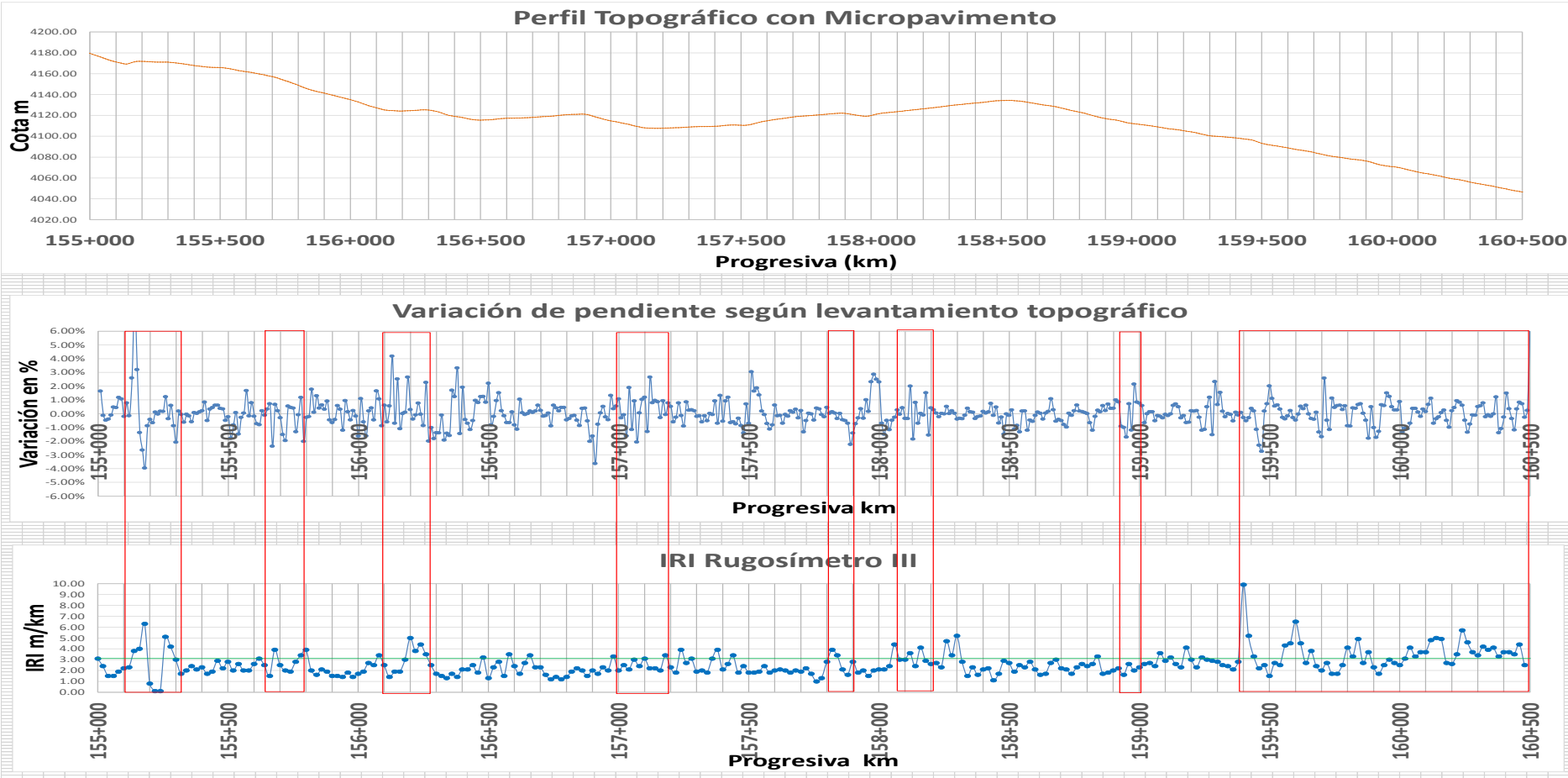
Comparación de perfil topográfico, variación de la pendiente e IRI en el sector Km 155+000-Km160+500
