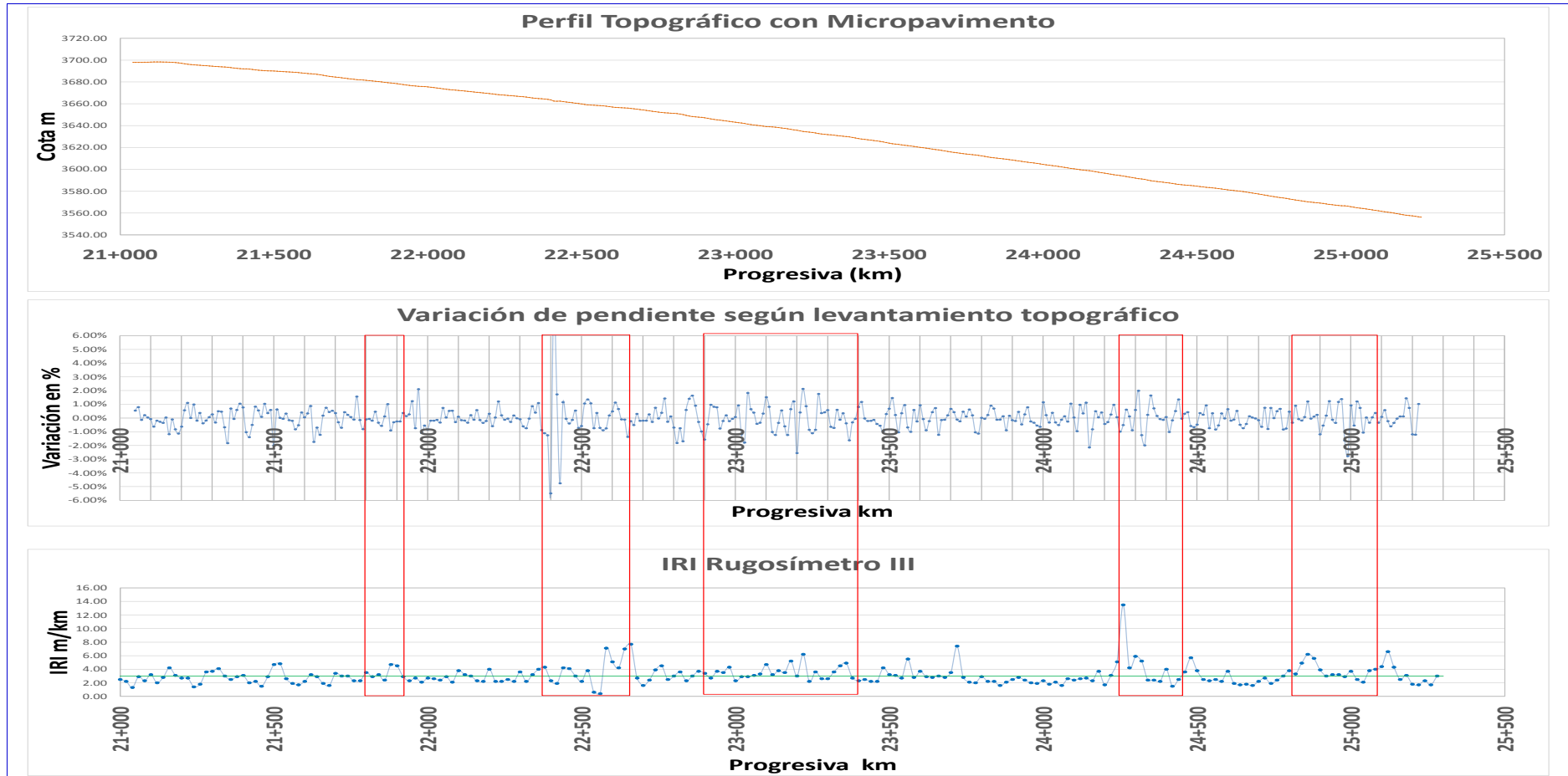
Comparación de perfil topográfico, variación de la pendiente e IRI en el sector Km 21+040- Km 25+228
