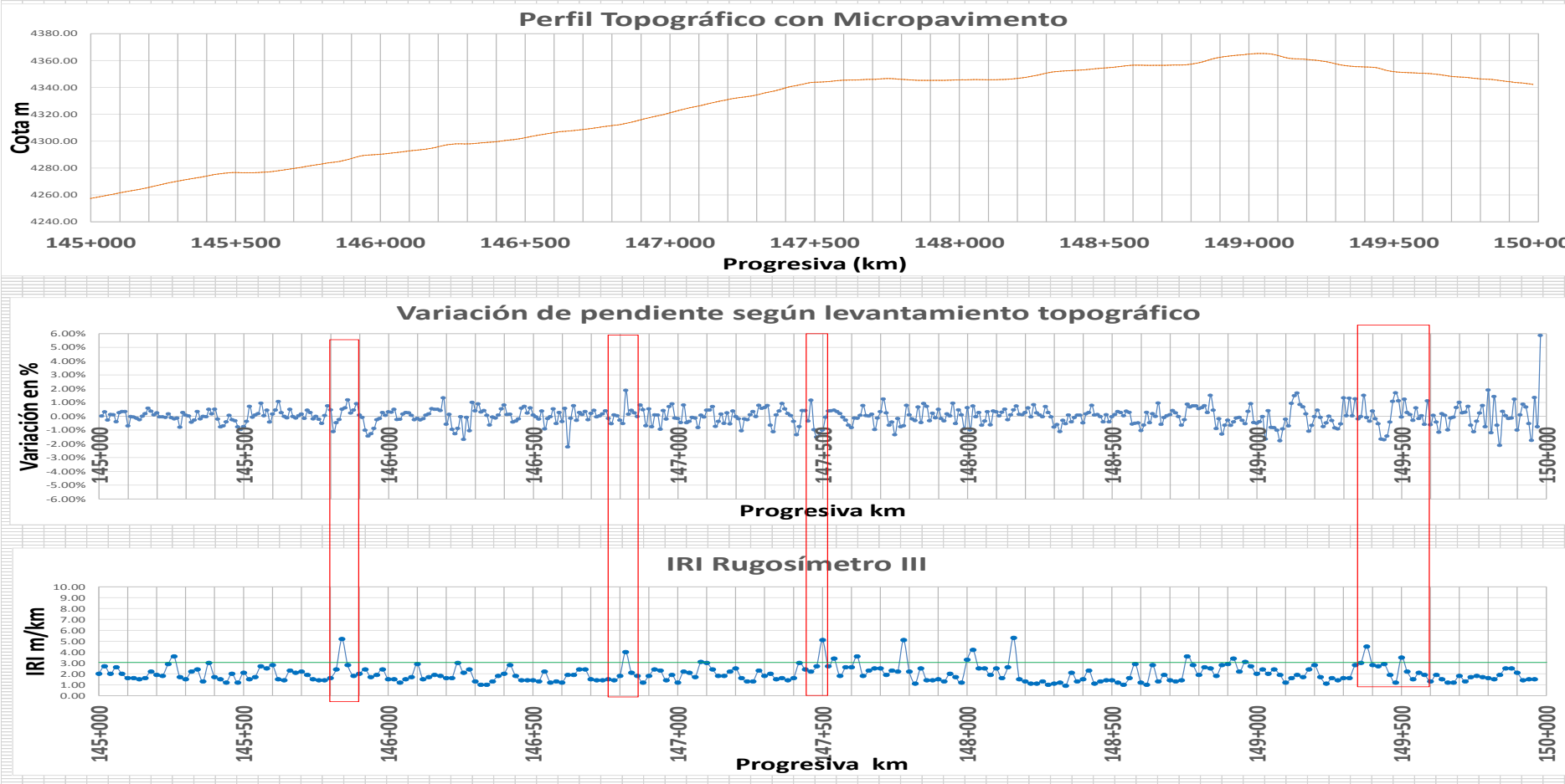
Comparación de perfil topográfico, variación de la pendiente e IRI en el sector Km 145+000-Km149+980
