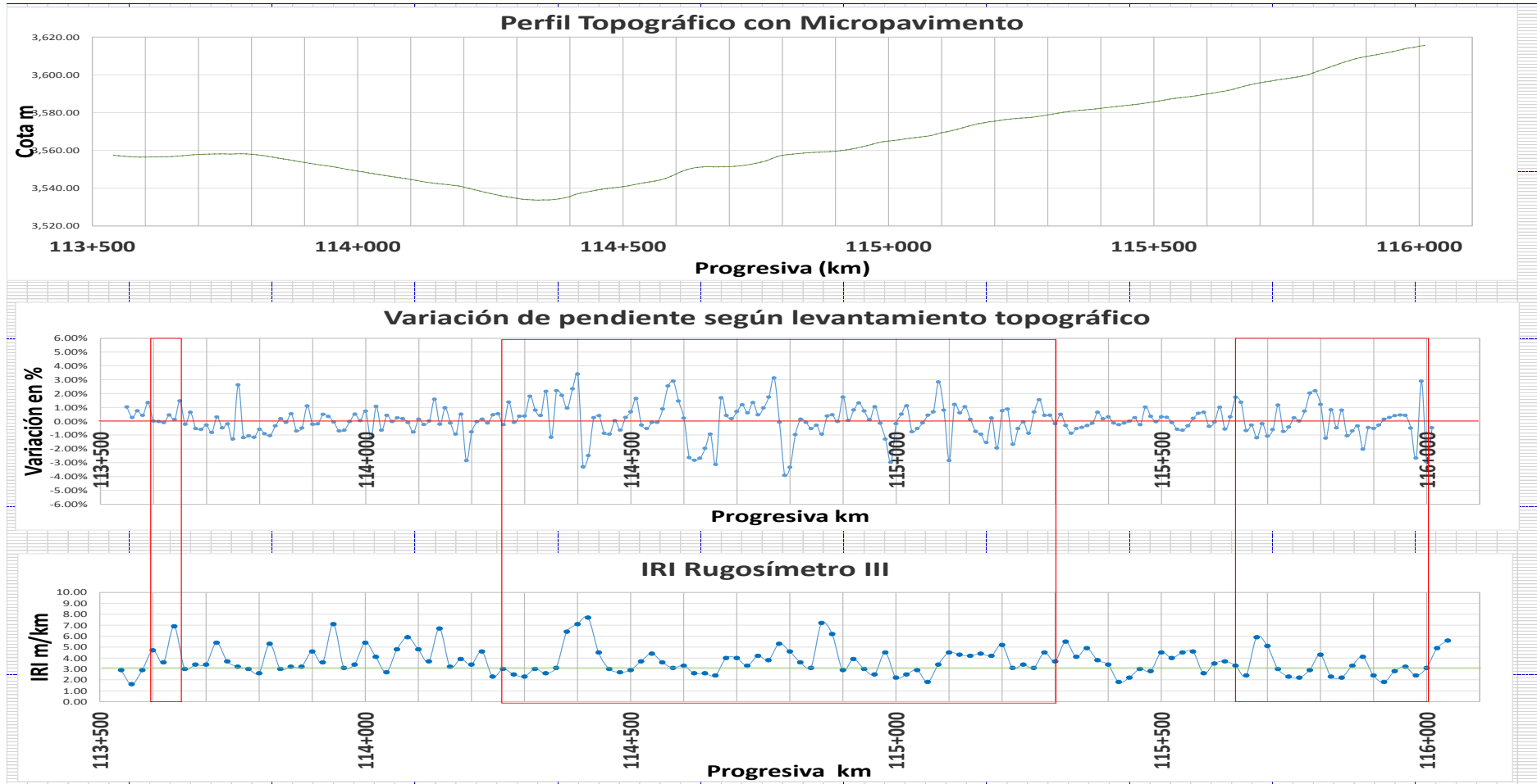
Comparación de perfil topográfico, variación de la pendiente e IRI en el sector Km 113+540 Km116+060
