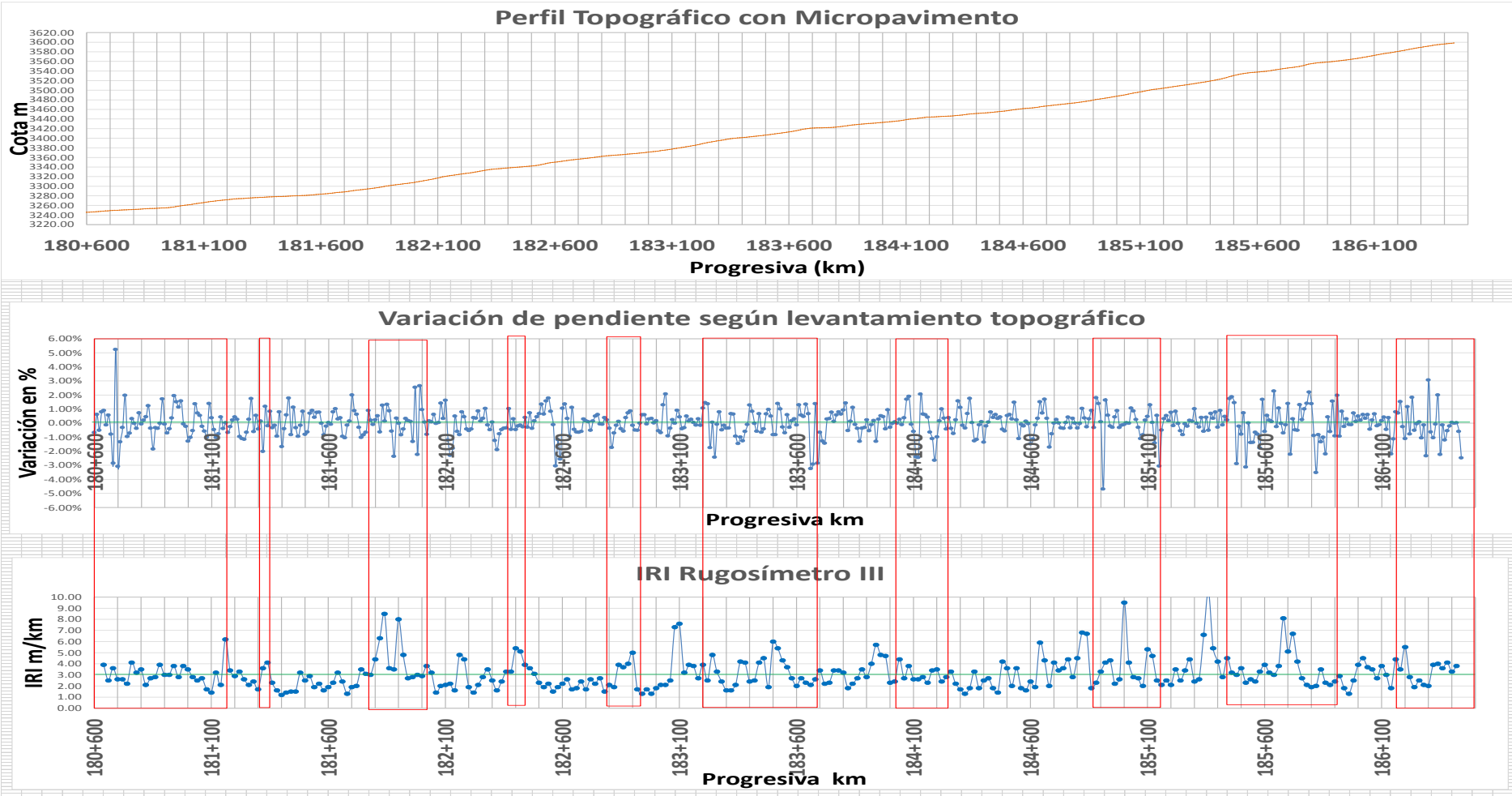
Comparación de perfil topográfico, variación de la pendiente e IRI en el sector Km 180+640-Km186+440
