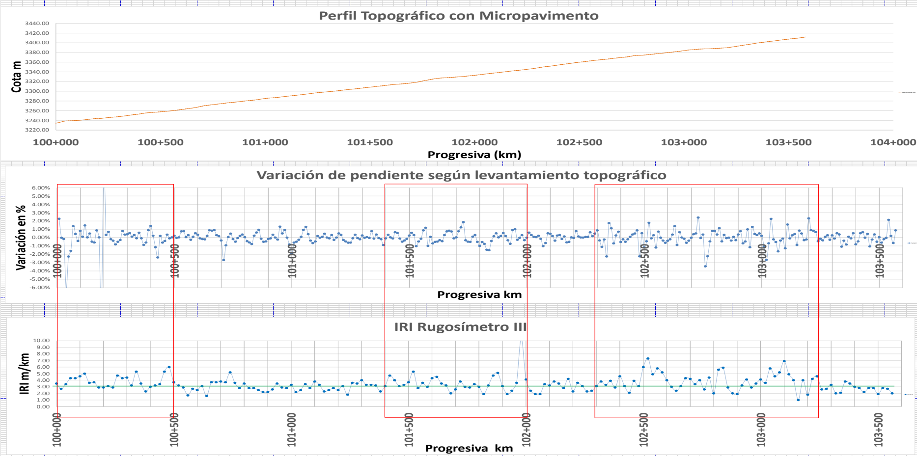
Comparación de perfil topográfico, variación de la pendiente e IRI en el sector Km 100+000-Km103+580
