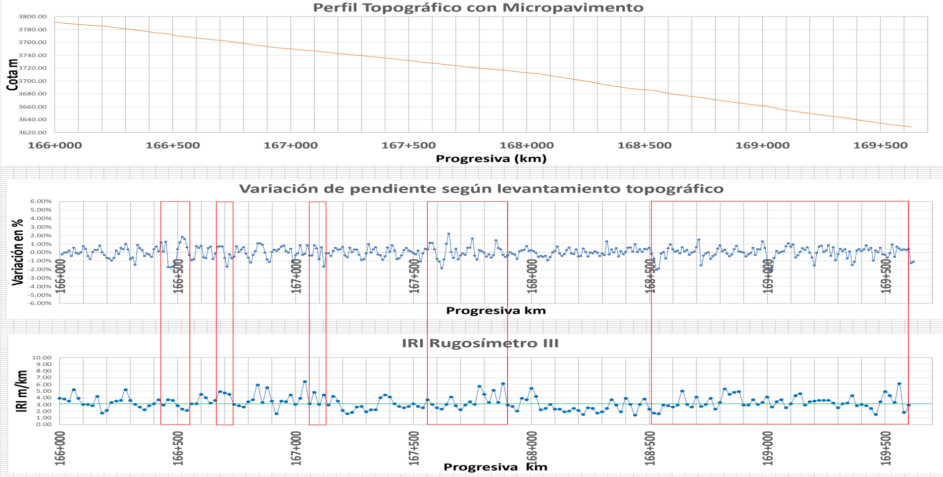
Comparación de perfil topográfico, variación de la pendiente e IRI en el sector Km 166+000-Km169+630
