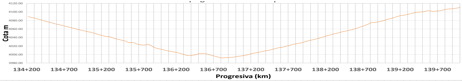
Comparación de perfil topográfico, variación de la pendiente e IRI en el sector Km 134+220-Km140+000
