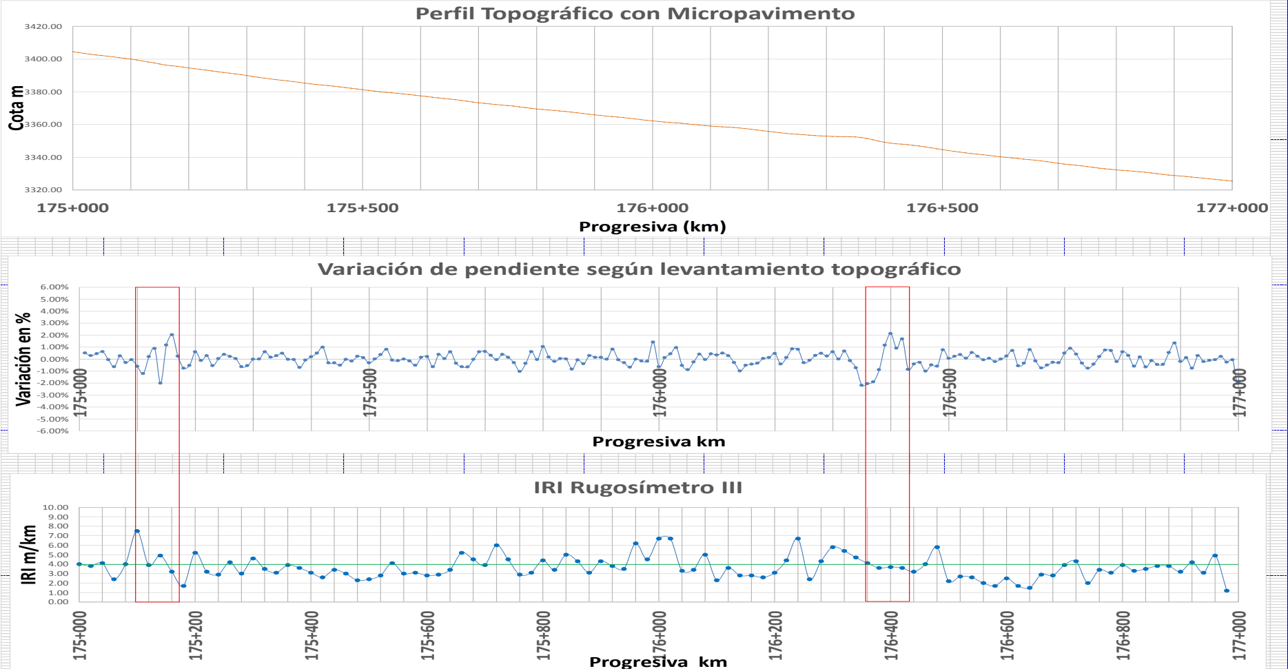
Comparación de perfil topográfico, variación de la pendiente e IRI en el sector Km 175+000-Km177+010
