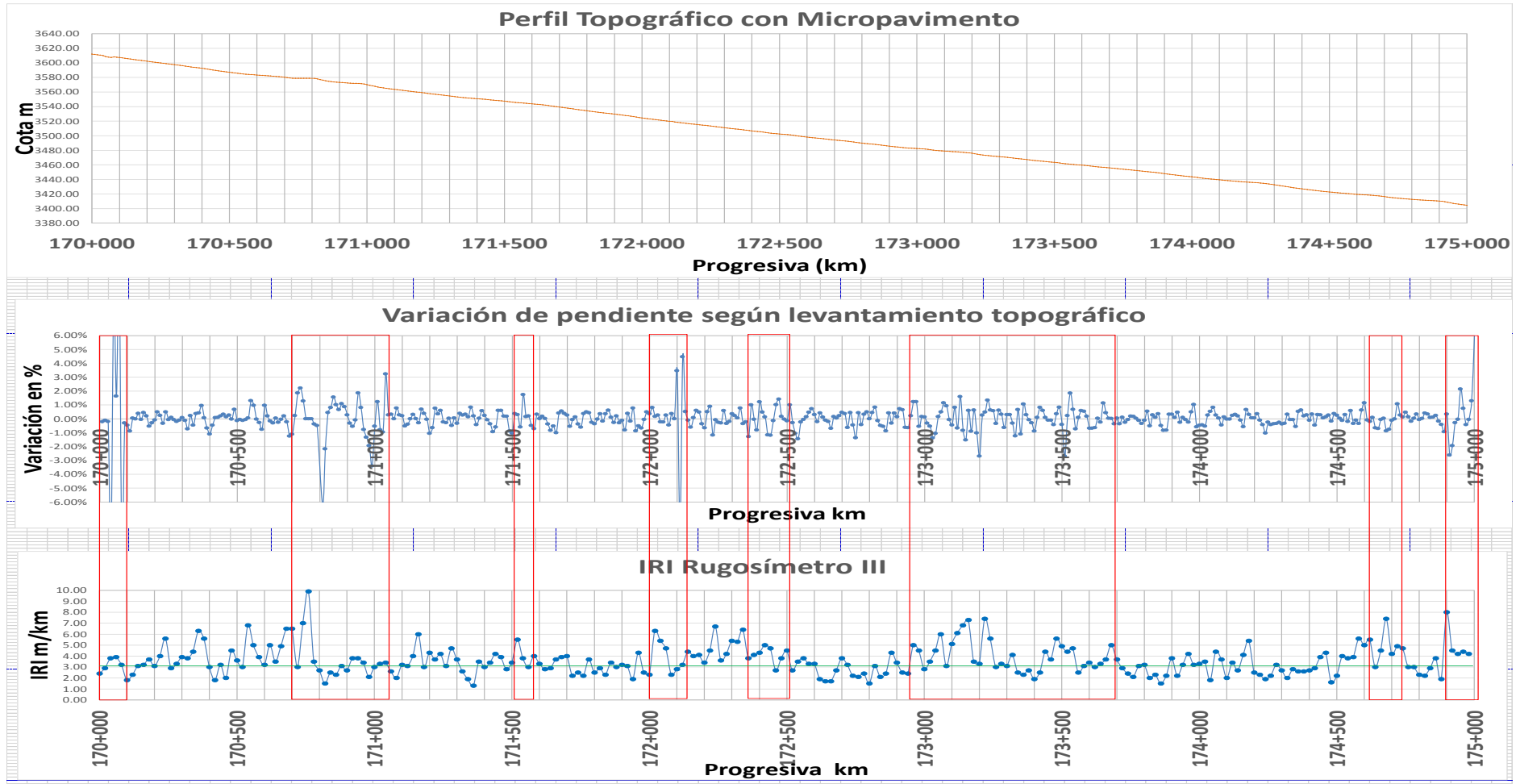
Comparación de perfil topográfico, variación de la pendiente e IRI en el sector Km 170+000- Km 175+000
