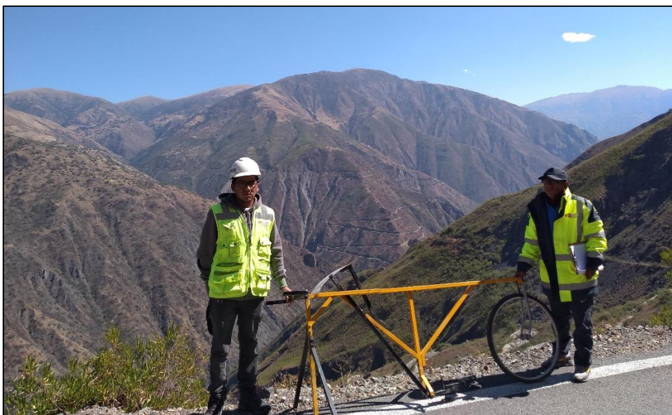
Fotografía 04. Personal Necesario para la Medición, Operario del Equipo y Asistente para anotar Lecturas del Tablero.
