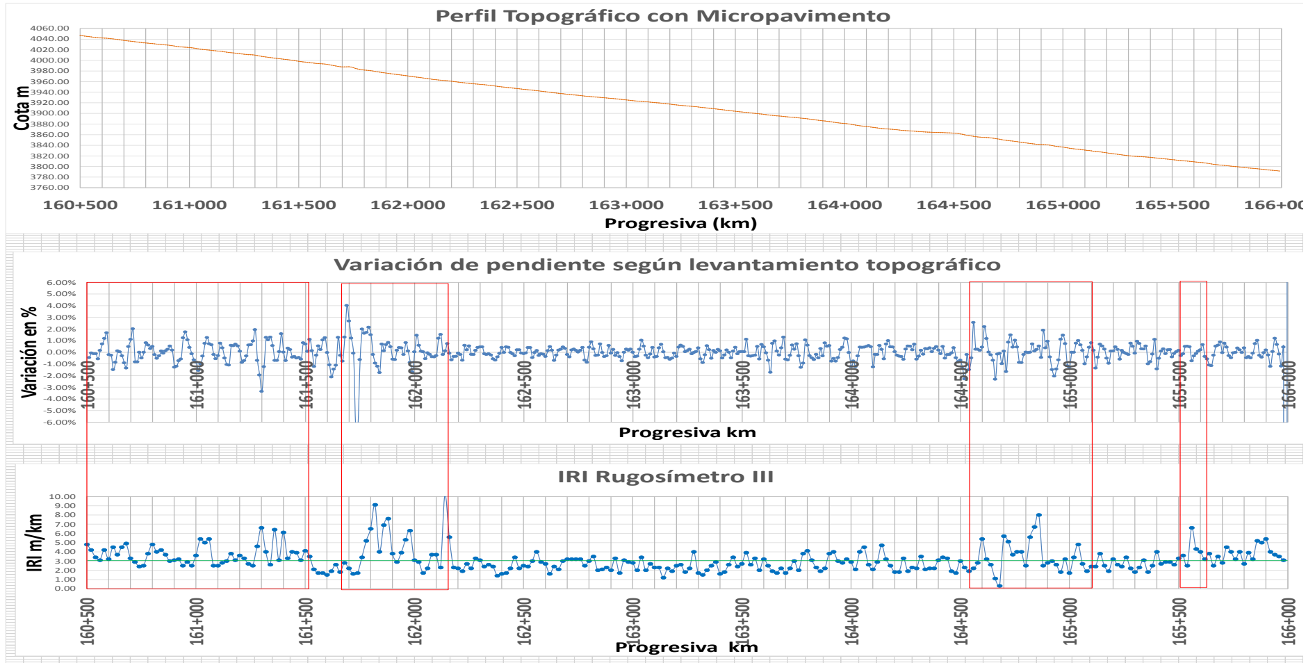
Comparación de perfil topográfico, variación de la pendiente e IRI en el sector Km 160+500-Km166+000
