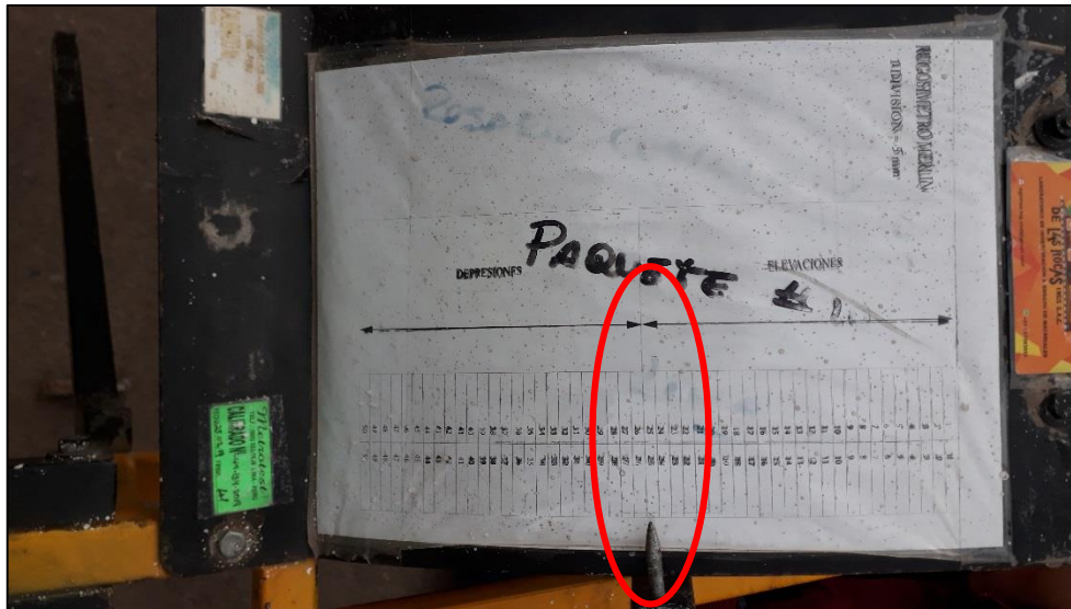
Fotografía 03. Verificación de Calibración del Equipo Merlín, El Tablero marca en la división 25 en una superficie horizontal.
