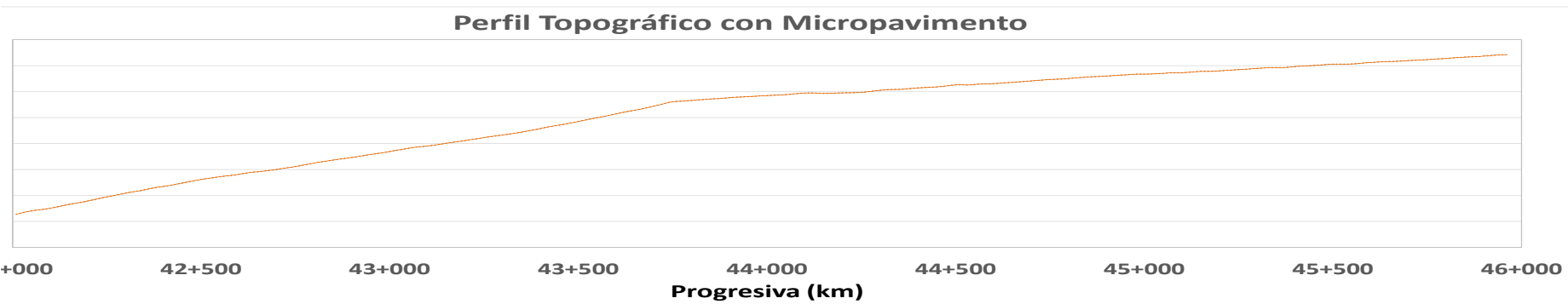
Comparación de perfil topográfico, variación de la pendiente e IRI en el sector Km 42+0000- Km 45+960
